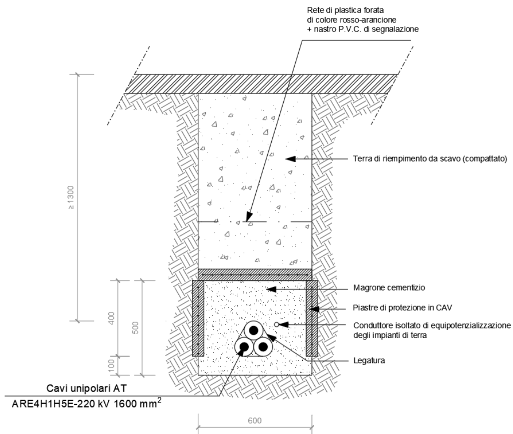
Figura 3.2 - Modalità di posa Cavo AT 220 kV
