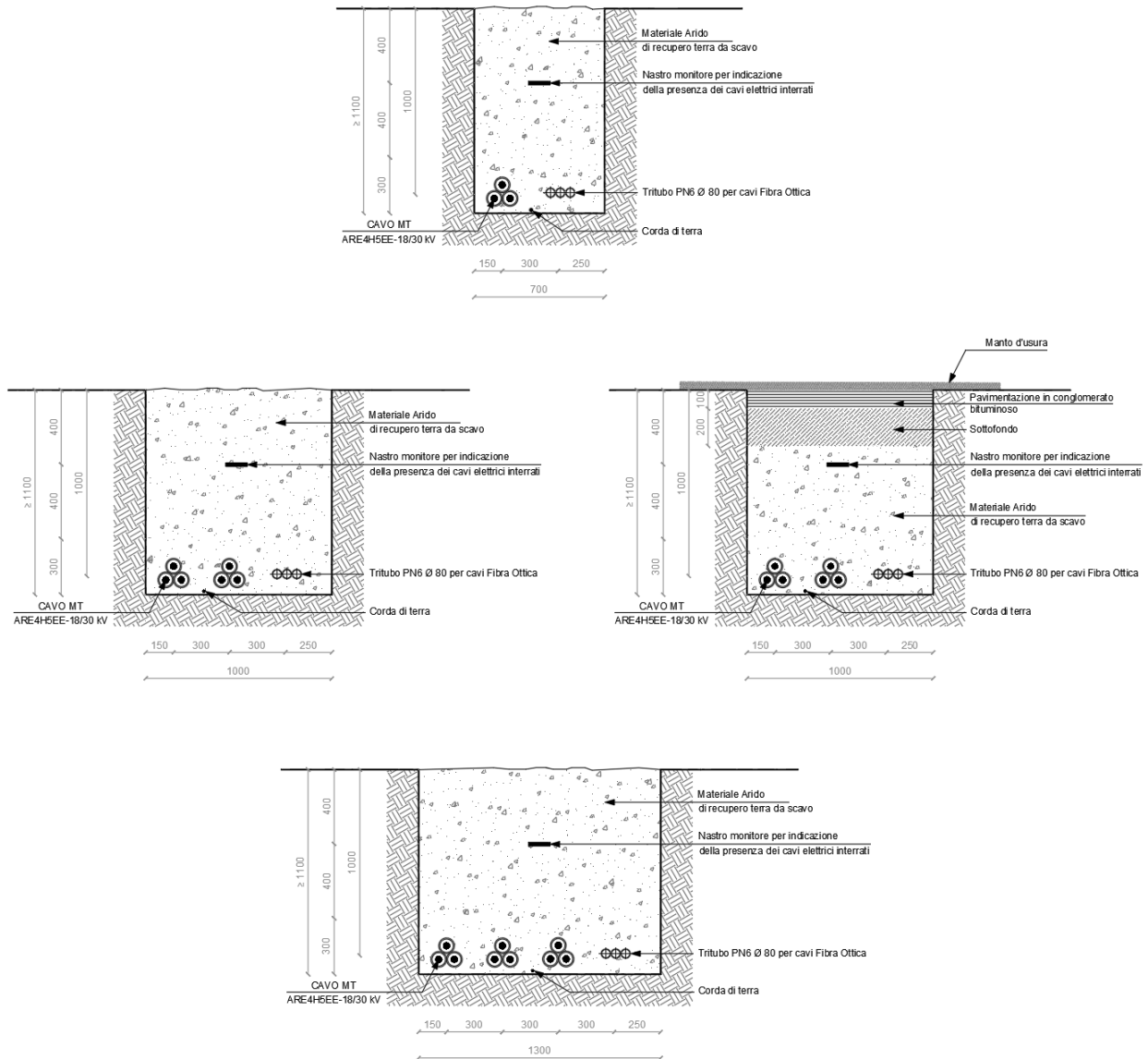
Figura 3.1 – Tipico modalità di posa cavidotto MT
