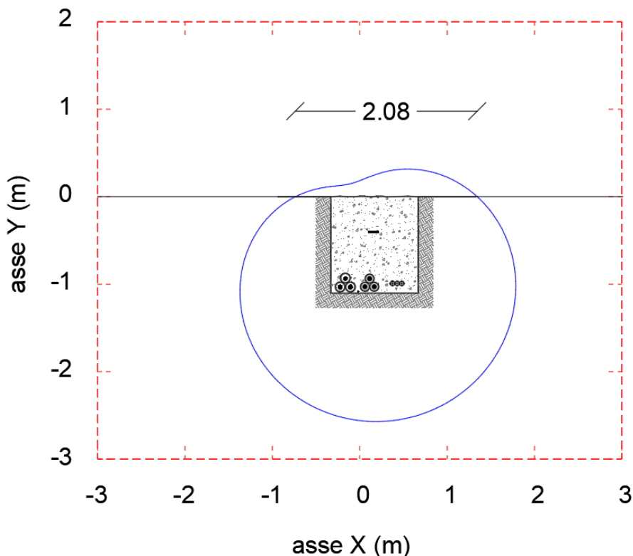
Figura 5.2 - Curva Equilivello 3 \mu T – 2 terne di cavi MT
