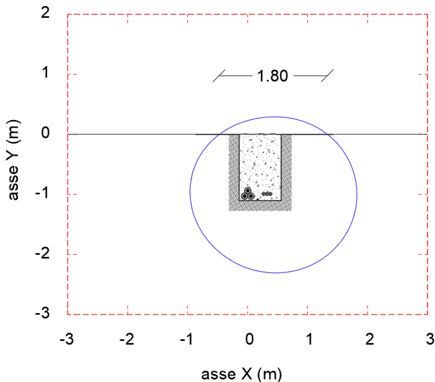
Figura 5.1 - Curva Equilivello 3\mu\text{T} – 1 terna di cavi MT
