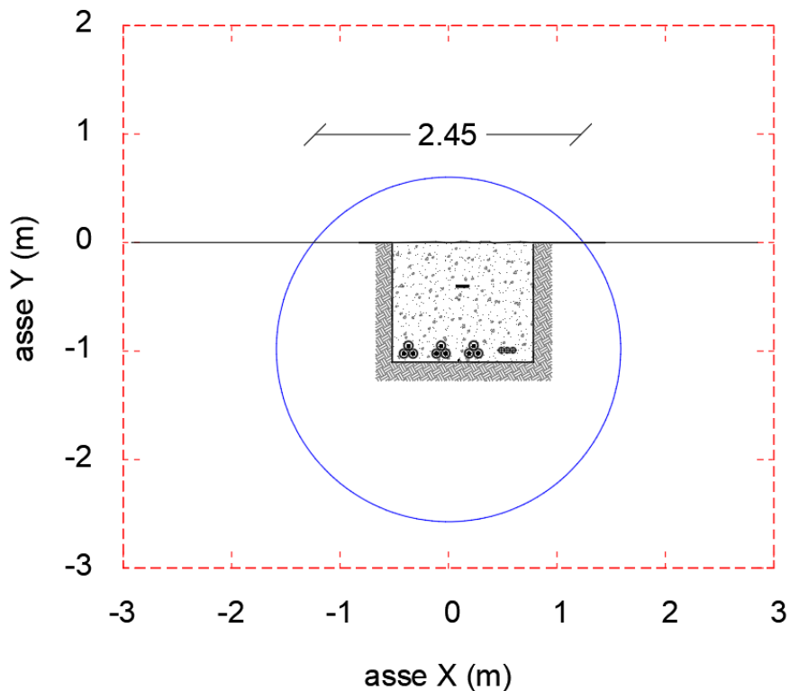
Figura 5.3 - Curva Equilivello 3 \mu\text{T} – 3 terne di cavi MT
