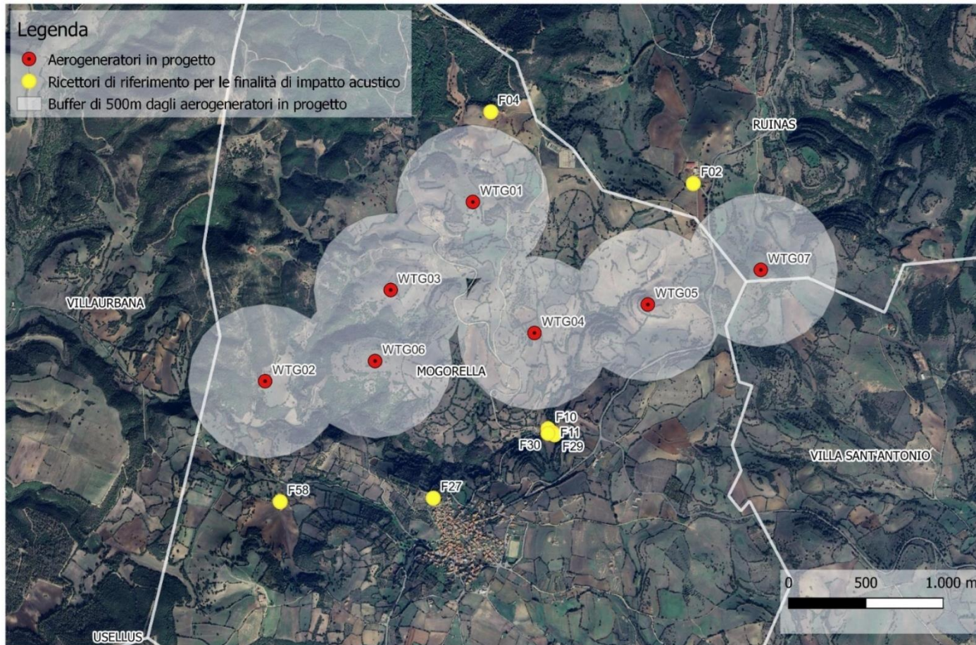
Figura 4.3: Individuazione planimetrica dei ricettori di impatto acustico
