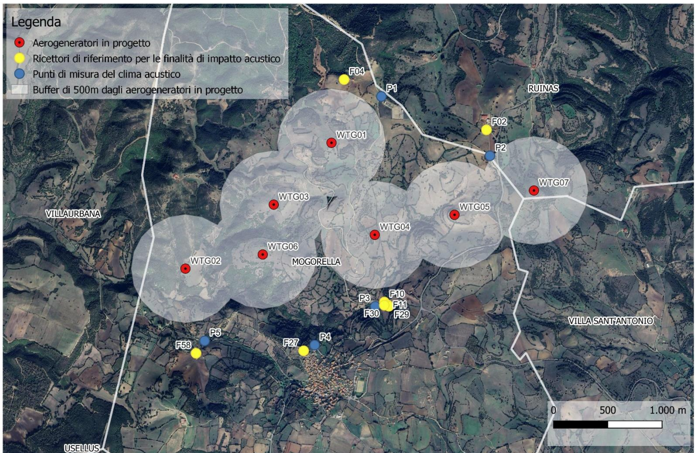
Figura 4.2: Ubicazione dei punti di misura del clima acustico rispetto ai fabbricati di interesse per l'impatto acustico e gli aerogeneratori in progetto
