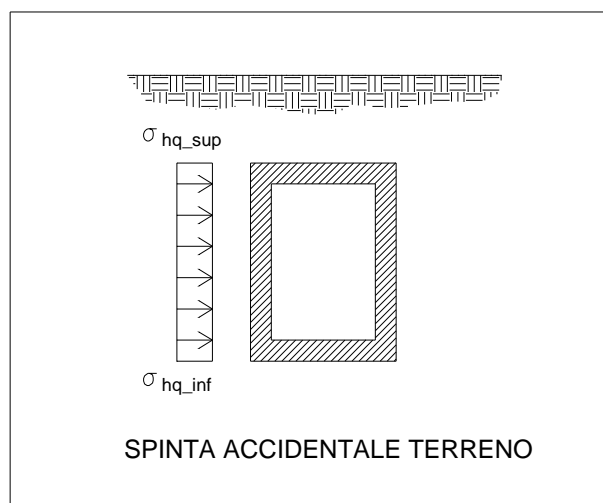
Figura 5 – Schema di carico spinta del terreno per sovraccarico stradale
