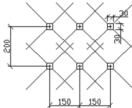
Figura 4 – Impronta di carico
