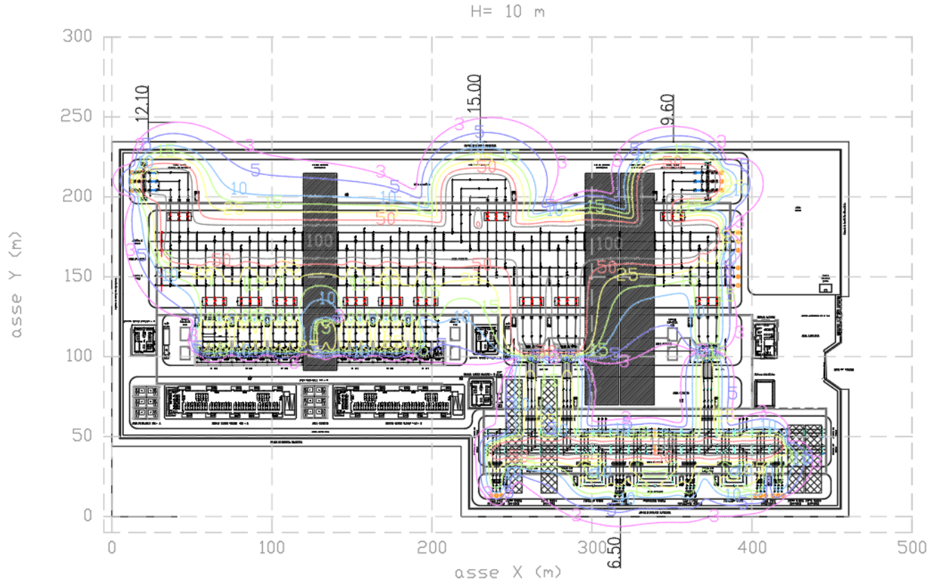
Figura 8 – Livelli di campo magnetico a 10 m dal piano della stazione
