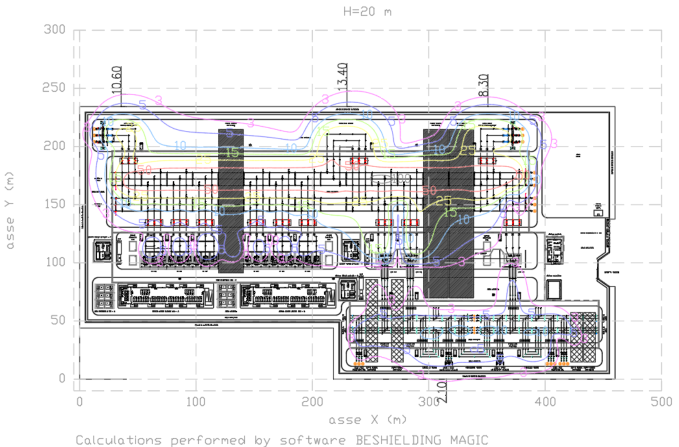
Figura 10 – Livelli di campo magnetico a 20 m dal piano della stazione
