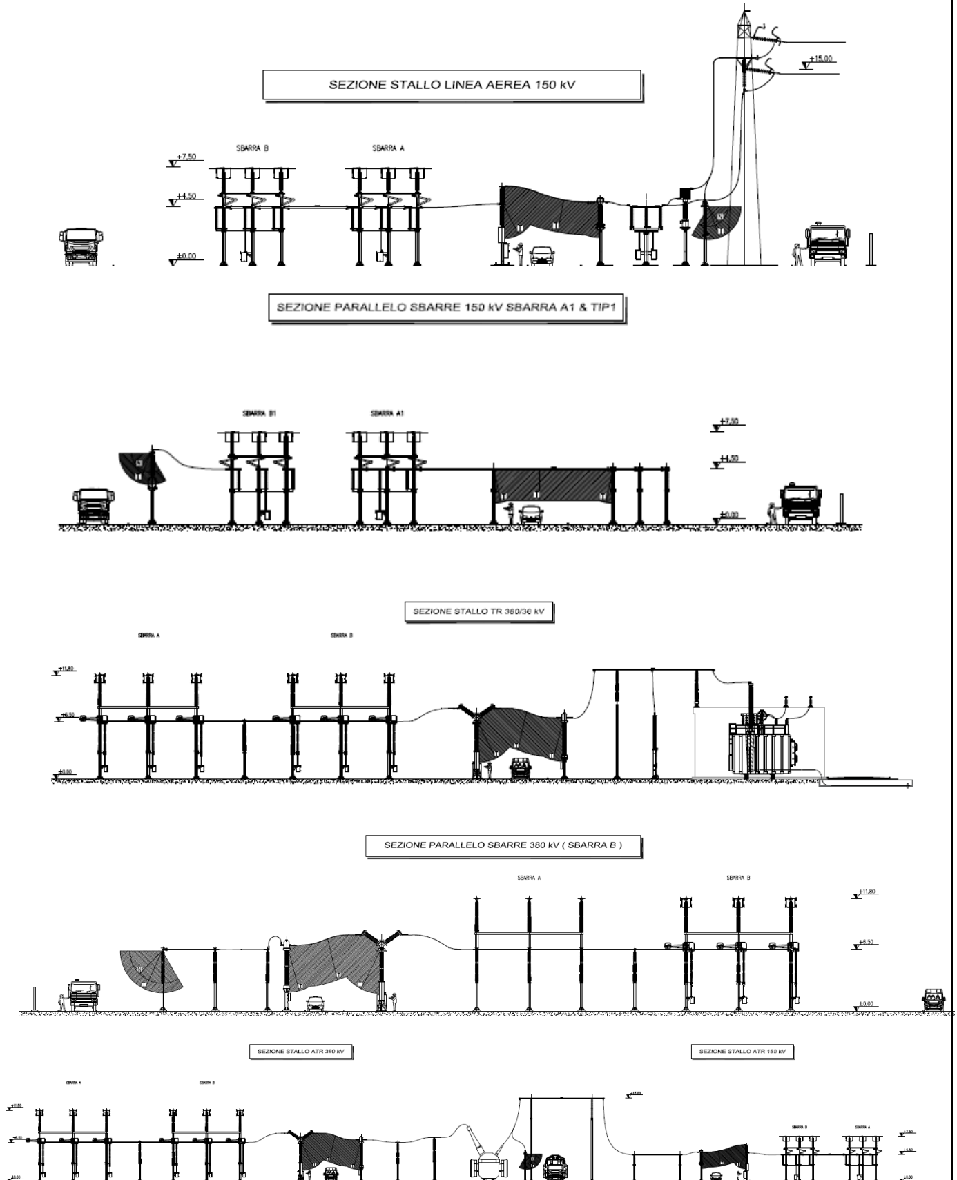
Figura 3 – Sezioni degli stalli linea e delle sbarre delle sezioni 380, 150 e 36 kV della stazione, rif. Doc. 70453
