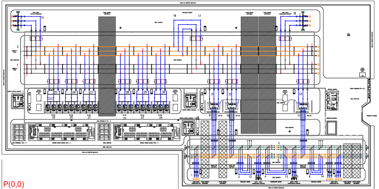
Figura 4 – Schematizzazione degli elementi attivi all'interno della planimetria
