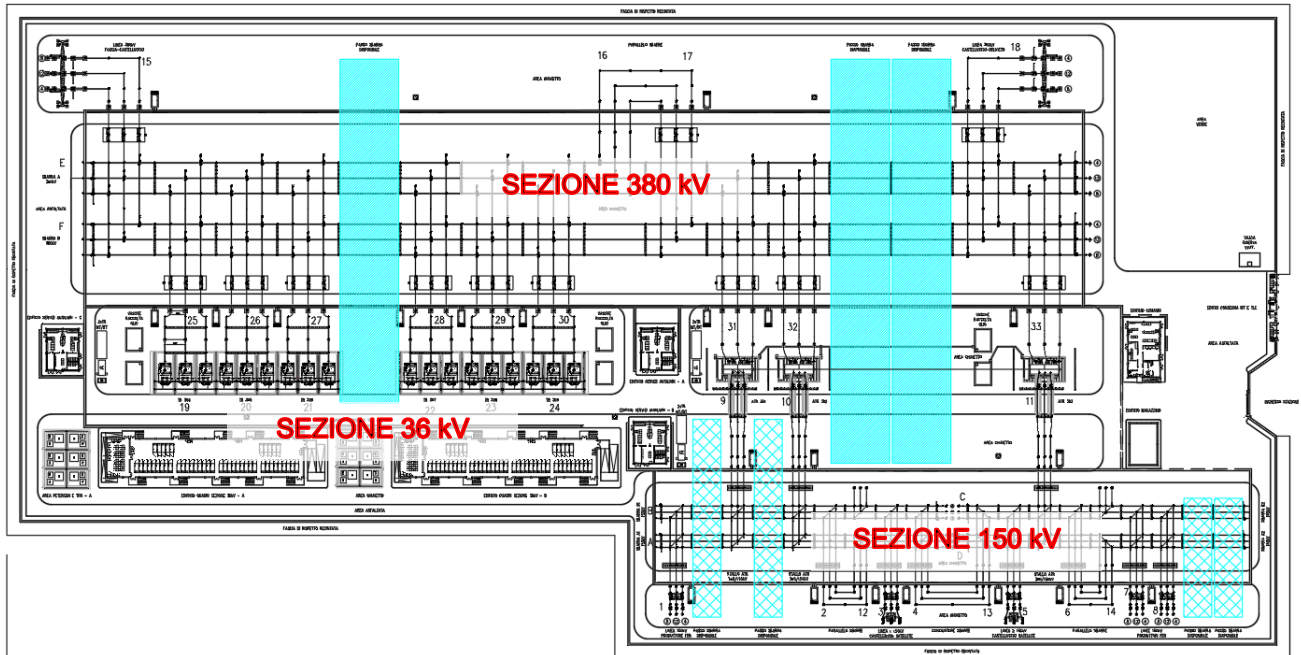
Figura 1: planimetria della stazione
