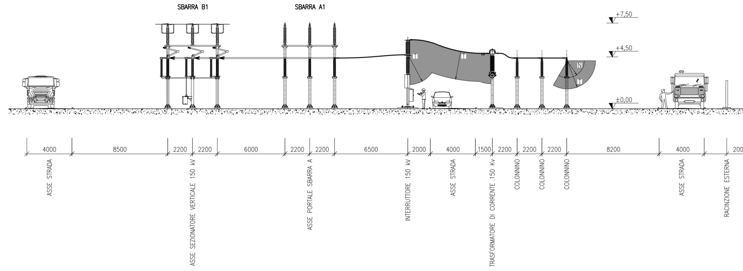
SEZIONE PARALLELO SBARRE 150 kV
