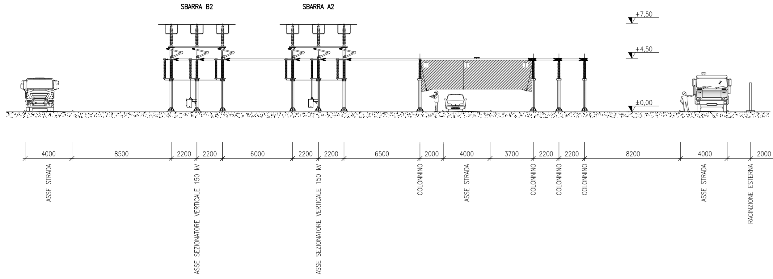
SEZIONE CONGIUNTURE SBARRE 150 kV
