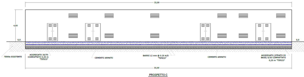
Fig. 8 - Cabina di ricezione, sezionamento e controllo
