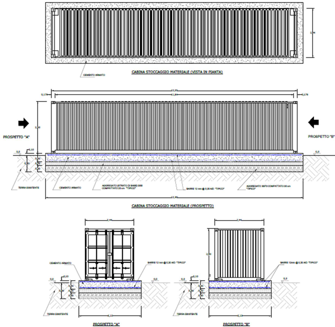
Fig. 9 - Cabina stoccaggio materiale
