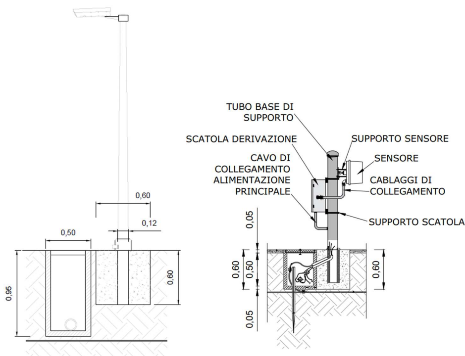
Fig. 14 – Sistema antintrusione
