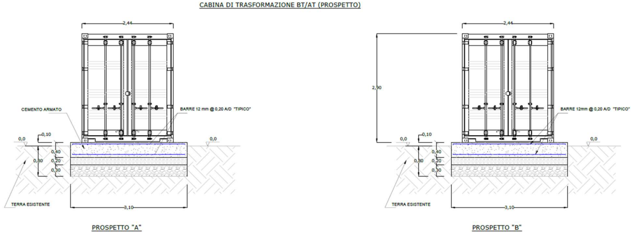
Fig. 7 - Cabina di trasformazione BT/AT
