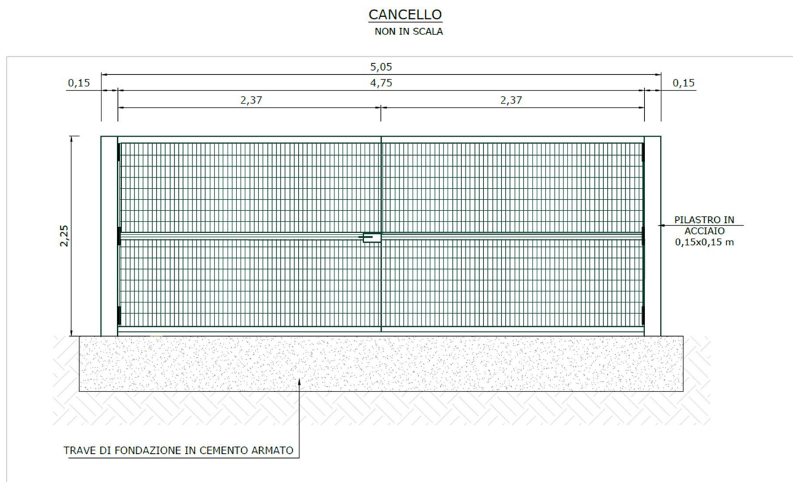
Fig. 12 – Cancello a doppia anta.
