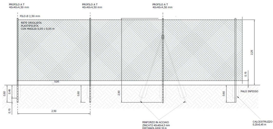
Fig. 11 – Recinzione perimetrale
