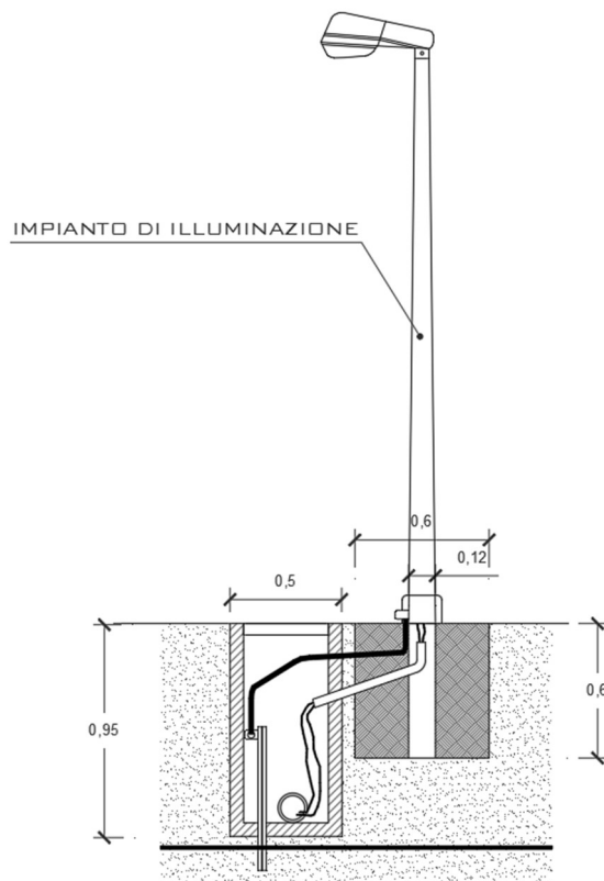
Fig. 15 – Sistema di illuminazione
