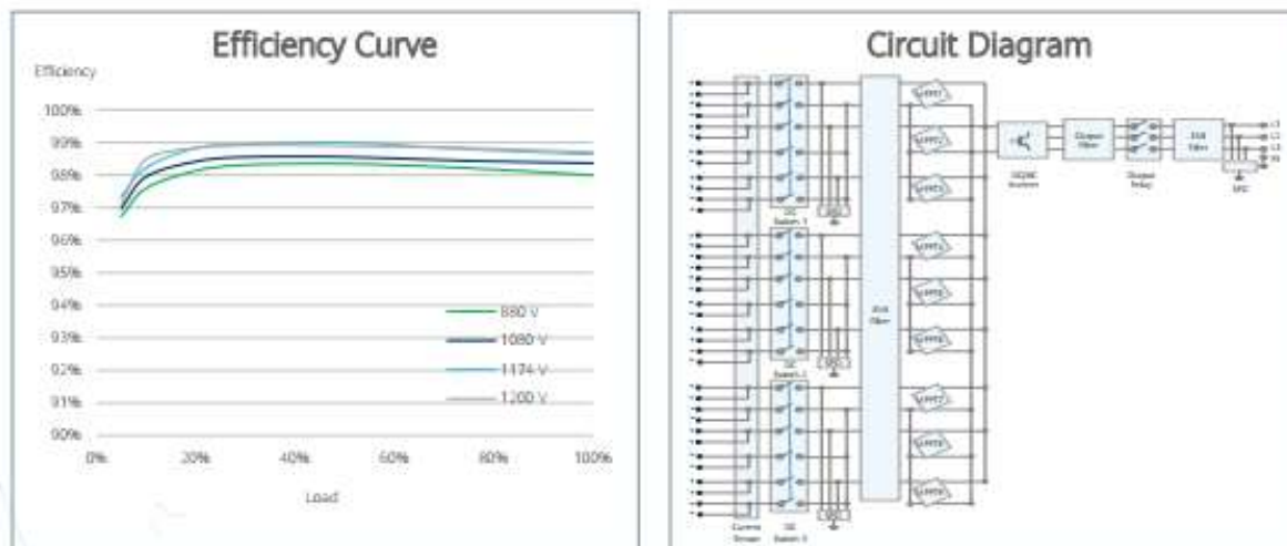
Fig. 6 - Dimensioni, specifiche tecniche e prestazionali dell'inverter
