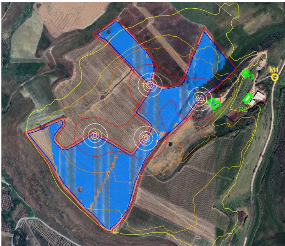
Figura 12 - Risultato della simulazione con linee di iso-rumorosità colorate da 20 dB (Rossa) a 10 (Gialla)
