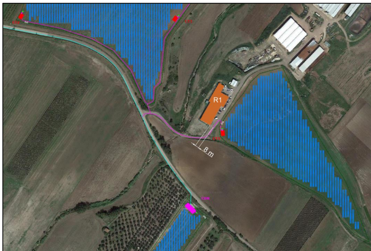
Figura 7 – Layout dell’impianto con indicazione dei ricettori potenzialmente sensibili
