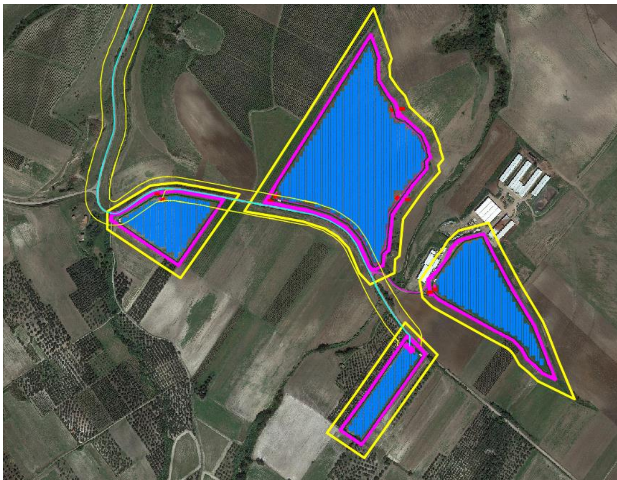
Figura 4 – Identificazione area vasta in giallo come buffer di 30 m intorno all'impianto ed al tracciato del cavidotto
