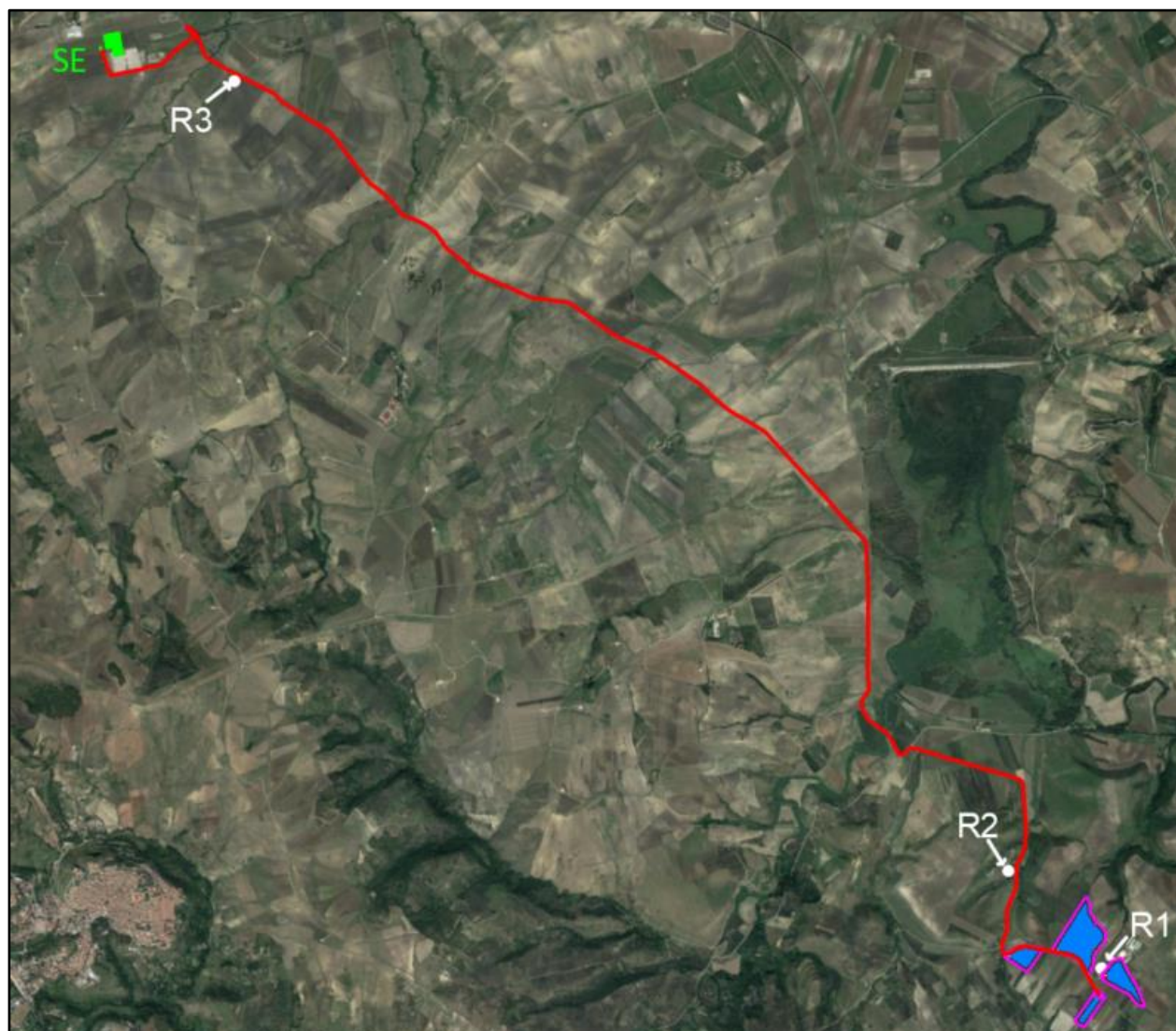
Figura 14 – Inquadramento su ortofoto percorso cavidotto e dei relativi recettori
