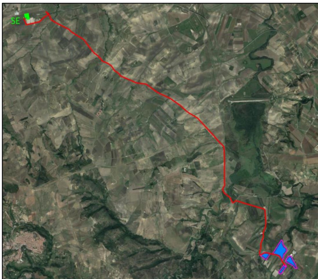
Figura 9 - Connessione alla RTN: confine catastale (in magenta), percorso del cavidotto (in rosso), futuro ampliamento della SE (in verde)
