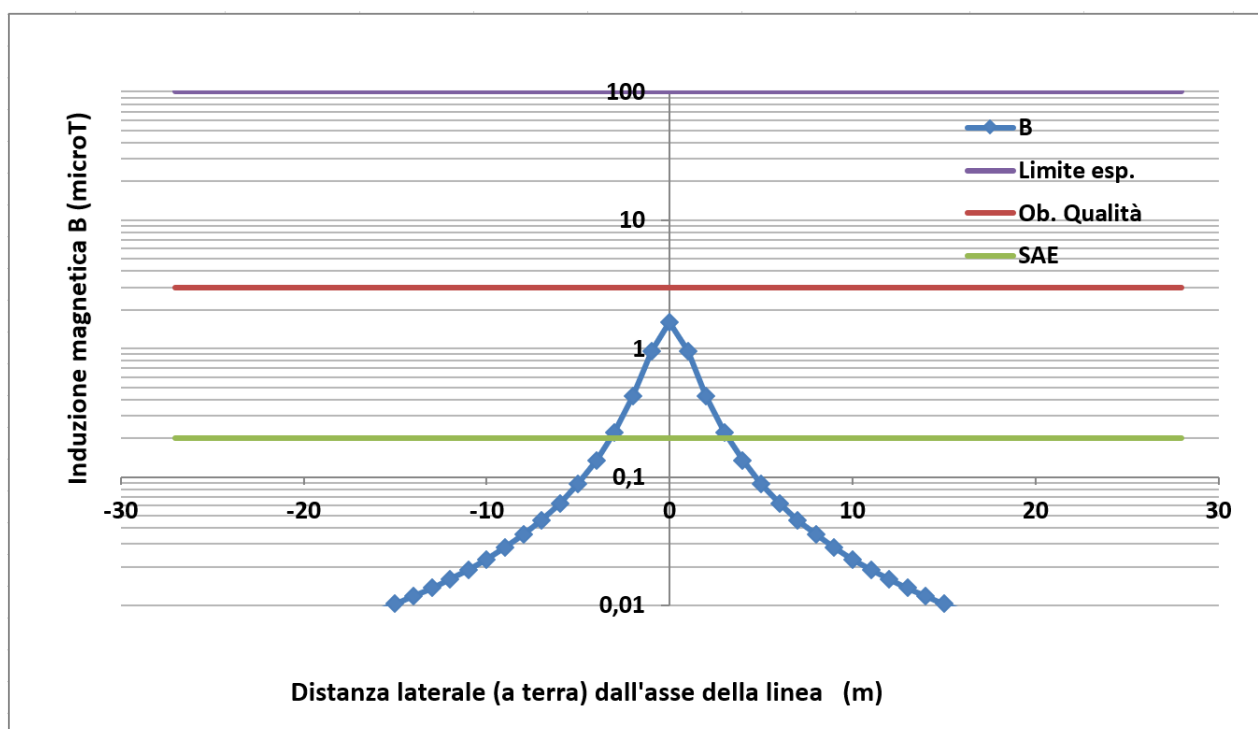
Figura 8 – Campo di induzione magnetica B ( \mu T ) generato dal cavidotto interno MT del progetto agrivoltaico in relazione ai limiti di esposizione e obiettivo di qualità-R1
