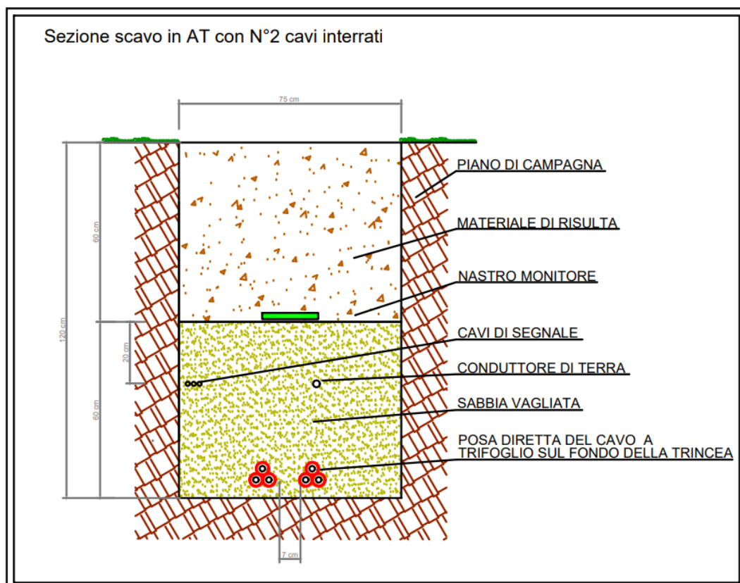
Figura 6 – Sezione di scavo per i cavidotti interrati in AT interni all'area d'impianto
