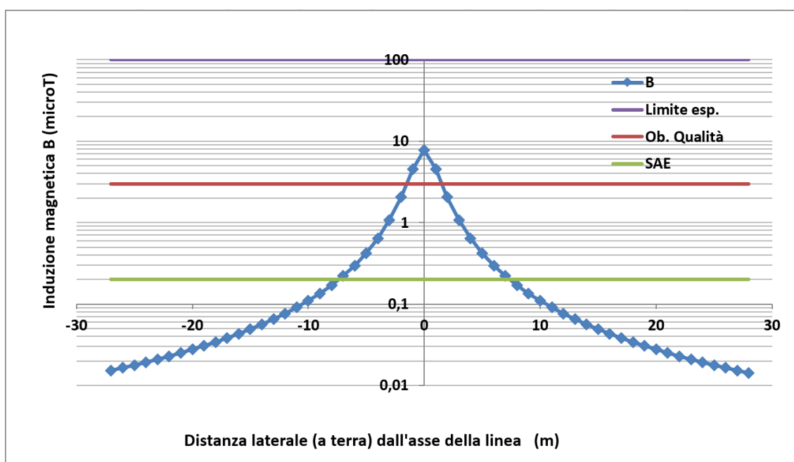
Figura 17 – Campo di induzione magnetica B ( \mu\text{T} ) generato dal cavidotto di evacuazione AT del progetto agrivoltaico in relazione ai limiti di esposizione e obiettivo di qualità.
