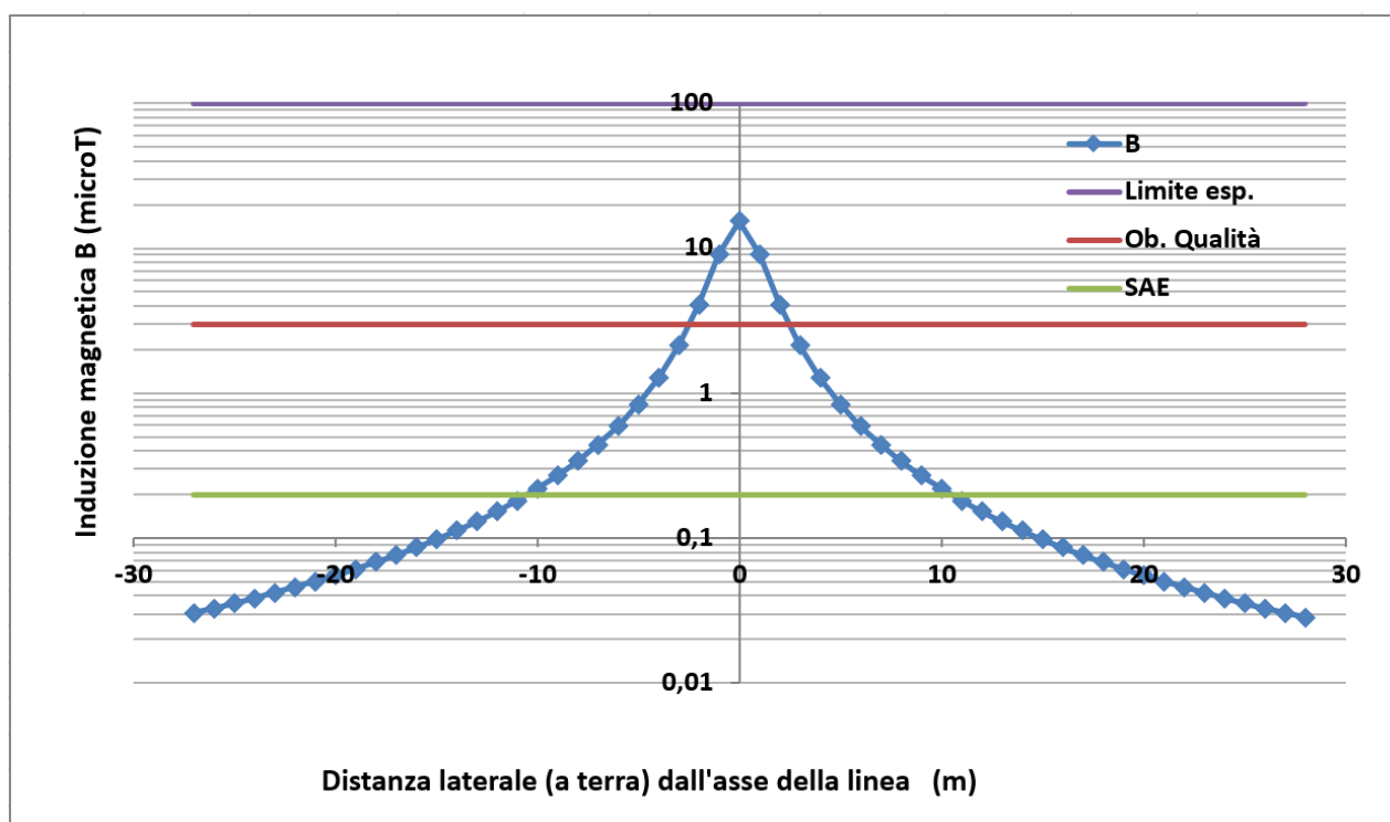
Figura 18 – Campo di induzione magnetica B ( \mu T) generato dal cavidotto di evacuazione AT del progetto agrivoltaico in relazione ai limiti di esposizione e obiettivo di qualità
