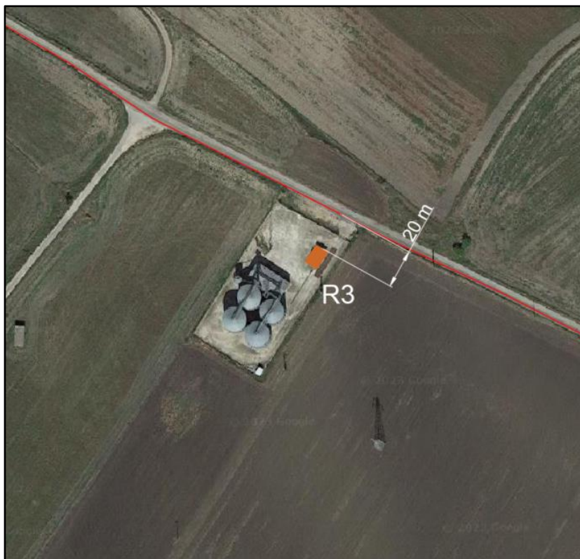
Figura 16 – Inquadramento su ortofoto-posizione dei recettori R3
