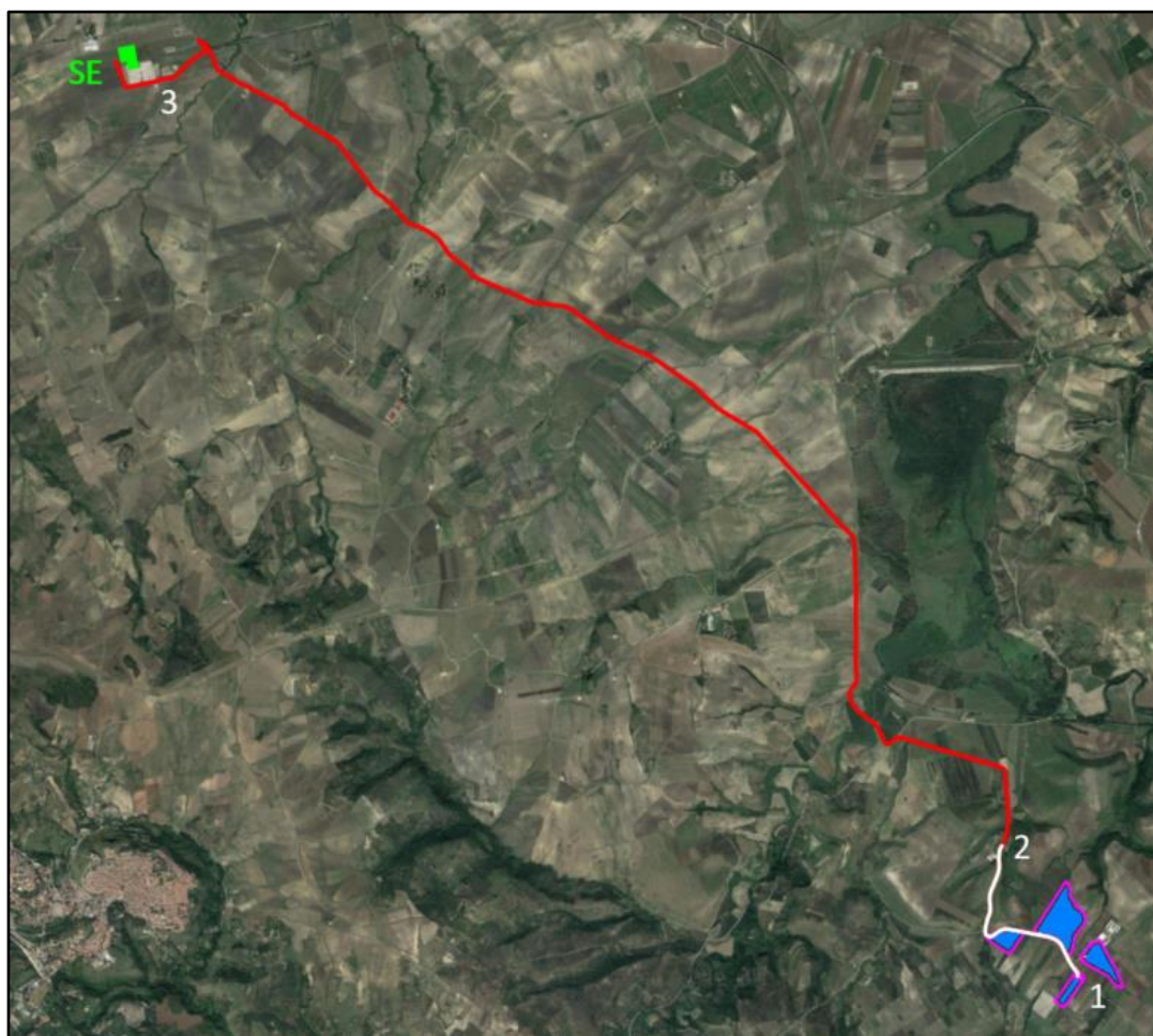
Figura 10 - Inquadramento su ortofoto della suddivisione del tracciato del cavidotto
