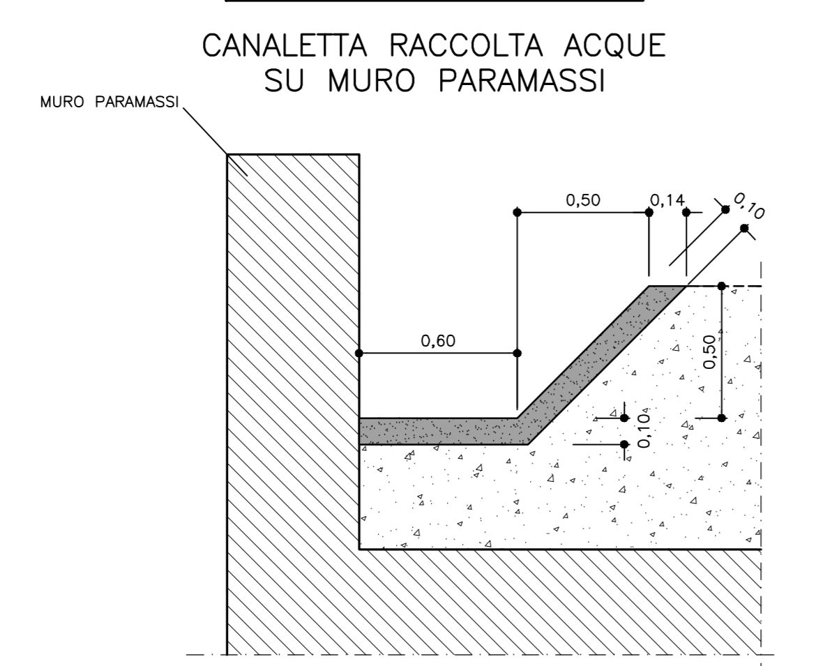
PARTICOLARE "2" SCALA 1:20
