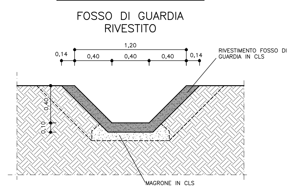
PARTICOLARE "1" SCALA 1:20
