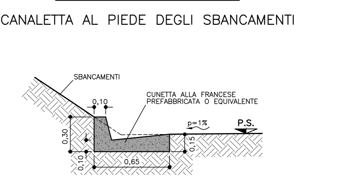
PARTICOLARE "3" SCALA 1:20
