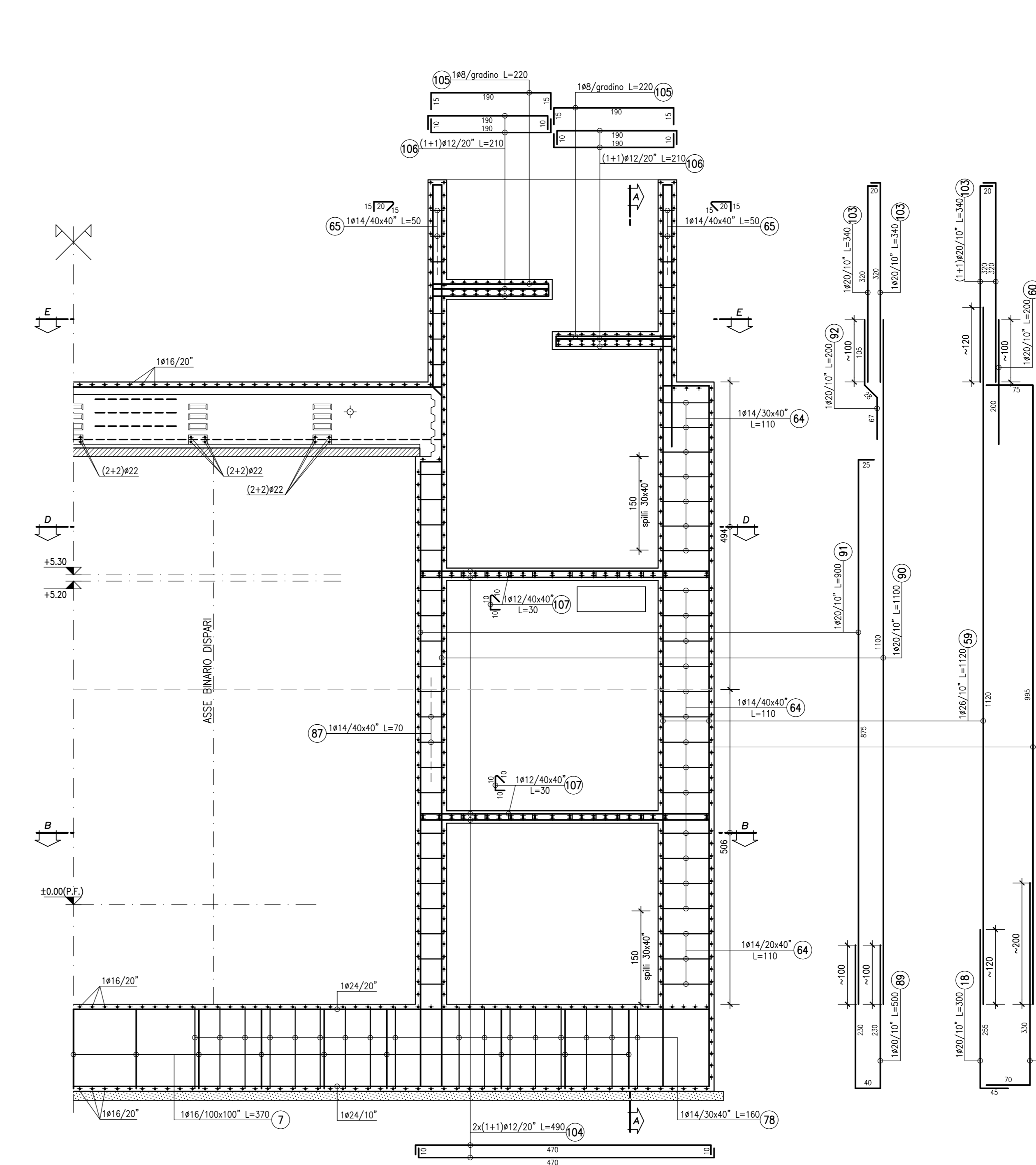
SEZIONE TRASVERSALE G-G scala 1:50
