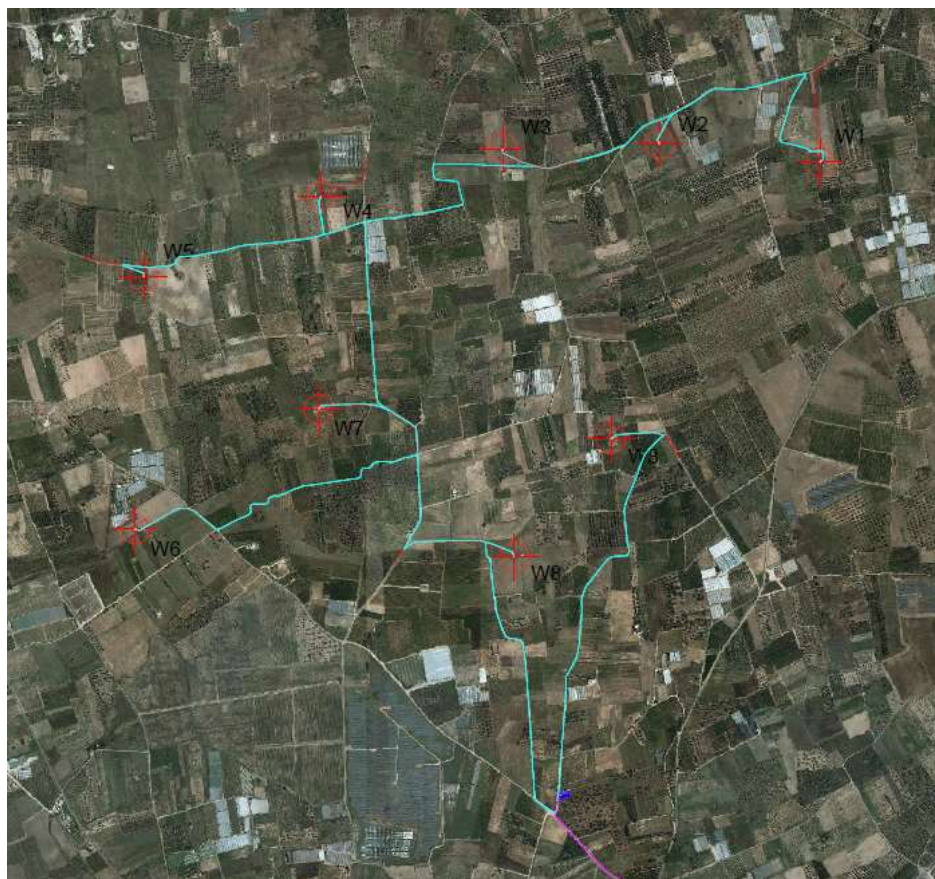
Figura 1.2.-1.:Layout di impianto (Fonte: Ortofoto SIT_Puglia).
