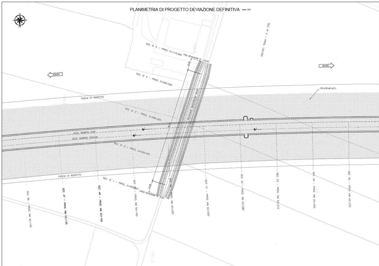
Planimetria di Progetto della Deviazione Definitiva alla pK 42+216.
