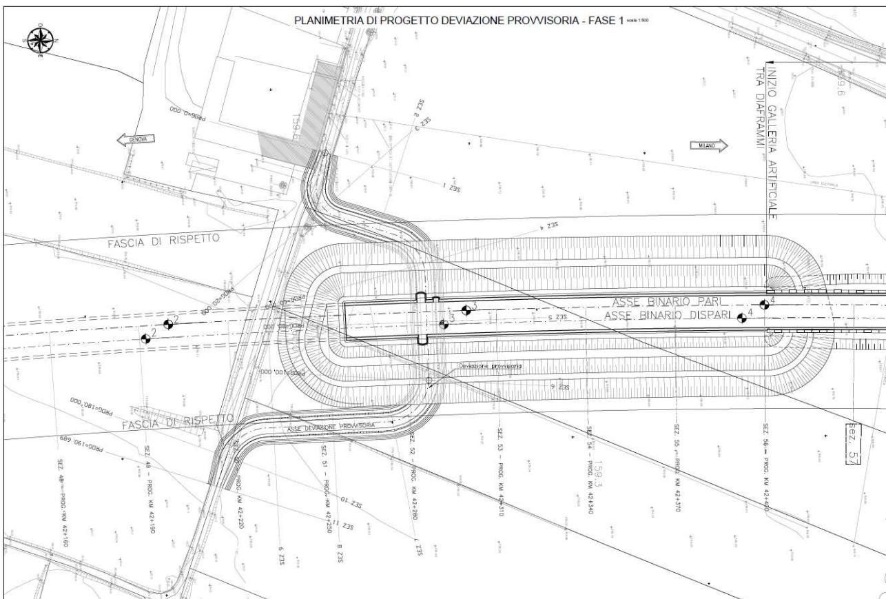
Planimetria di Progetto della Deviazione Provvisoria alla pK 42+216 – Fase 1.
