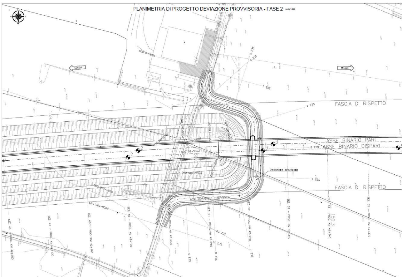
Planimetria di Progetto della Deviazione Provvisoria alla pK 42+216 – Fase 2.
