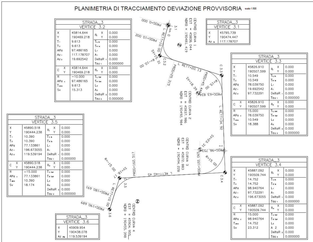
Planimetria di Tracciamento della Deviazione Provvisoria alla pK 42+216.
