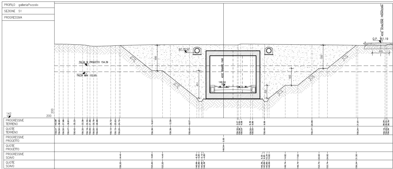
Sezione Trasversale della Deviazione Provvisoria alla pK 42+216.
