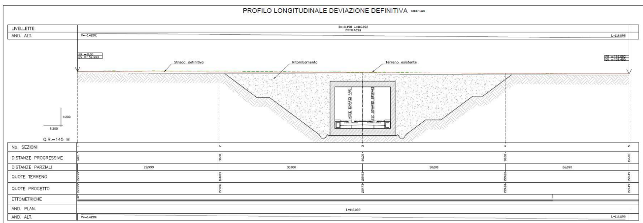
Profilo Longitudinale della Deviazione Definitiva alla pK 42+216.
