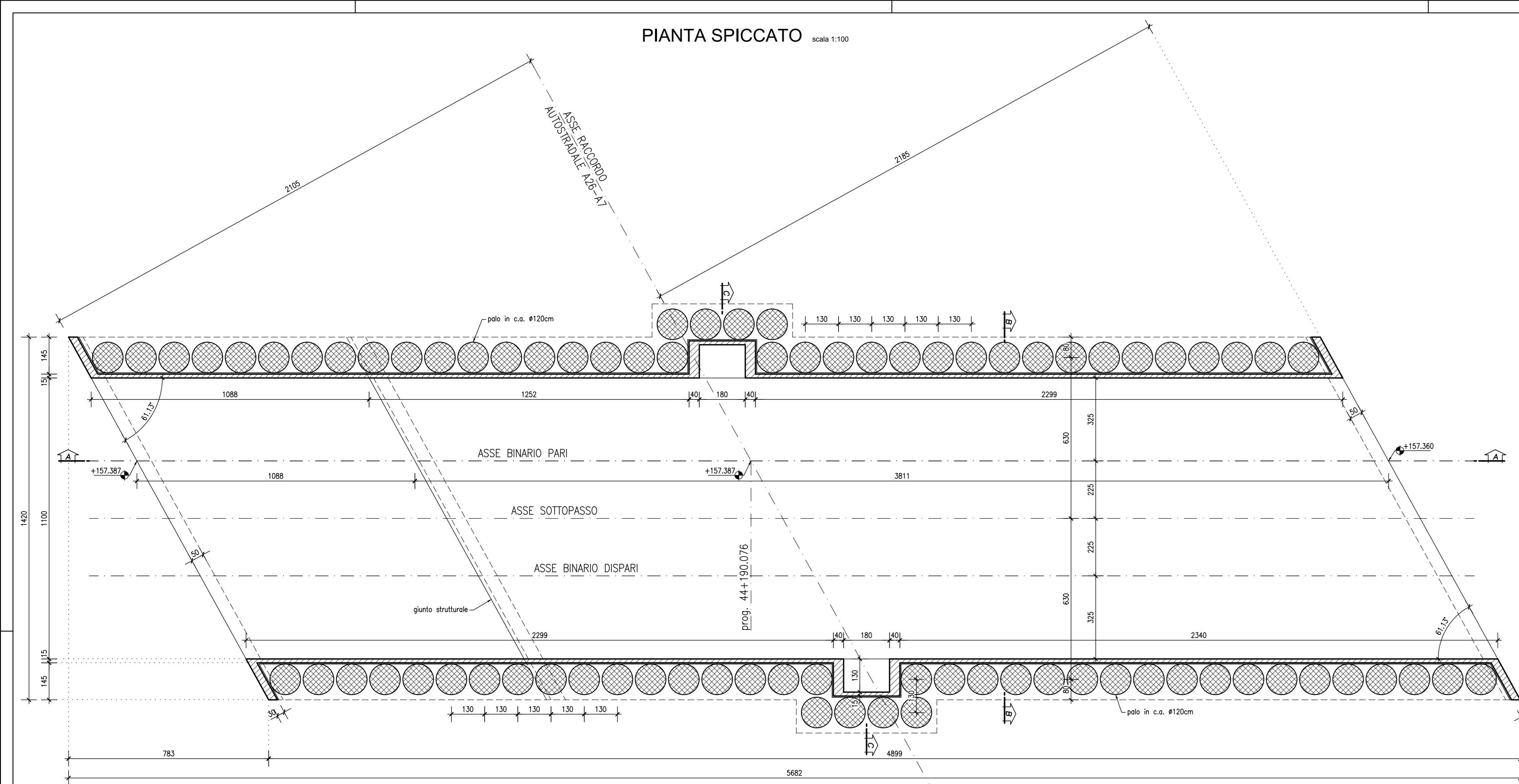
PIANTA COPERTURA scala 1:100
