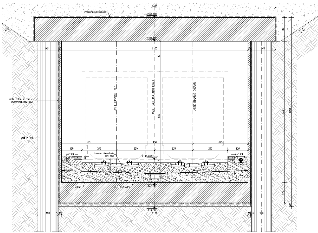
Figura 2. Sottopasso ferroviario. Sezione trasversale sezione corrente
