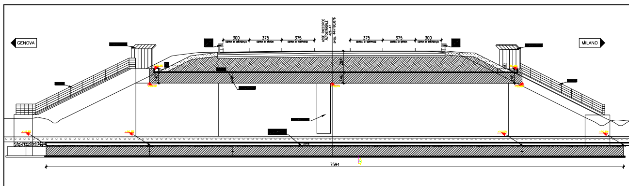
Figura 1. Sottopasso ferroviario. Sezione longitudinale in asse opera
