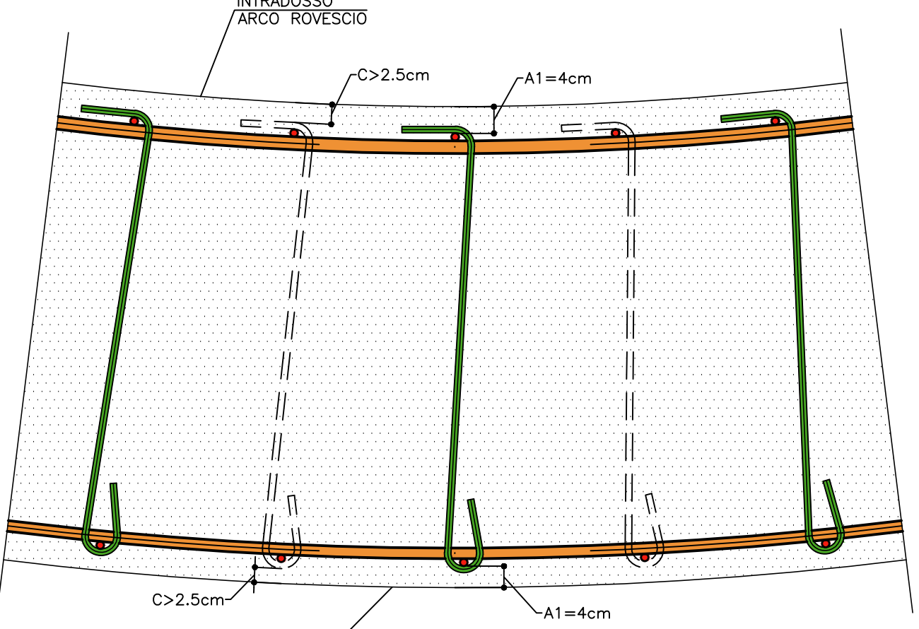
PARTICOLARE "2" SCALA 1:10 PARTICOLARE COPRIFERRO ARCO ROVESCIO
