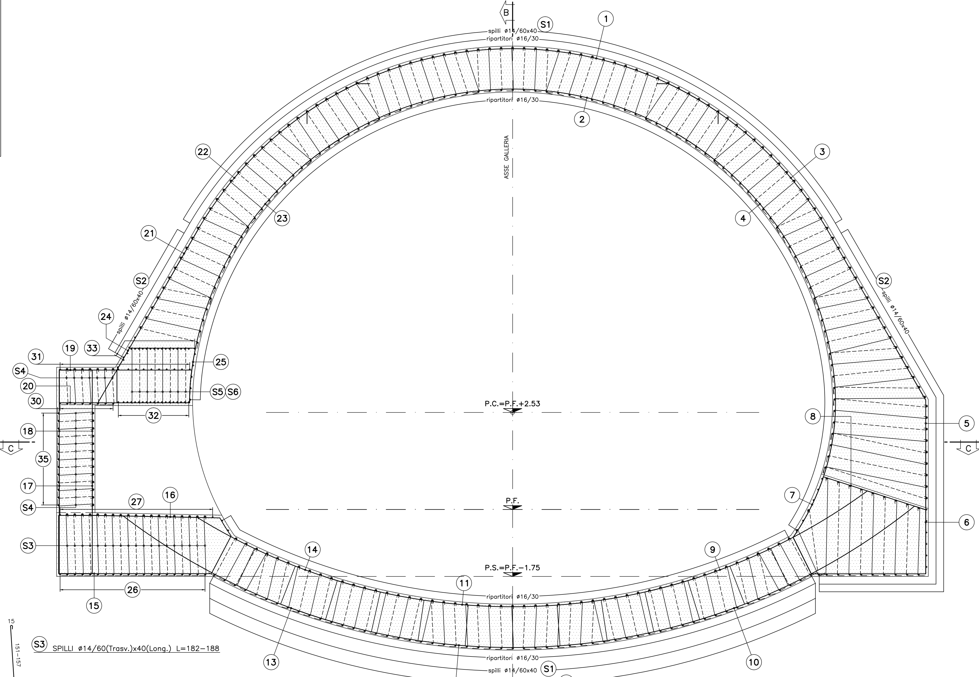
SEZIONE A-A SCALA 1:50 SEZIONE TRASVERSALE
