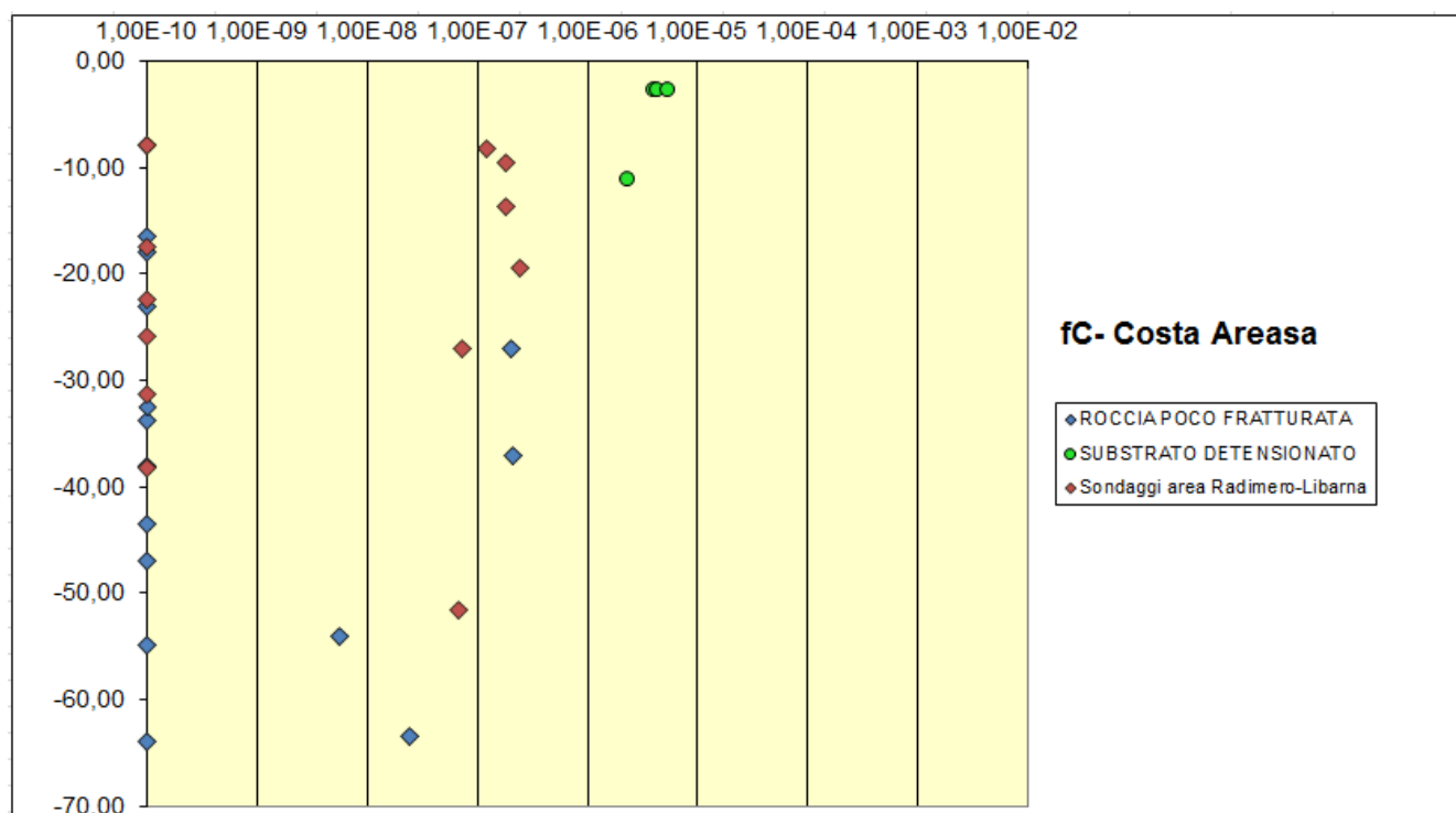
Figura 3 - Distribuzione dei valori di permeabilità ottenuti da prove in foro per la formazione di Costa Areaa (fCa), secondo la profondità (i valori pari a 1E-10 sono stati attribuiti indicativamente alle prove con assorbimento nullo, per significare che l'ammasso roccioso ha permeabilità bassissima, comunque inquadrabile nella classe AFTES minore, con K < 1E-8 ).
