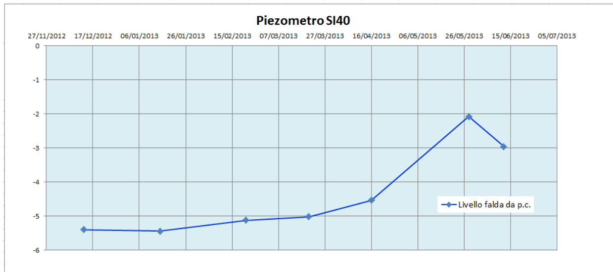
Figura 5 Piezometro del sondaggio SI40 (Progetto Esecutivo – Lotto 1) Monitoraggio della falda nel periodo 13/12/2012 – 12/06/2013
