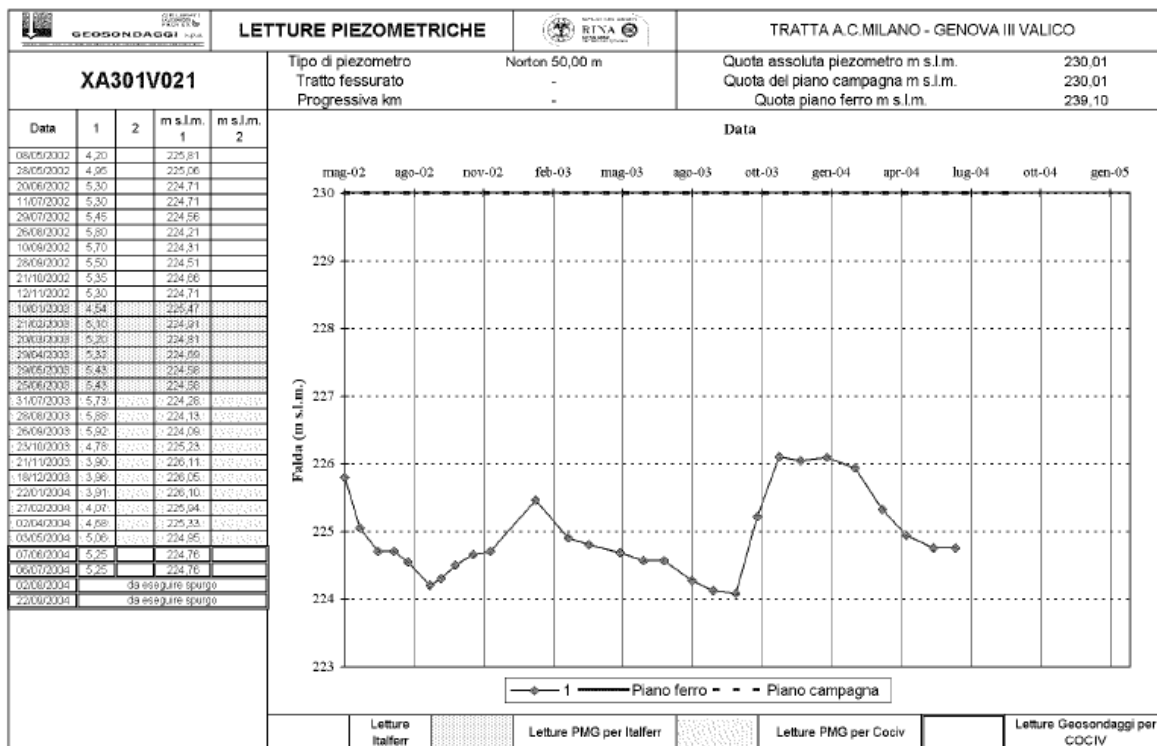
Figura 1 – Piezometro del sondaggio XA301V021 (Progetto Preliminare) Monitoraggio della falda nel periodo 8/5/2002 – 6/7/2004.
