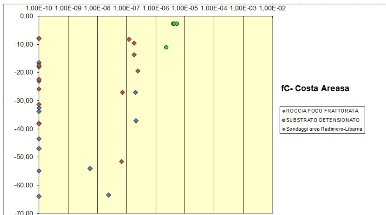
Figura 3 - Distribuzione dei valori di permeabilità ottenuti da prove in foro per la formazione di Costa Areasa (fCa), secondo la profondità (i valori pari a 1\text{E-}10 sono stati attribuiti indicativamente alle prove con assorbimento nullo, per significare che l'ammasso roccioso ha permeabilità bassissima, comunque inquadrabile nella classe AFTES minore, con K < 1\text{E-}8 ).
