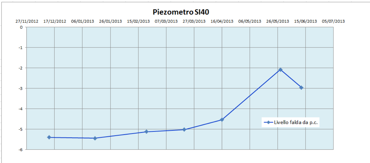
Figura 6 – Piezometro del sondaggio SI40 (Progetto Esecutivo – Lotto 1) Monitoraggio della falda nel periodo 13/12/2012 – 12/06/21013
