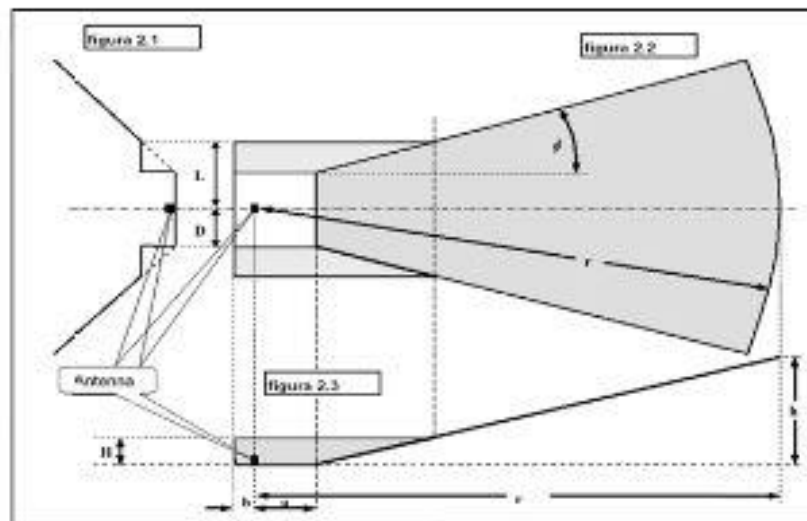
Figura 7 – BRA per apparati direzionali (Elementi base per la costruzione delle Building Restricted Areas ENAV/ENAC) Le dimensioni delle sopracitate superfici sono tabulate e riportate nel documento "Elementi base per la costruzione delle Building Restrcted Areas" disponibile dal sito di ENAC. La valutazione delle possibili interferenze con le Building Restricted Areas è stata effettuata con il supporto dell'utility di pre-analisi di ENAV: il risultato è che il progetto non interferisce con tali aree.
