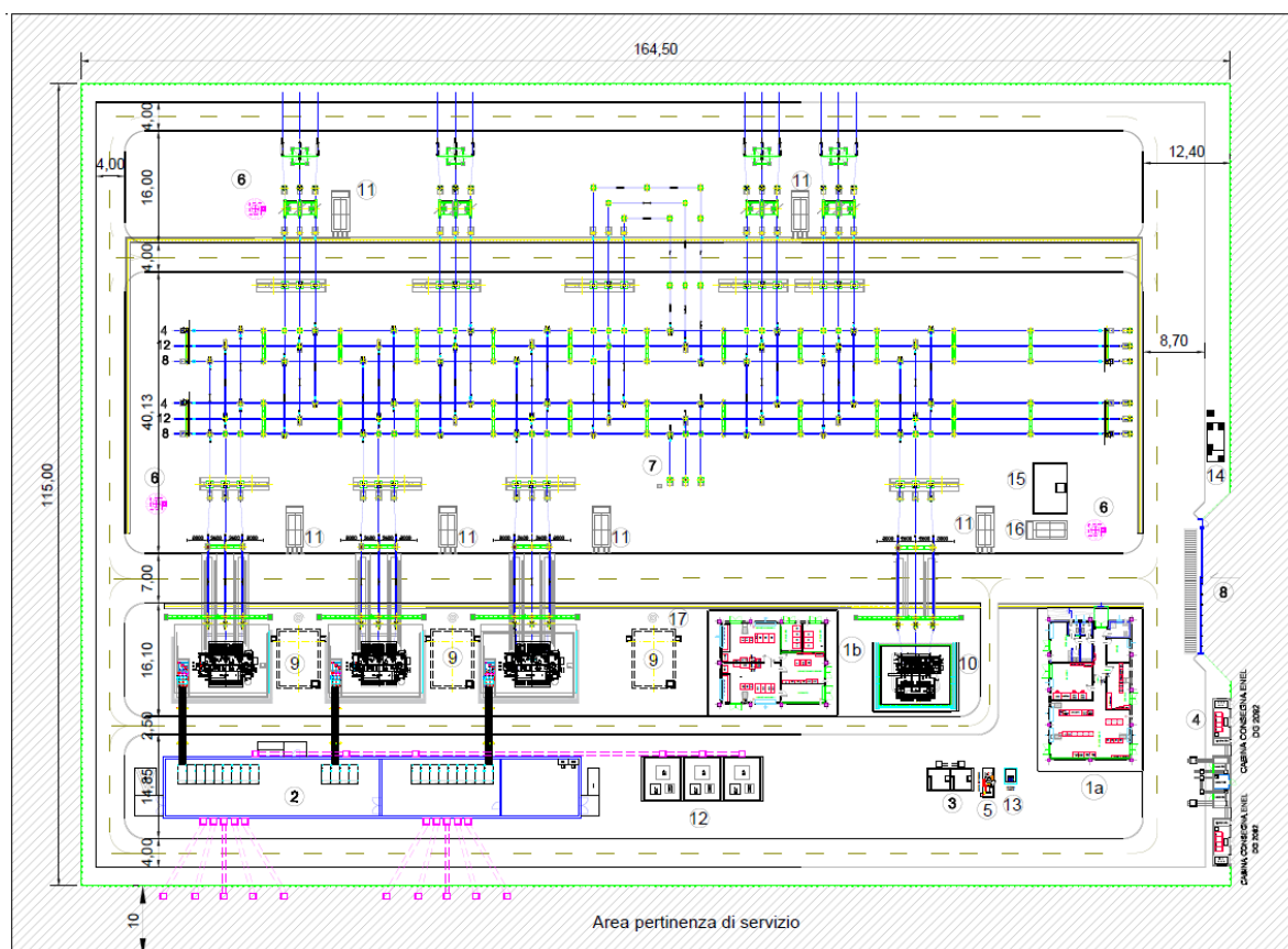
Fig.1 Planimetria elettromeccanica SE Buseto 2
