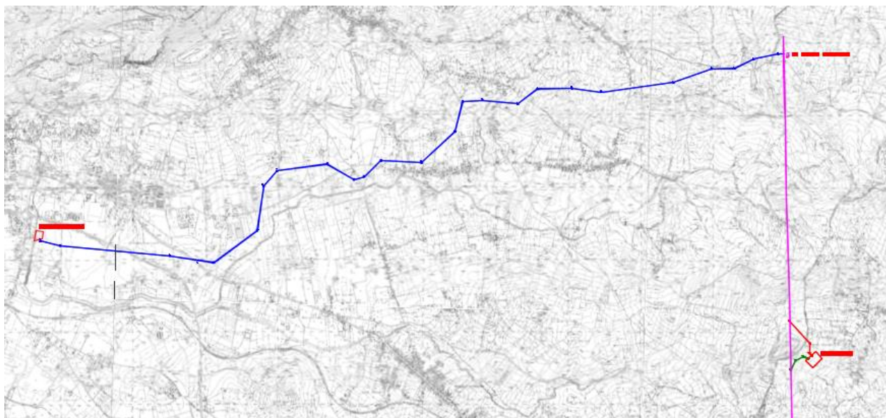
Figura 3: Tracciato elettrodotto 150 kV "Buseto-CP Ospedaletto"
