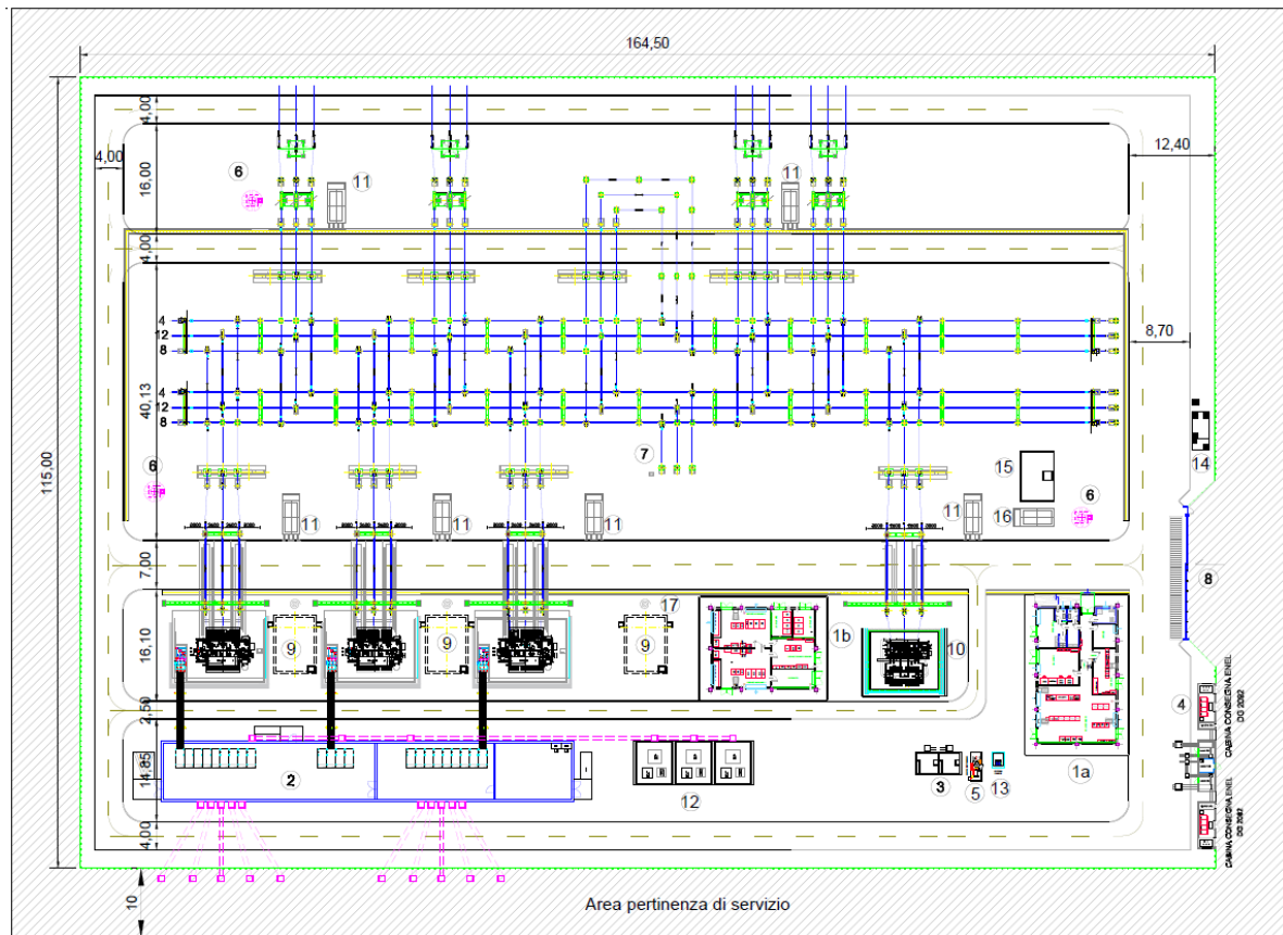
Fig.1 Planimetria elettromeccanica SE Busetto 2
