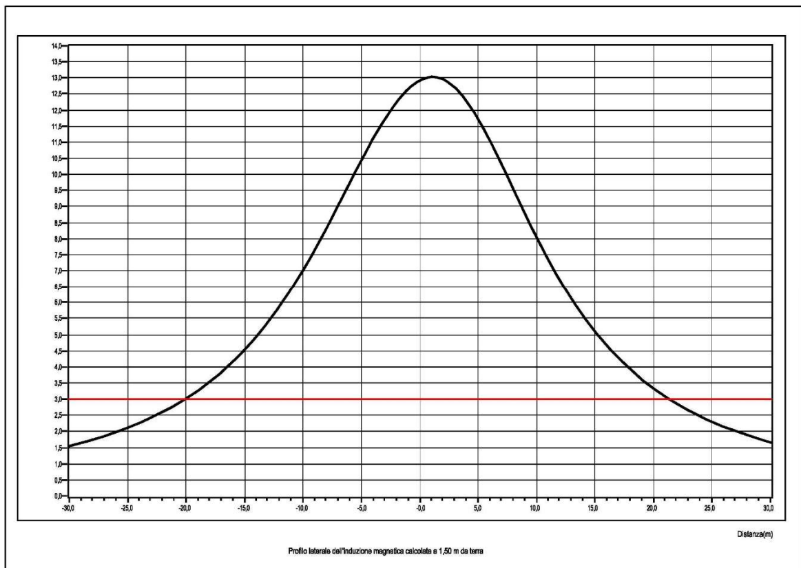
Figura 1: andamento dell'induzione magnetica in una sezione perpendicolare agli assi delle linee, calcolata ad 1,5 m dal suolo nel caso di franco minimo pari a 10,0 m per il sostegno di amarro con mensole a triangolo (in rosso l'obiettivo di qualità pari a 3 µT).
