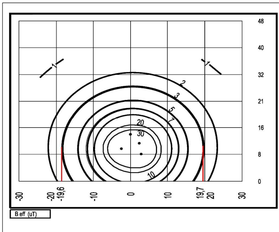
Figura 3: Curve di isocampo a 3 \mu\text{T} in una sezione perpendicolare all'asse linea per un sostegno in amarro con mensole disposte a triangolo. DPA = 19,70m.
