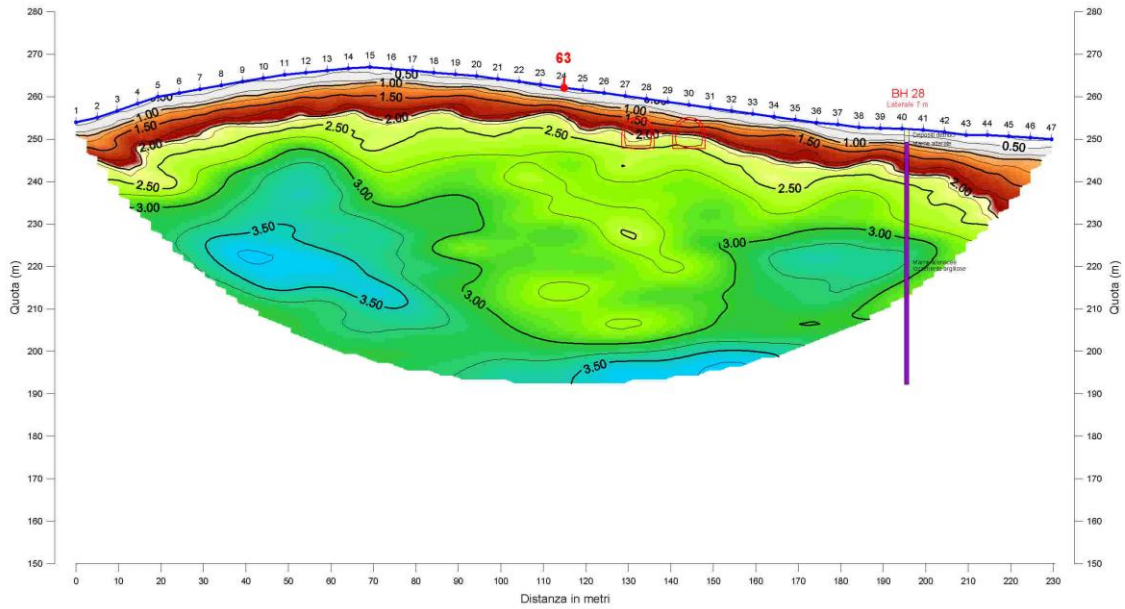
Figura 6-3 Linea tomografica 62
