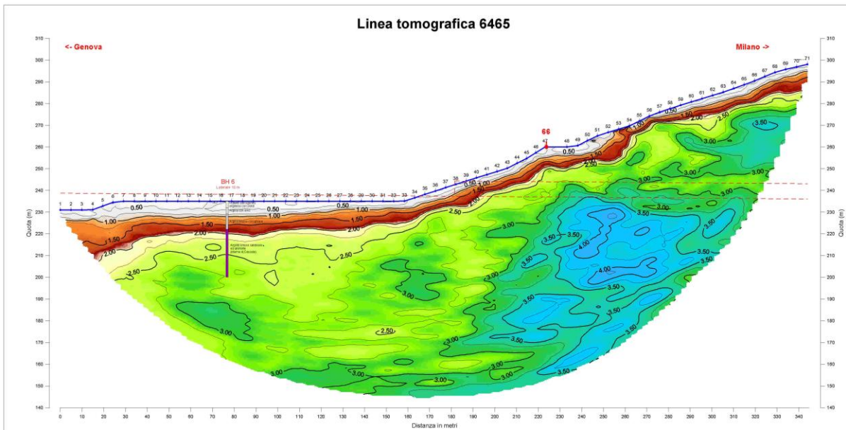
Figura 6-5 Linea tomografica 64-65
