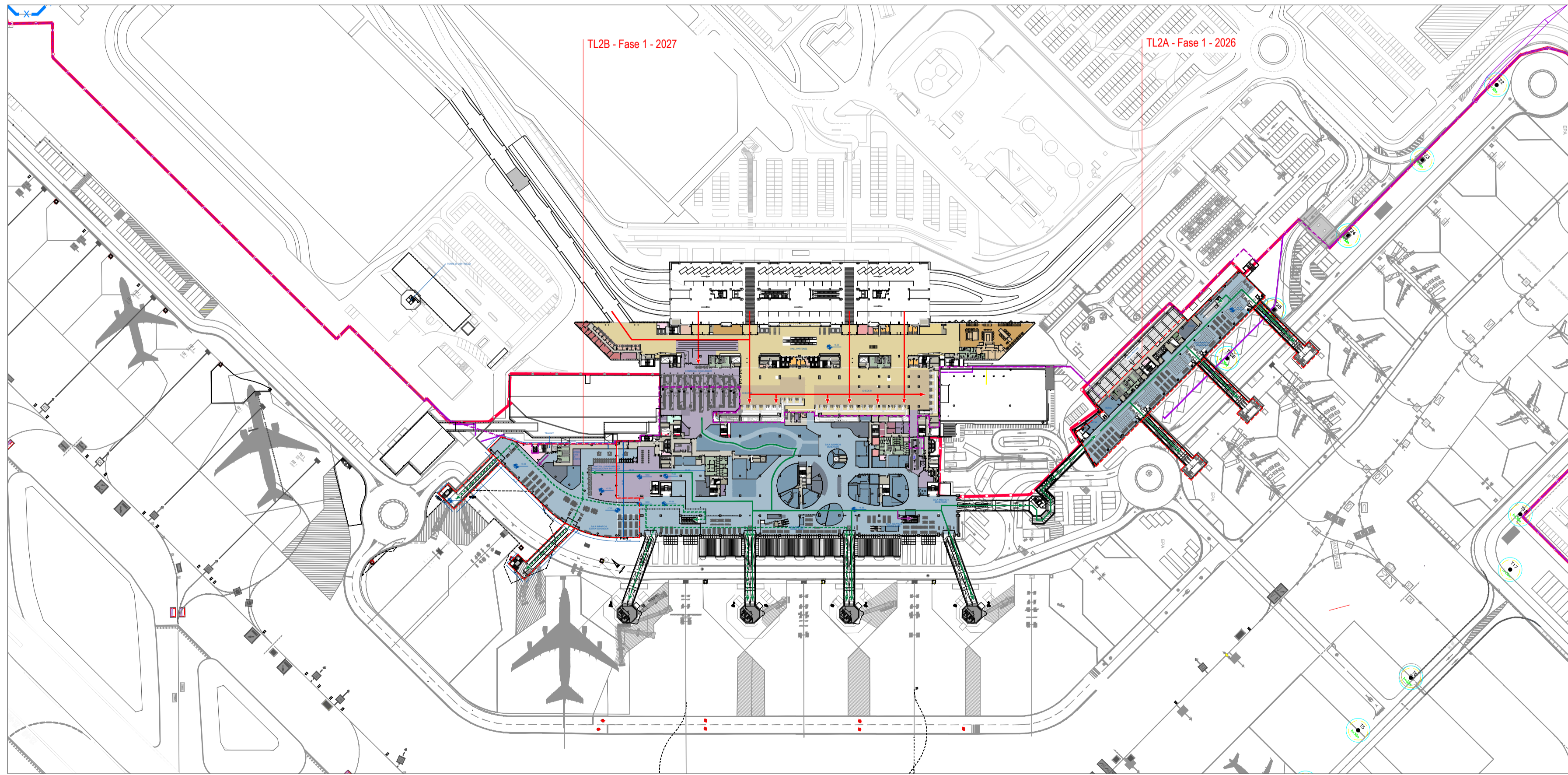
3 Pianta Piano Primo - Terminal - 2028 Sc. 1:2000
