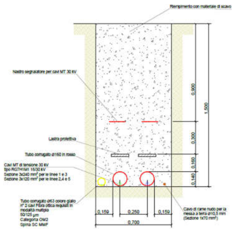
Sezione E-E' - Cavidotto MT-BT interno scala 1:20
