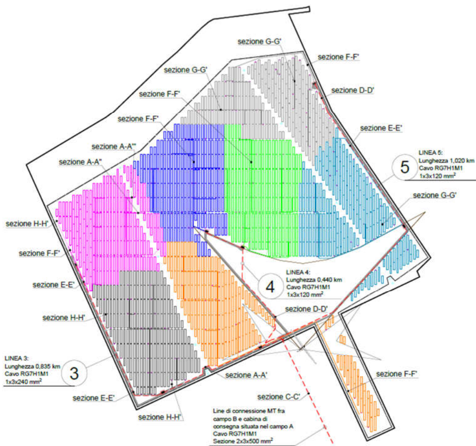
Layout generale cavidotti impianto - Campo B scala 1:5.000
