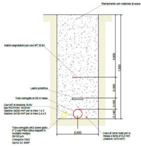
Sezione D-D' - Cavidotto MT interno scala 1:20
