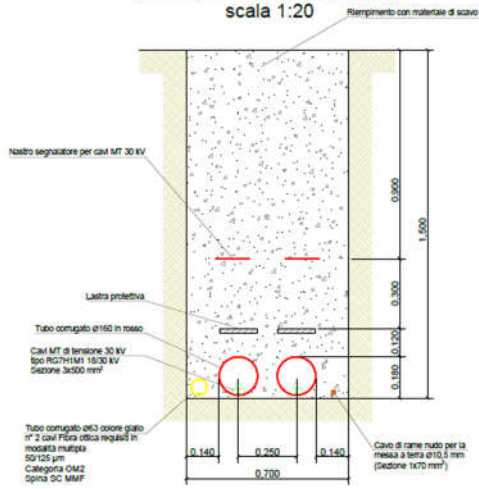
Sezione C-C' - Cavidotto MT di collegamento fra campo B e cabina di raccolta scala 1:20
