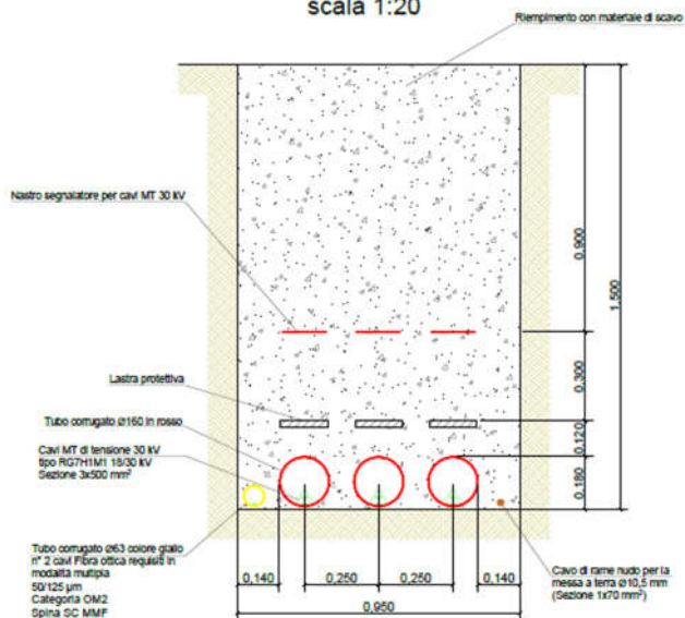
Sezione B-B' - Cavidotto MT esterno scala 1:20
