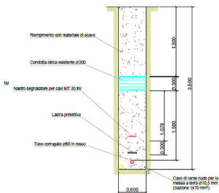
Sezione A-A''' - Interferenza dorsale BT secondaria con singola linea con condotta idrica esistente scala 1:50
