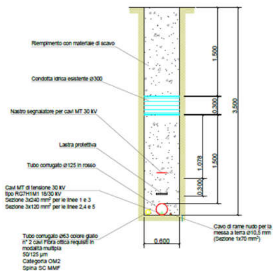
Sezione A-A - Interferenza cavidotto MT interno con condotta idrica esistente scala 1:50
