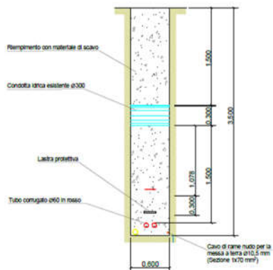
Sezione A-A'' - Interferenza dorsale BT secondaria con doppia linea con condotta idrica esistente scala 1:50
