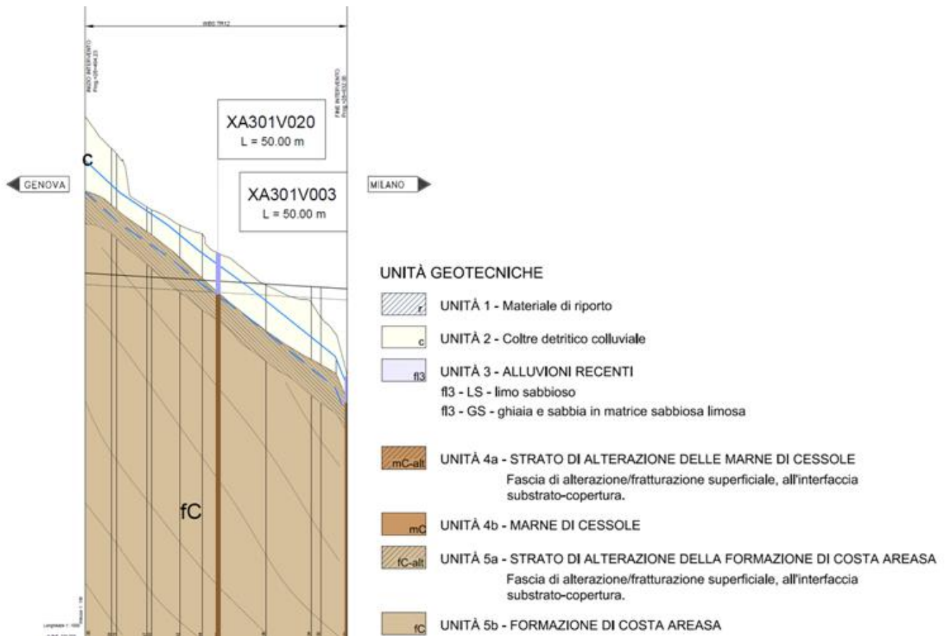
Figura 7-1 Profilo geologico TR12
