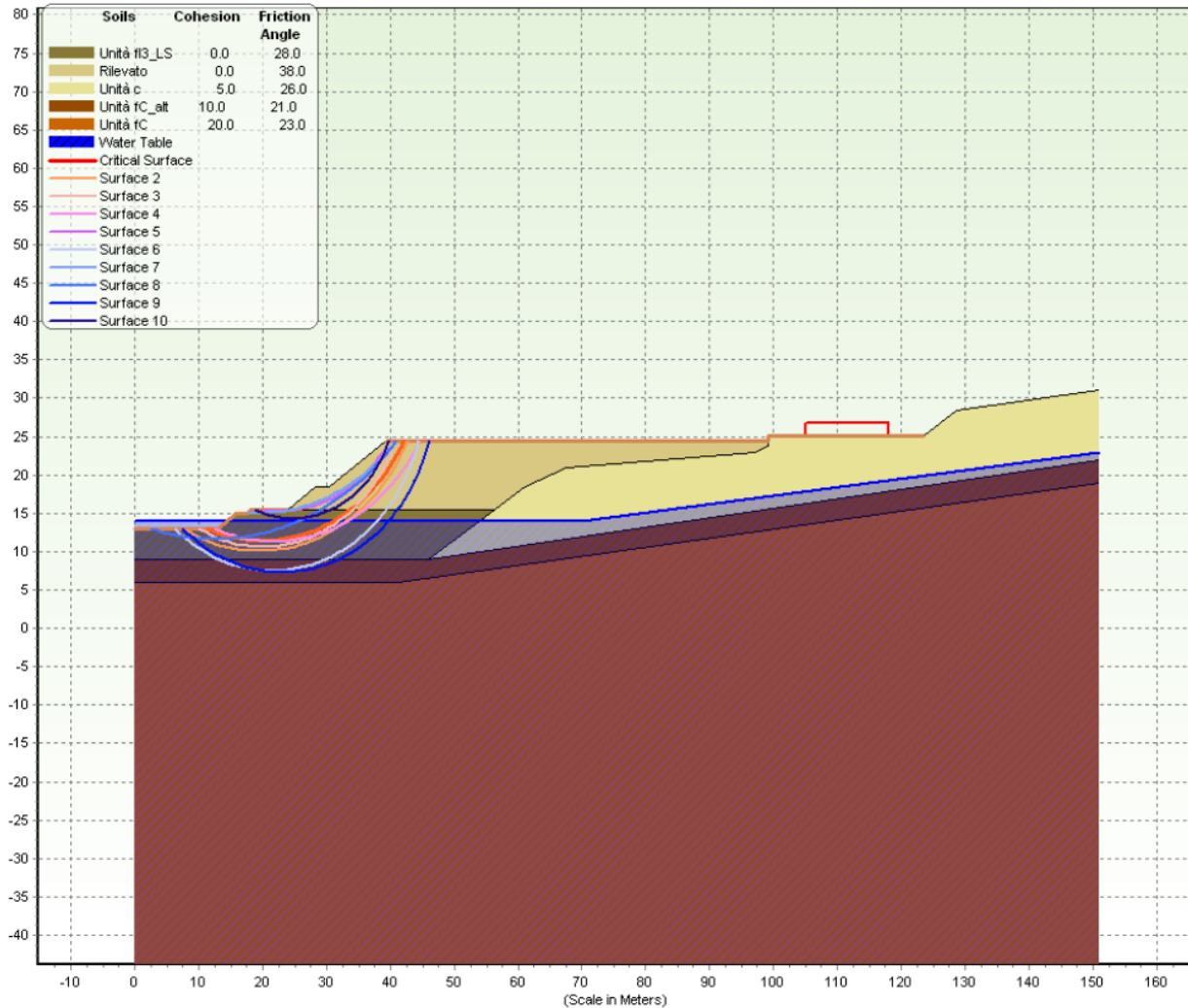
Figura 5-3 TR12 – Verifica di stabilità globale condizioni statiche sezione pk 28+550
