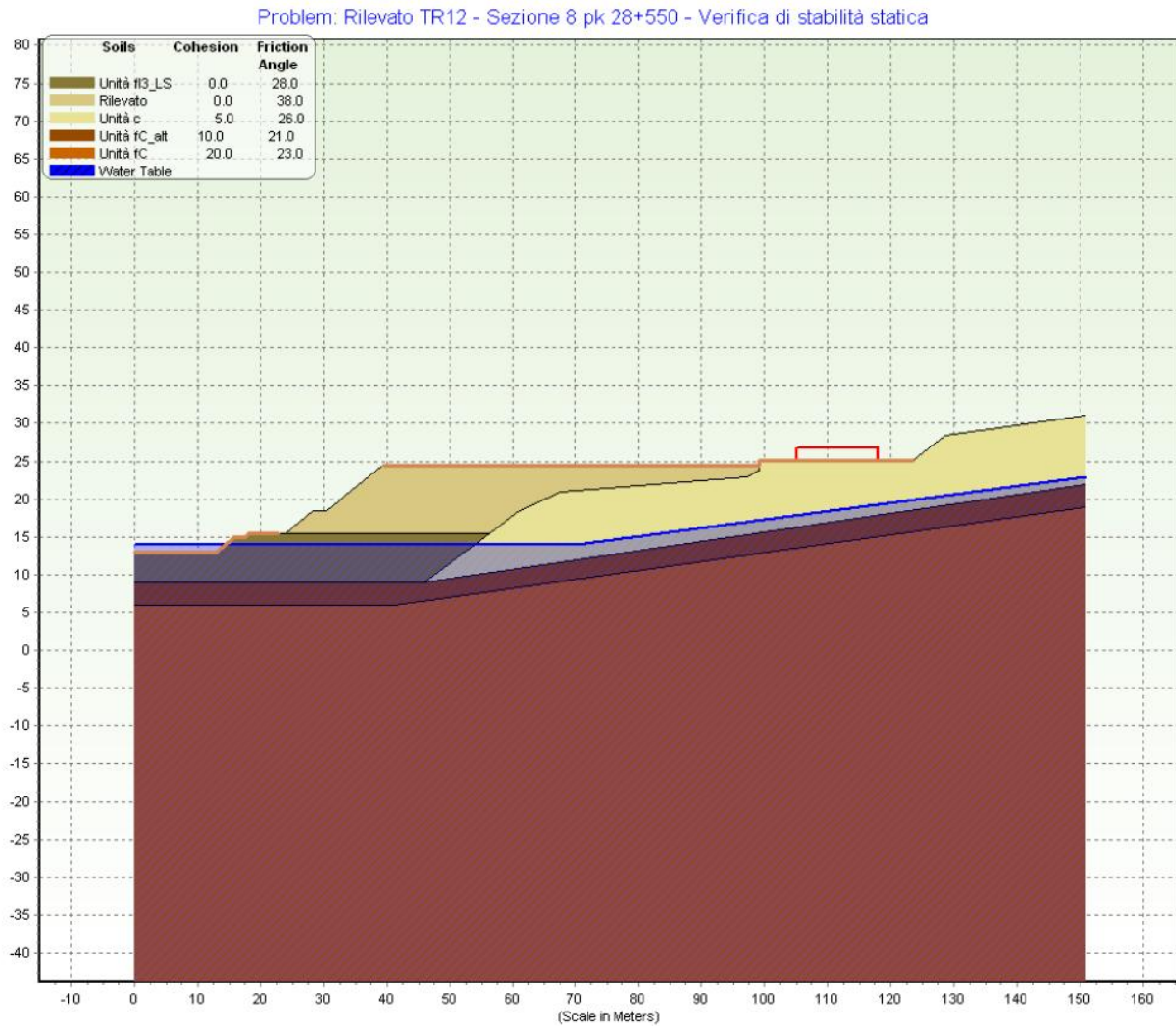
Figura 5-2 TR12 – Geometria della sezione di calcolo pk 28+550
