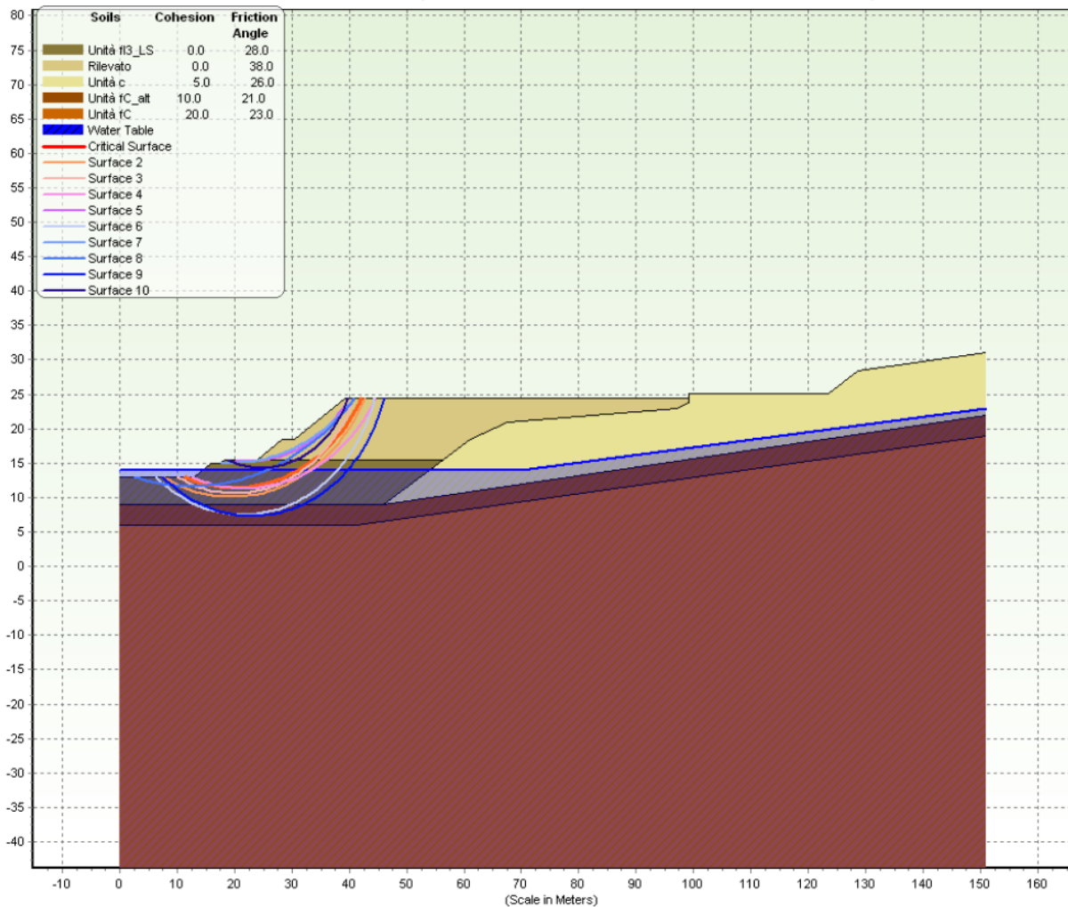
Figura 5-4 TR12 – Verifica di stabilità globale condizioni sismiche sezione pk 28+550
