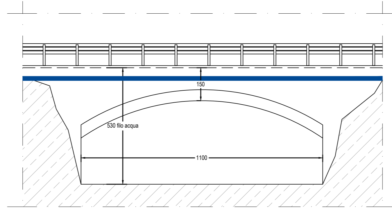
Sezione trasversale - 1:100
