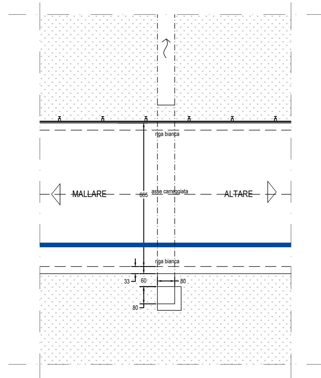
Planimetria generale attraversamento - 1:100
