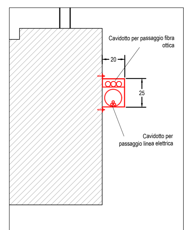
Particolare costruttivo - 1:20
