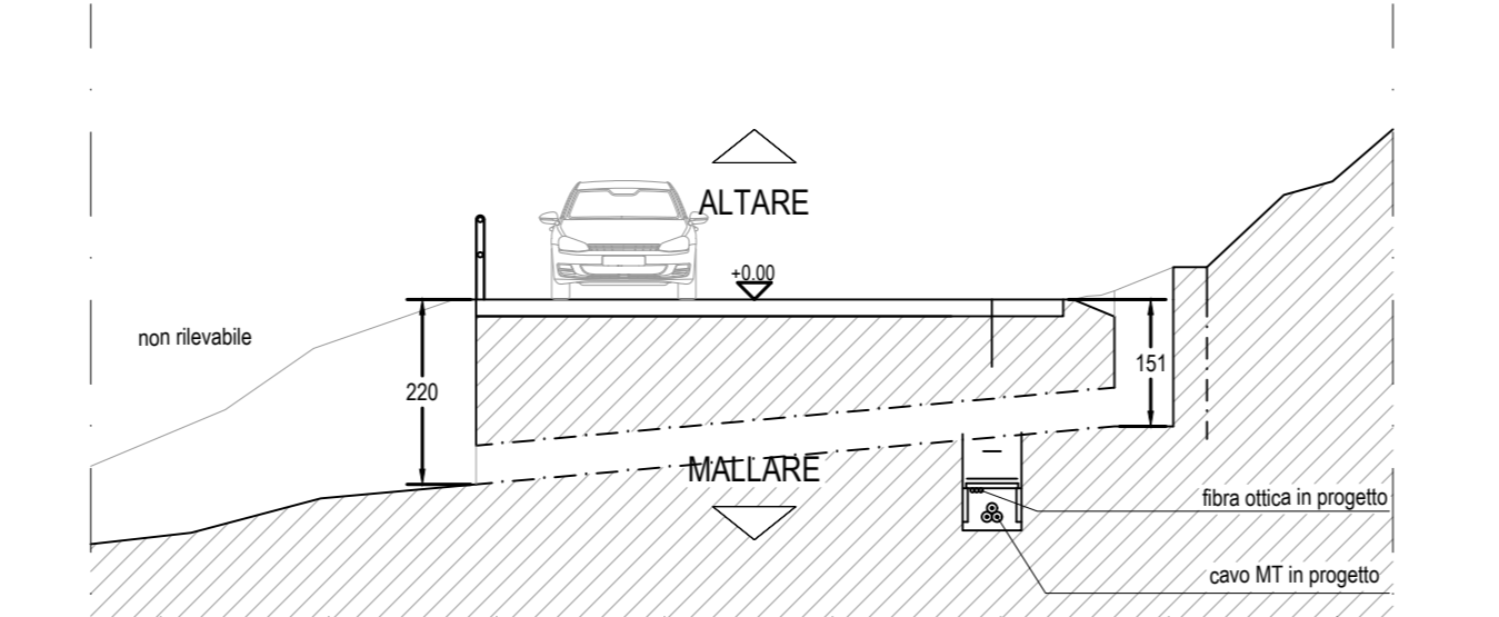
Sezione trasversale - 1:100
