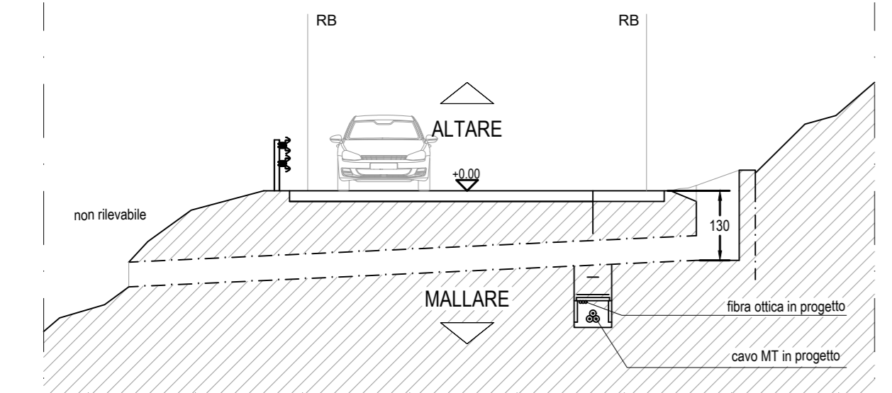
Sezione trasversale - 1:100
