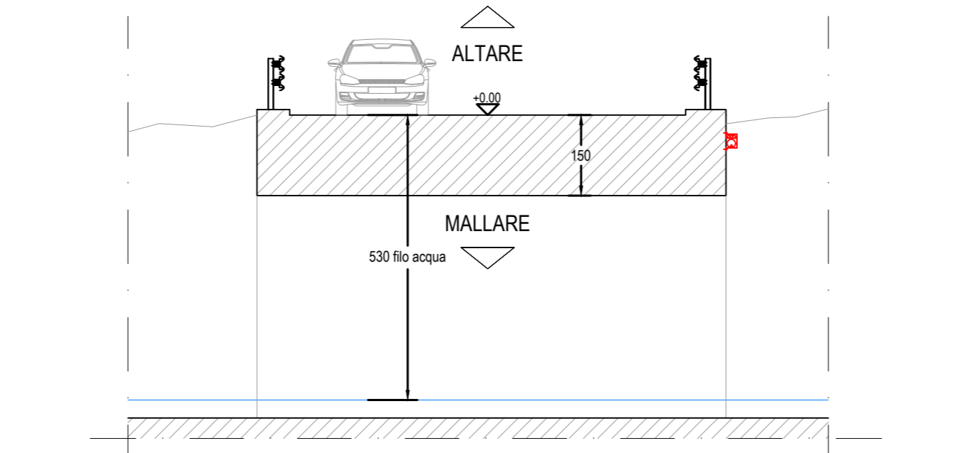
Sezione trasversale - 1:100
