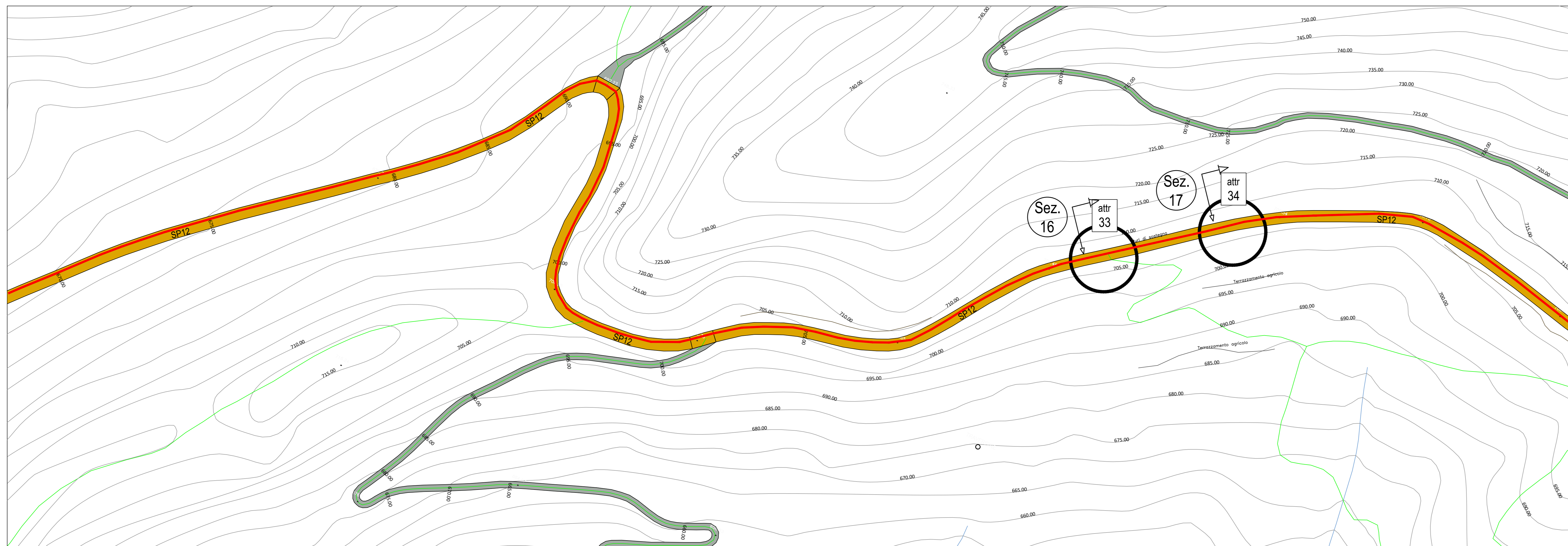
PLANIMETRIA DI INTERVENTO 13 base CTR - scala 1:1000
