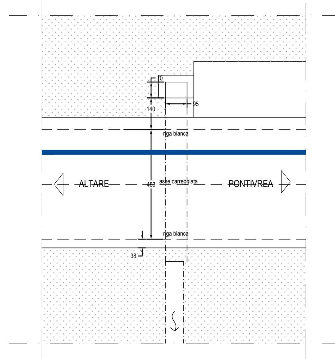
Planimetria generale attraversamento - 1:100
