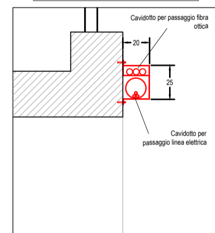
Particolare costruttivo - 1:20
