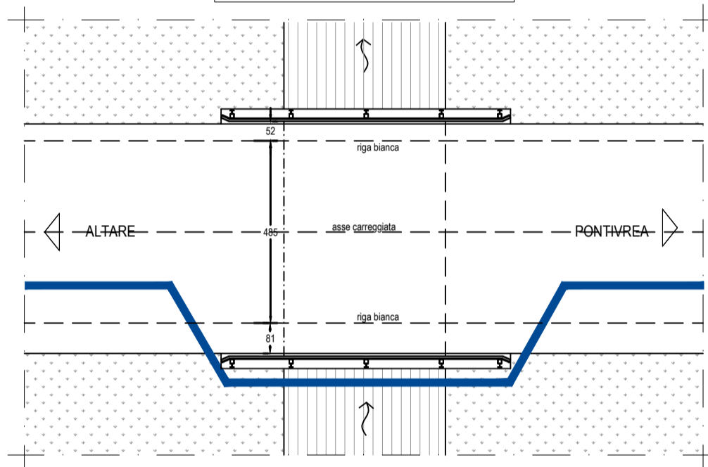
Planimetria generale attraversamento - 1:100
