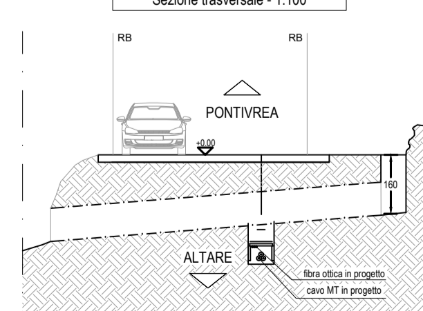
Sezione trasversale - 1:100
