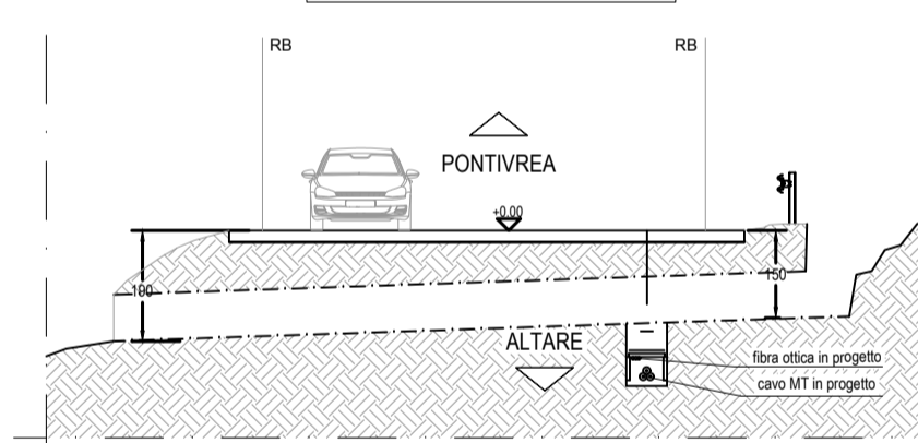
Sezione trasversale - 1:100
