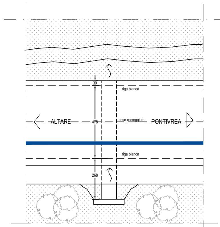
Planimetria generale attraversamento - 1:100
