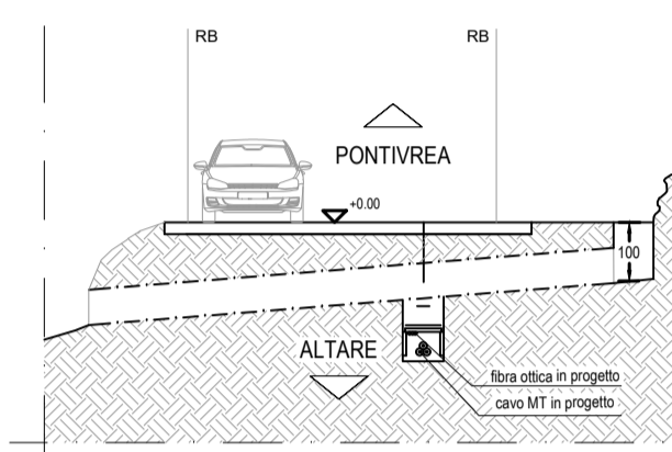
Sezione trasversale - 1:100
