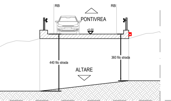
Sezione trasversale - 1:100
