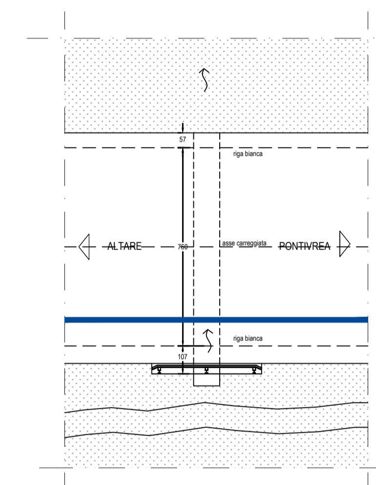
Planimetria generale attraversamento - 1:100
