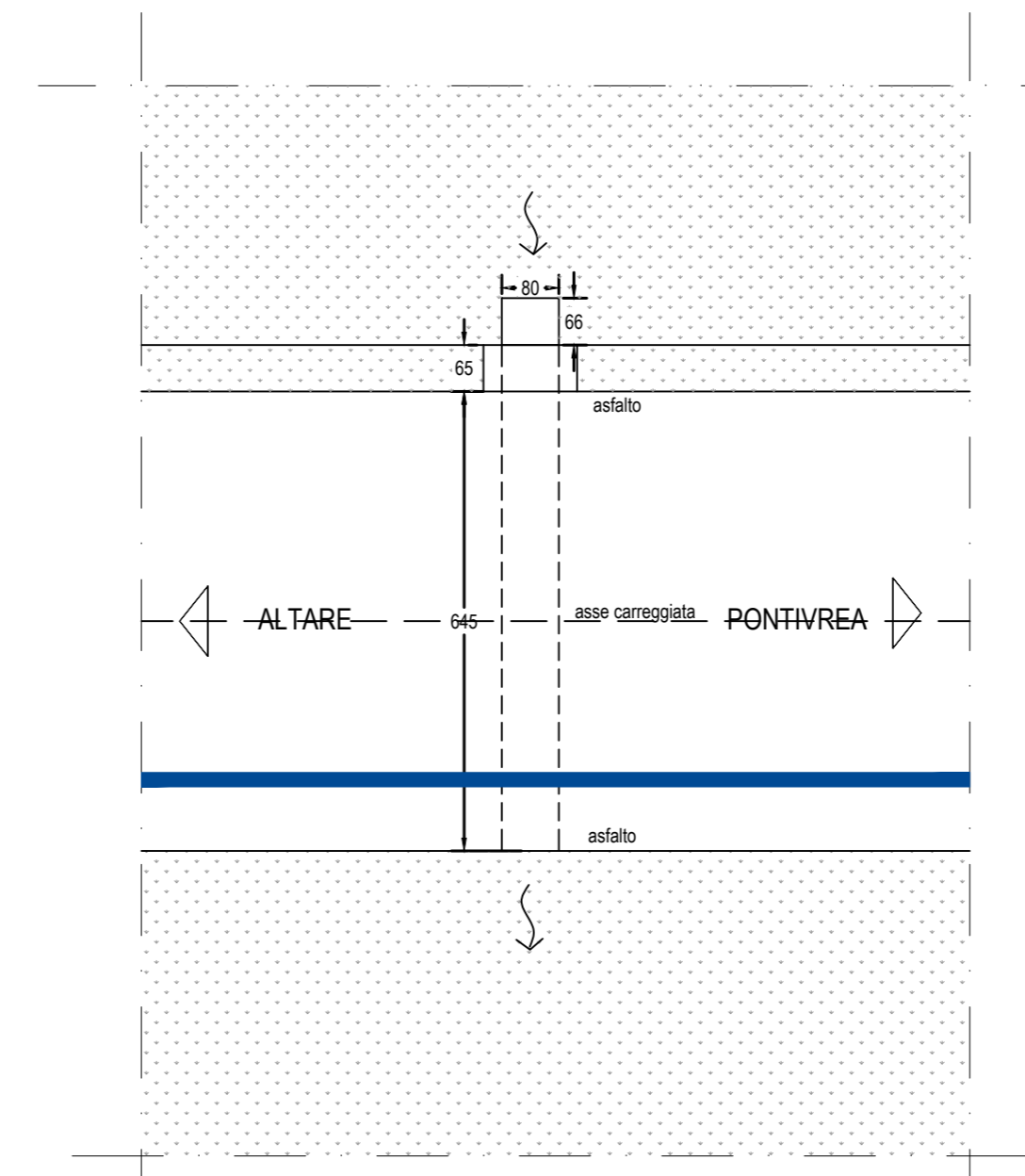
Planimetria generale attraversamento - 1:100
