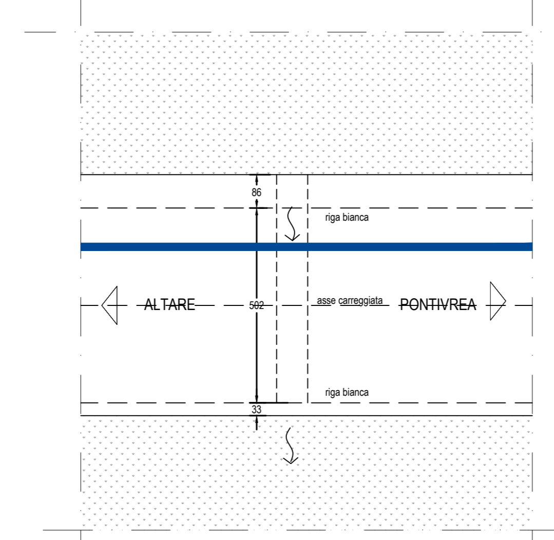
Planimetria generale attraversamento - 1:100
