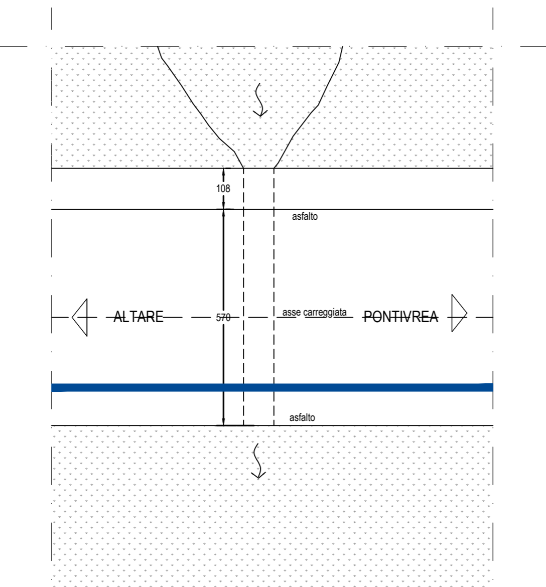
Planimetria generale attraversamento - 1:100
