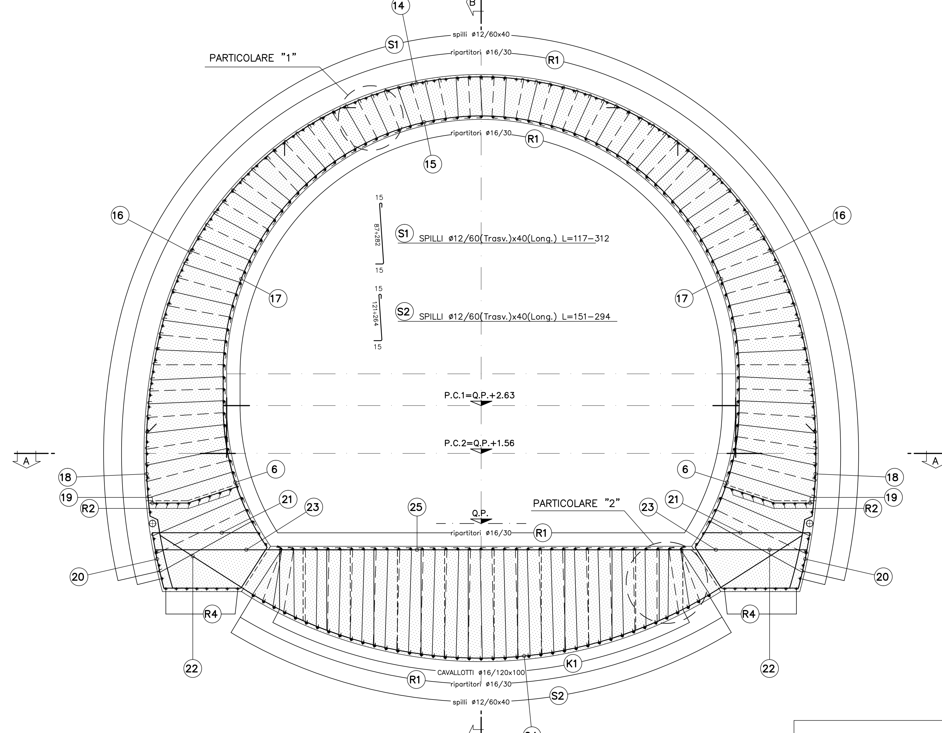
SEZIONE D-D SCALA 1:50
