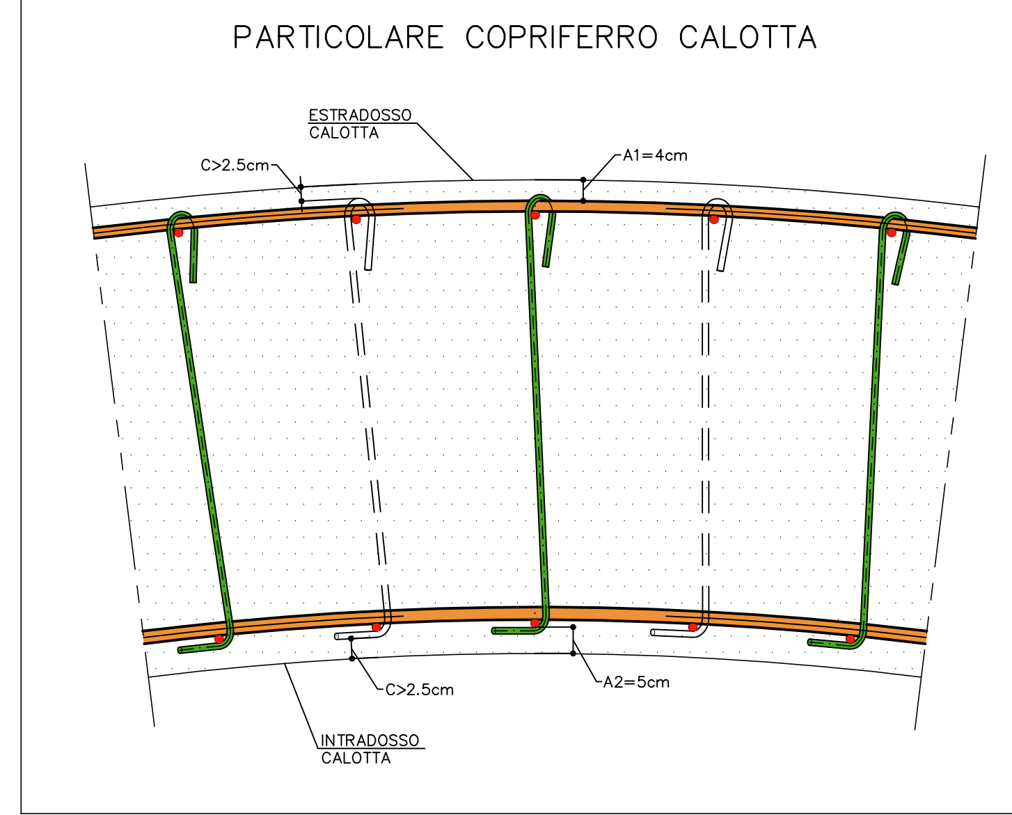
PARTICOLARE "1" SCALA 1:10
