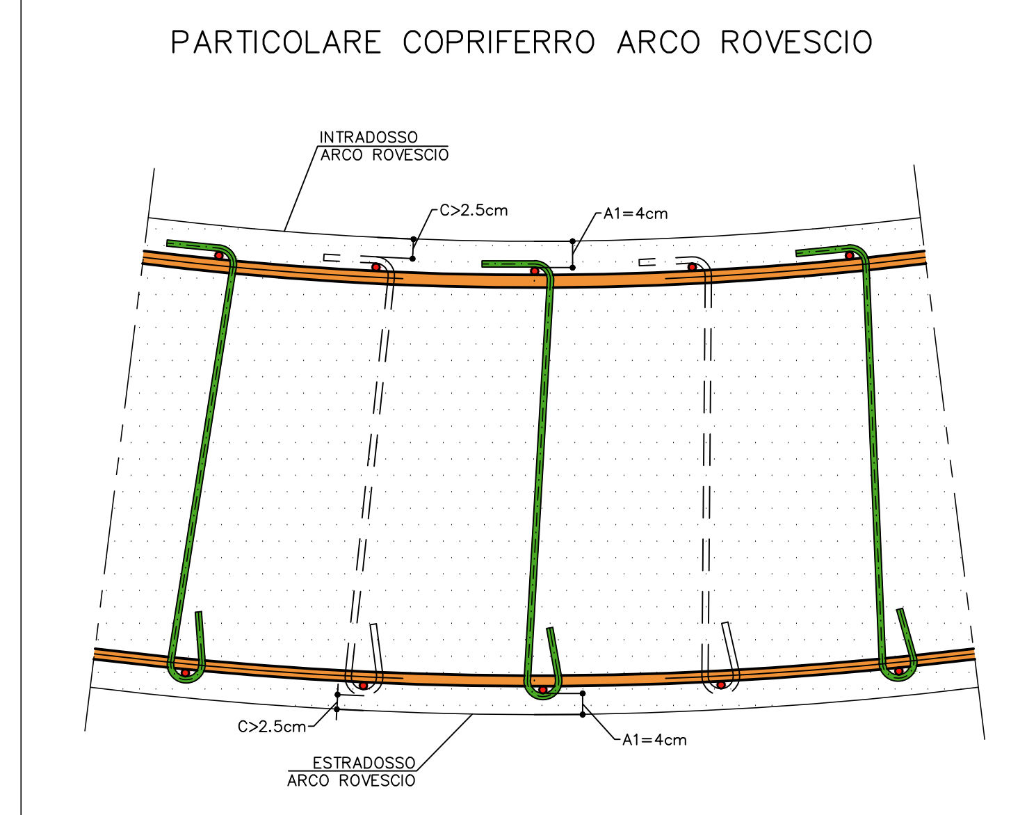
PARTICOLARE "2" SCALA 1:10
