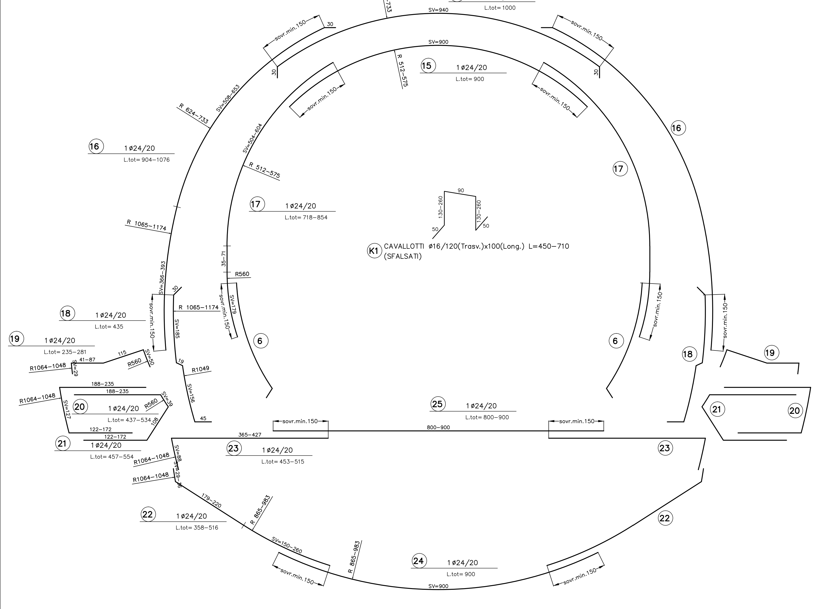
ESPLOSO
