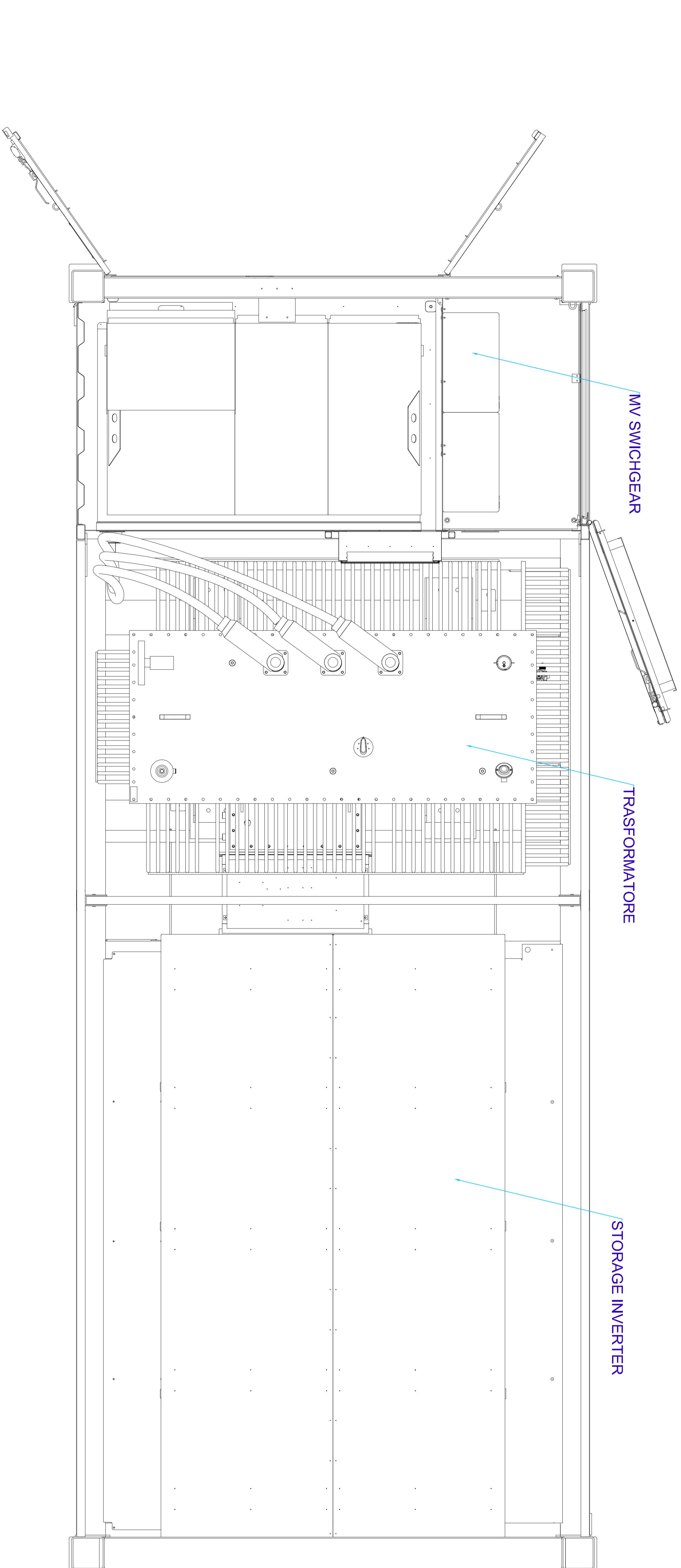
PROSPETTO DALL'ALTO SPS (VISTA CON COMPONENTI)
