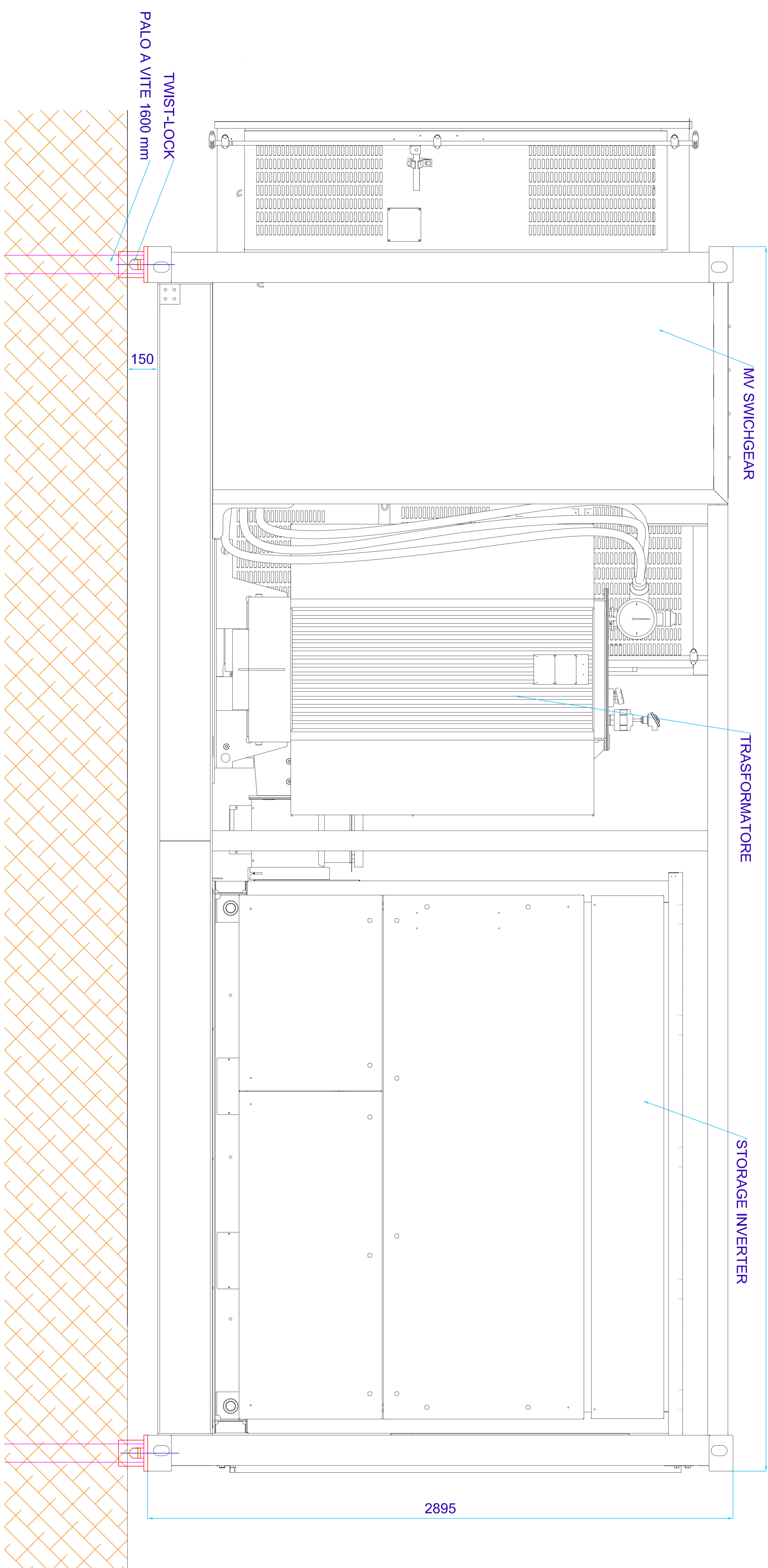
PROSPETTO LATERALE SPS (VISTA CON COMPONENTI)
