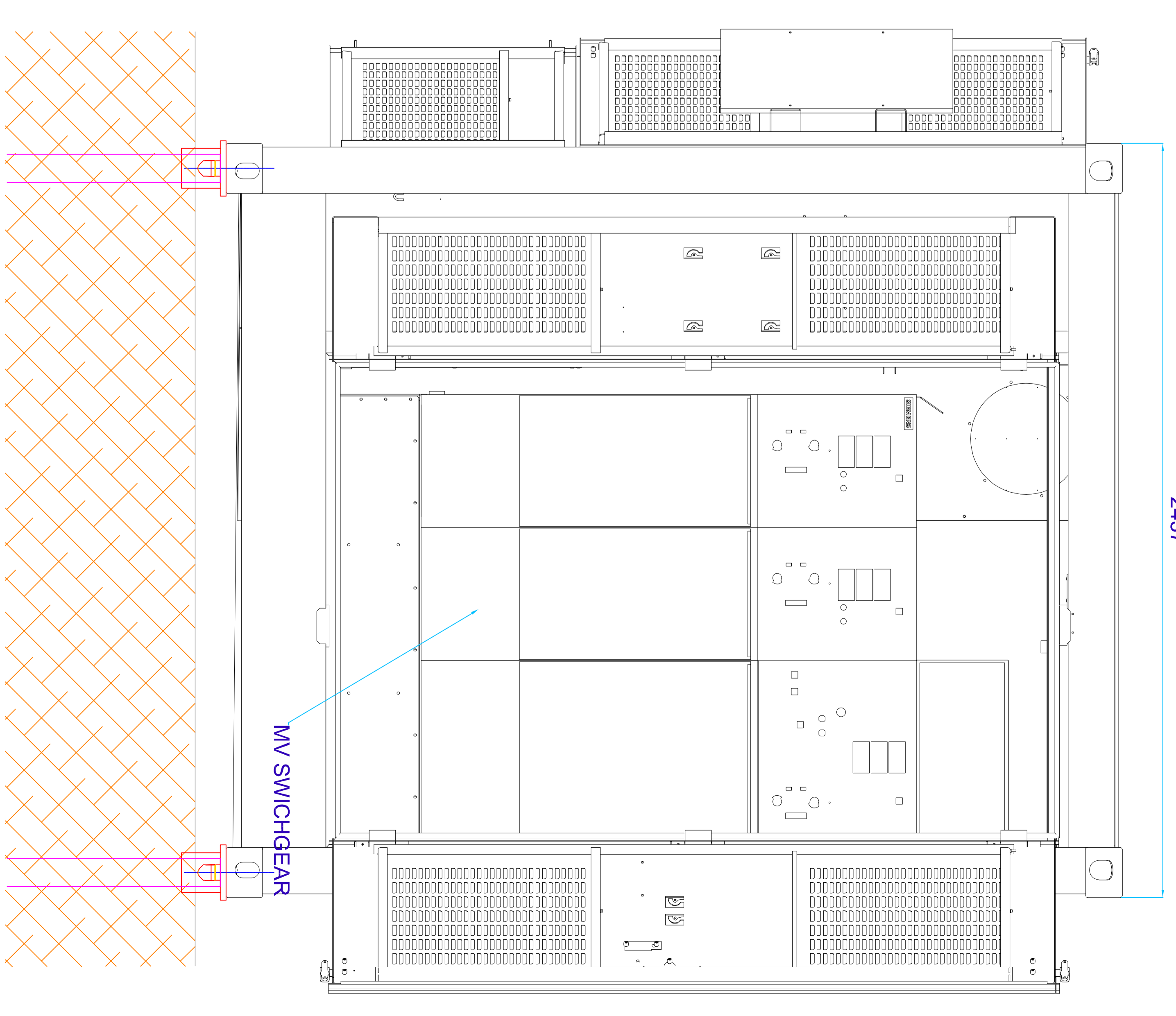
PROSPETTO FRONTALE SPS (VISTA CON COMPONENTI)
