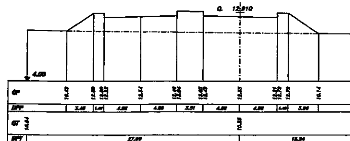
SEZIONE 281 PROGRESSIVA 23750.00
