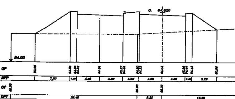
SEZIONE 845 PROGRESSIVA 58900.00
