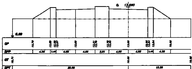
SEZIONE 276 PROGRESSIVA 23500.00
