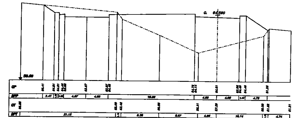
SEZIONE 990 PROGRESSIVA 87180.00
