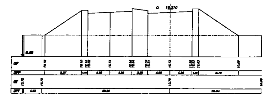
SEZIONE 266 PROGRESSIVA 23000.00
