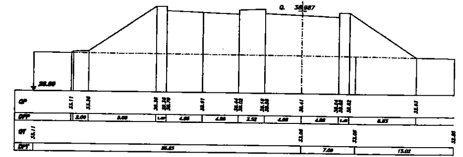
SEZIONE 576 PROGRESSIVA 41600.00
