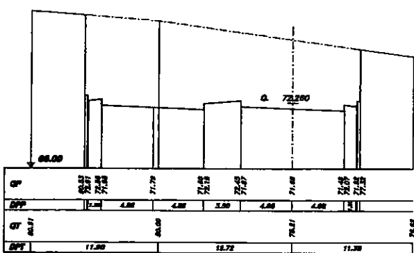
SEZIONE 839 PROGRESSIVA 58620.00
