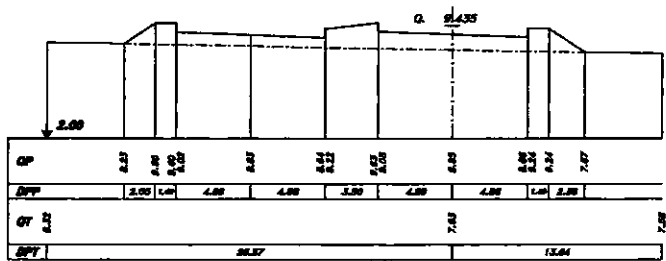
SEZIONE 231 PROGRESSIVA 21250.00
