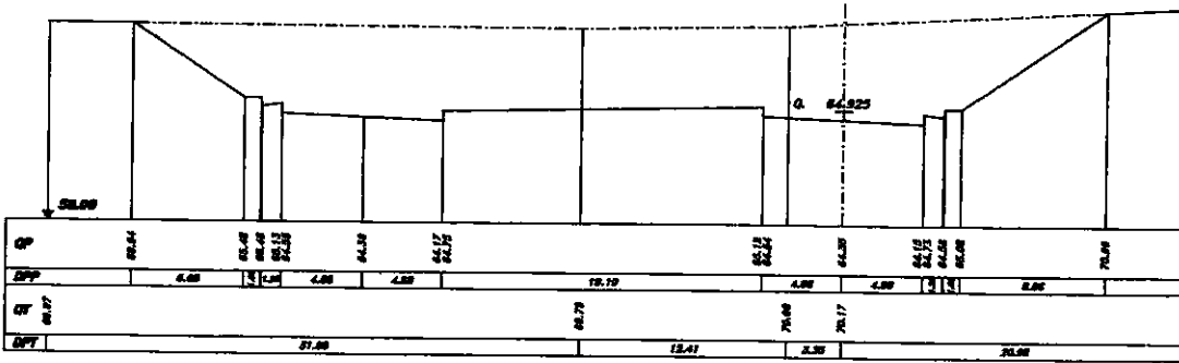
SEZIONE 987 PROGRESSIVA 86180.00
