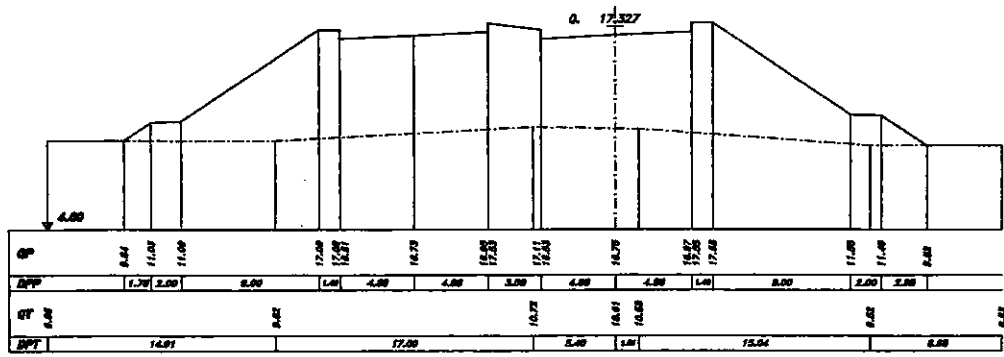
SEZIONE 260 PROGRESSIVA 22700.00
