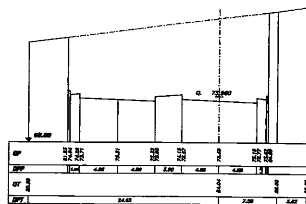
SEZIONE 836 PROGRESSIVA 58500.00
