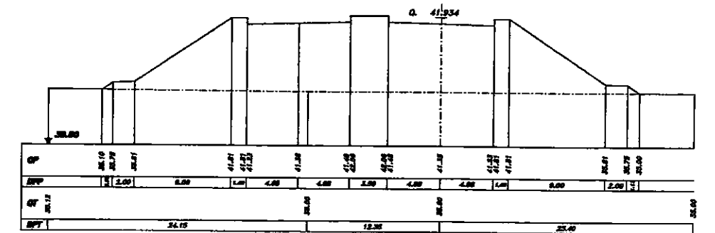
SEZIONE 77 PROGRESSIVA 6270.00
