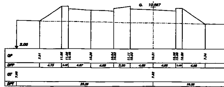
SEZIONE 229 PROGRESSIVA 21150.00
