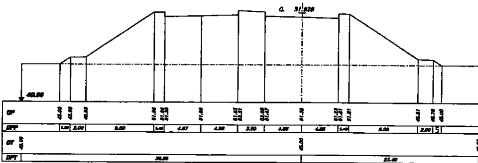
SEZIONE 792 PROGRESSIVA 54078.00
