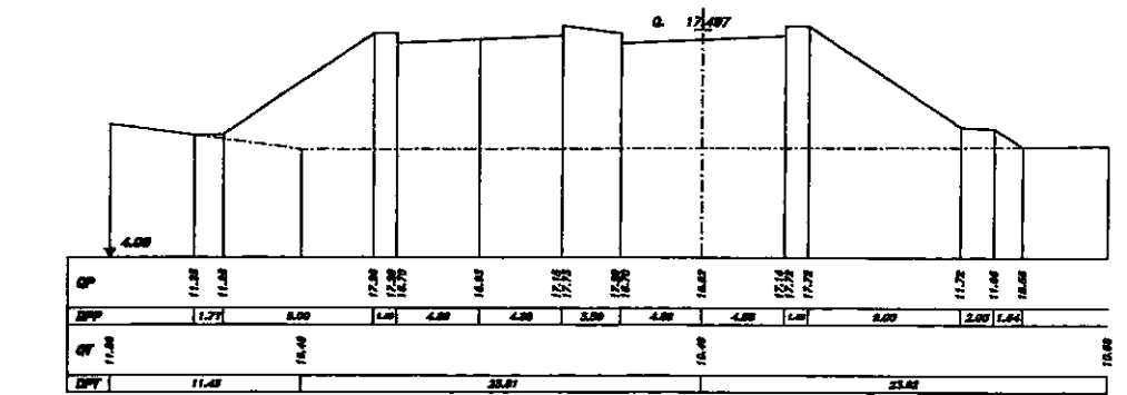
SEZIONE 263 PROGRESSIVA 22800.00
