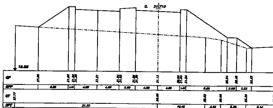
SEZIONE 886 PROGRESSIVA 59200.00
