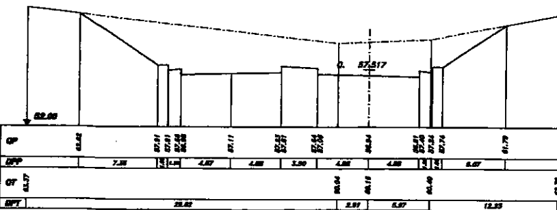
SEZIONE 798 PROGRESSIVA 54300.00
