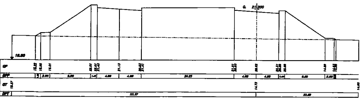
SEZIONE 191 PROGRESSIVA 14050.00
