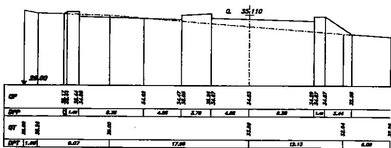
SEZIONE 882 PROGRESSIVA 59050.00
