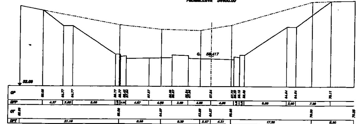
SEZIONE 799 PROGRESSIVA 54400.00
