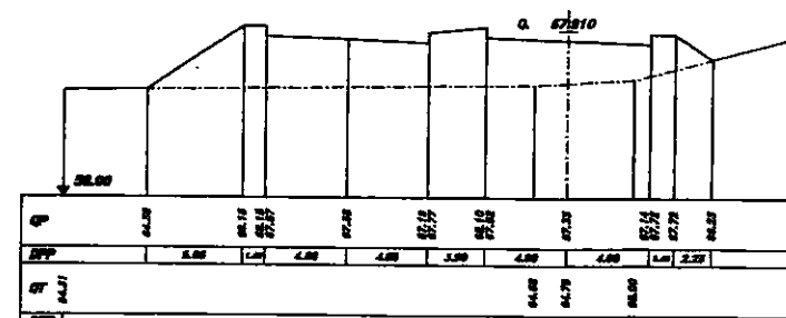
SEZIONE 843 PROGRESSIVA 58800.00
