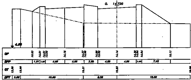
SEZIONE 270 PROGRESSIVA 23300.00
