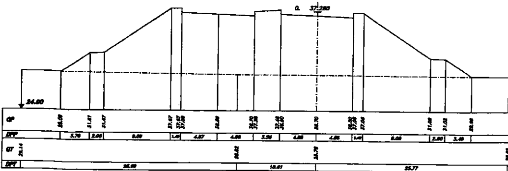
SEZIONE 580 PROGRESSIVA 42000.00
