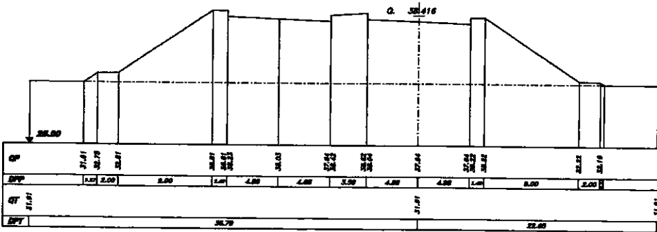
SEZIONE 574 PROGRESSIVA 41600.00
