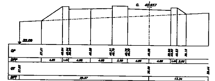
SEZIONE 74 PROGRESSIVA 5900.00
