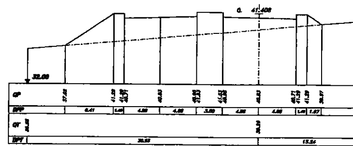
SEZIONE 73 PROGRESSIVA 5750.00
