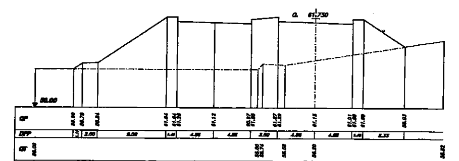
SEZIONE 847 PROGRESSIVA 58960.00
