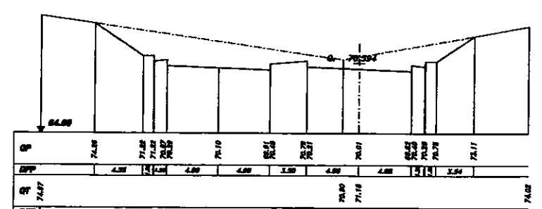
SEZIONE 841 PROGRESSIVA 58700.00
