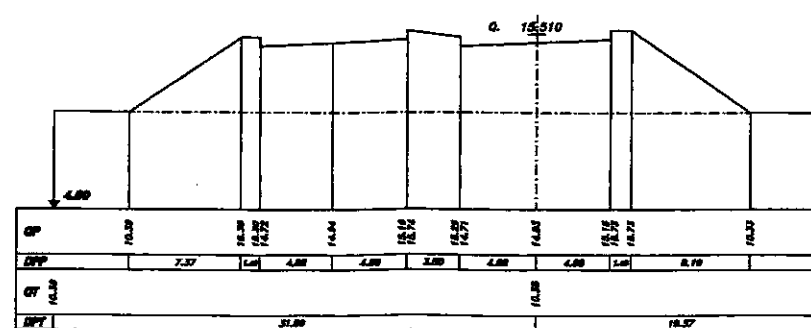
SEZIONE 268 PROGRESSIVA 23100.00
