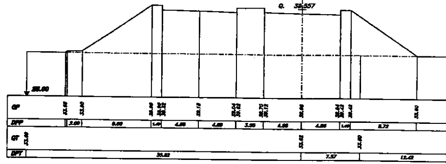
SEZIONE 575 PROGRESSIVA 41600.00
