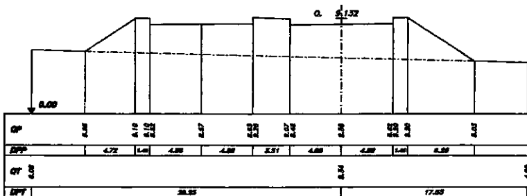
SEZIONE 234 PROGRESSIVA 21400.00
