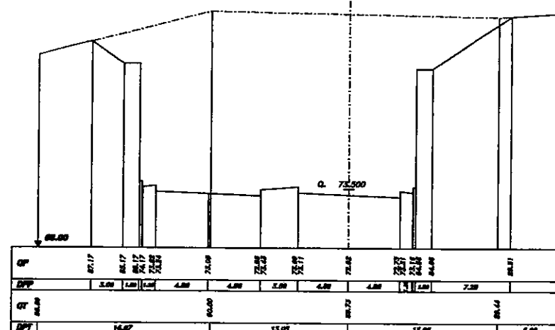
SEZIONE 837 PROGRESSIVA 58540.00
