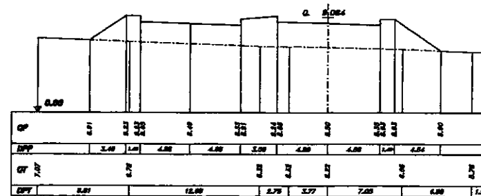
SEZIONE 232 PROGRESSIVA 21300.00
