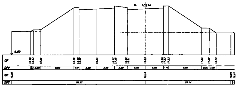
SEZIONE 267 PROGRESSIVA 23050.00
