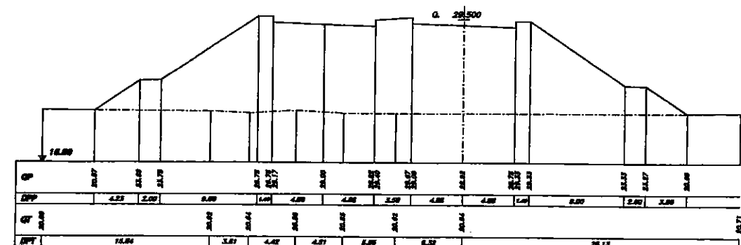
SEZIONE 890 PROGRESSIVA 59450.00
