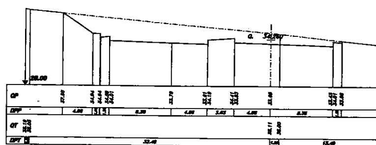
SEZIONE 883 PROGRESSIVA 59100.00
