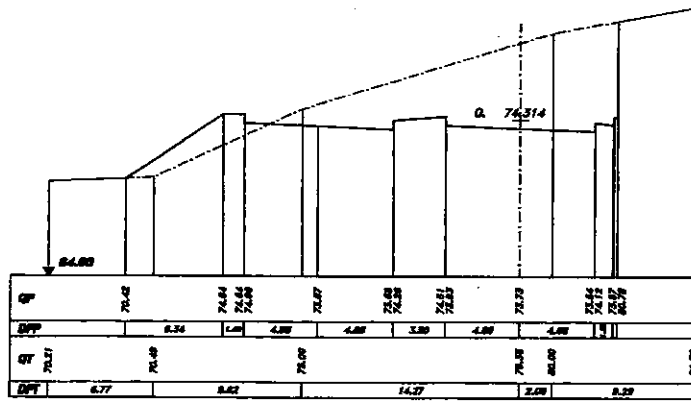
SEZIONE 839 PROGRESSIVA 58620.00
