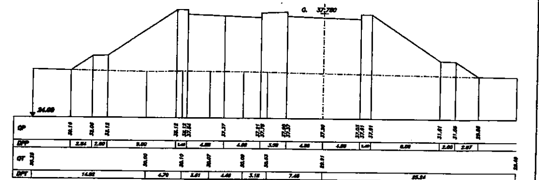
SEZIONE 581 PROGRESSIVA 42000.00
