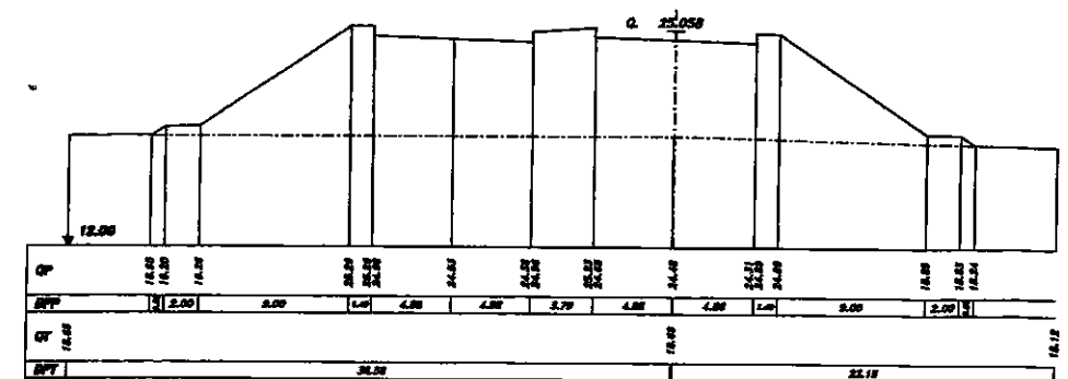
SEZIONE 890 PROGRESSIVA 59450.00
