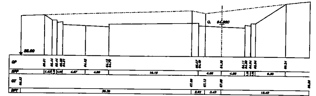
SEZIONE 984 PROGRESSIVA 85790.00
