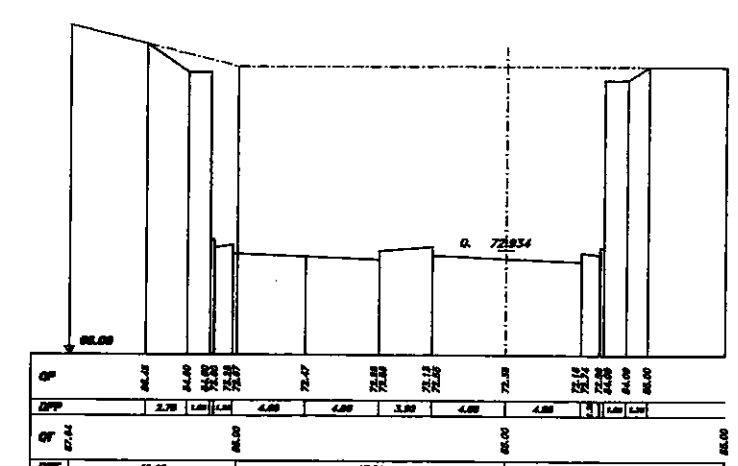
SEZIONE 838 PROGRESSIVA 58580.00
