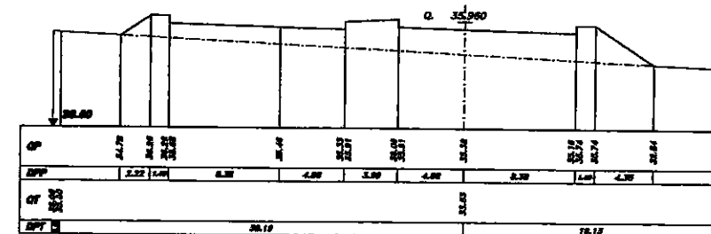
SEZIONE 884 PROGRESSIVA 59150.00
