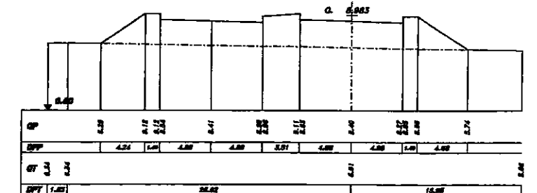
SEZIONE 233 PROGRESSIVA 21350.00
