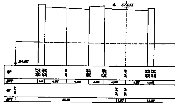
SEZIONE 578 PROGRESSIVA 41770.00
