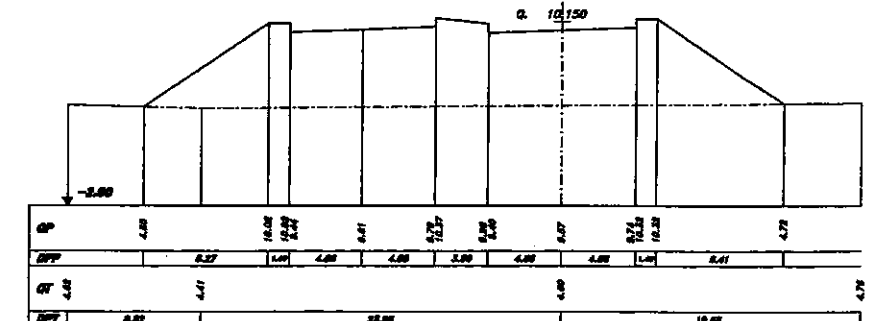
SEZIONE 236 PROGRESSIVA 21500.00
