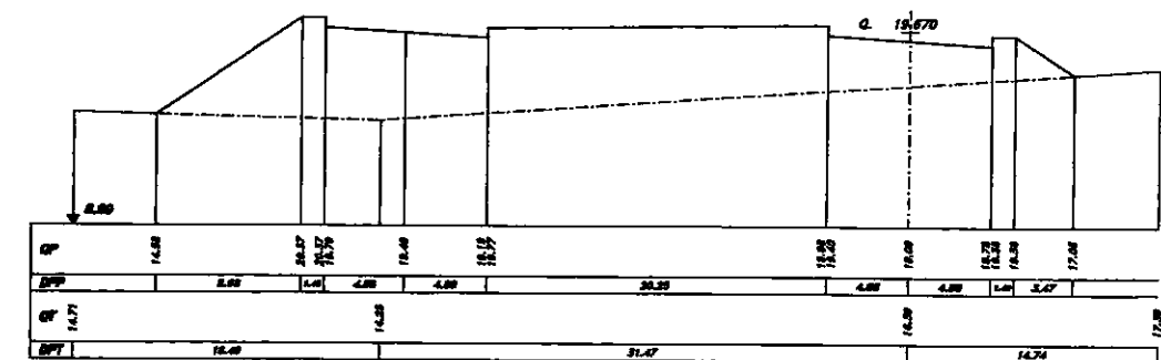
SEZIONE 190 PROGRESSIVA 14000.00
