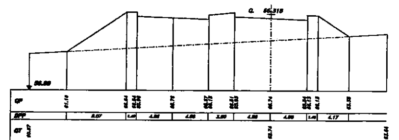
SEZIONE 847 PROGRESSIVA 58960.00
