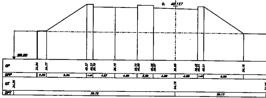
SEZIONE 574 PROGRESSIVA 41600.00
