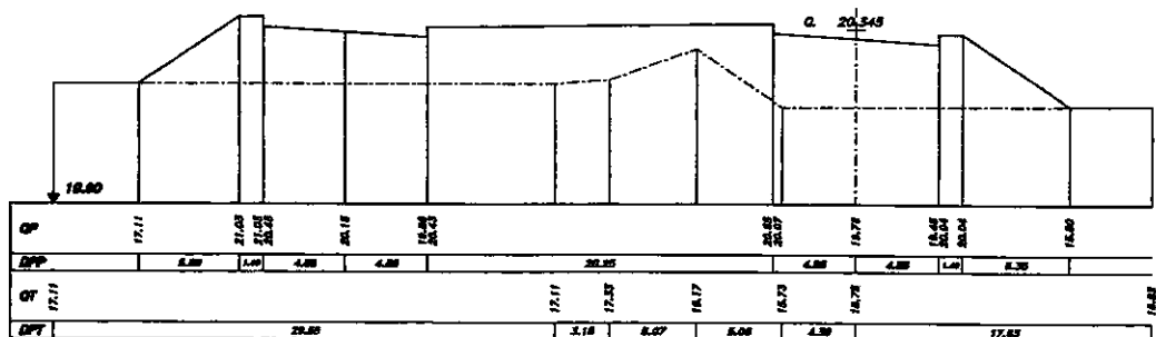
SEZIONE 187 PROGRESSIVA 13850.00
