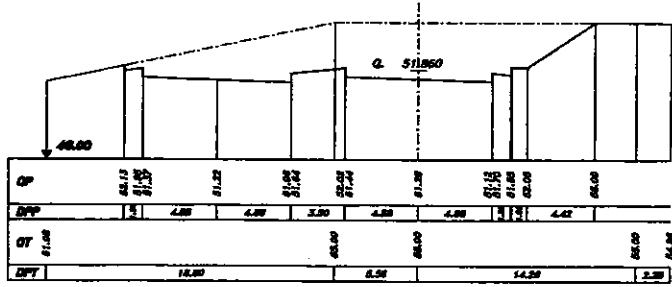
SEZIONE 792 PROGRESSIVA 54078.00
