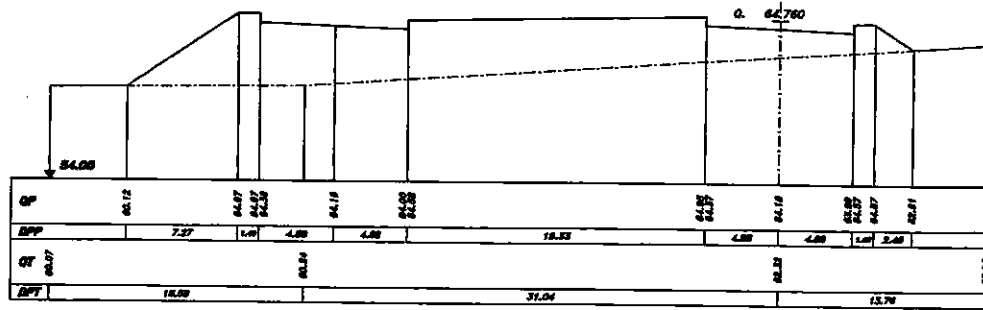
SEZIONE 985 PROGRESSIVA 85805.00
