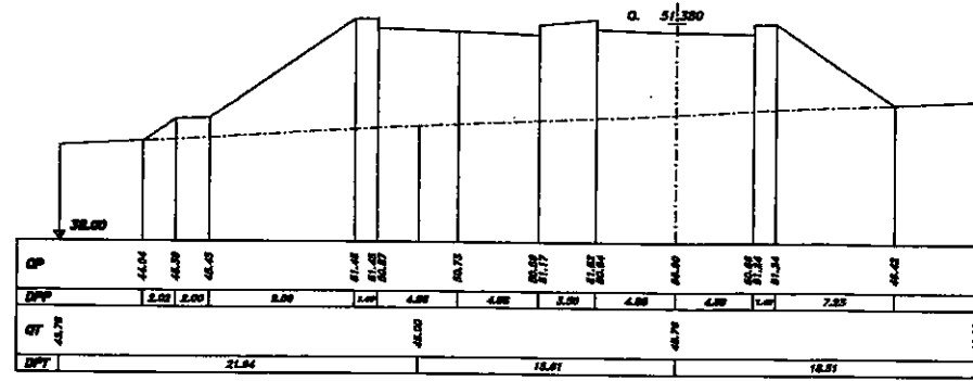
SEZIONE 789 PROGRESSIVA 53790.00
