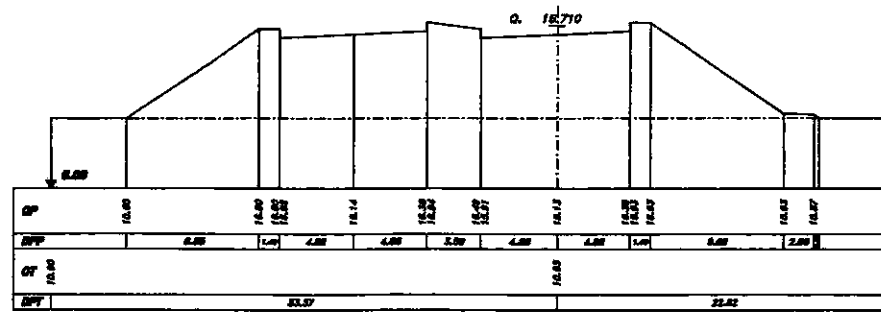
SEZIONE 268 PROGRESSIVA 23100.00
