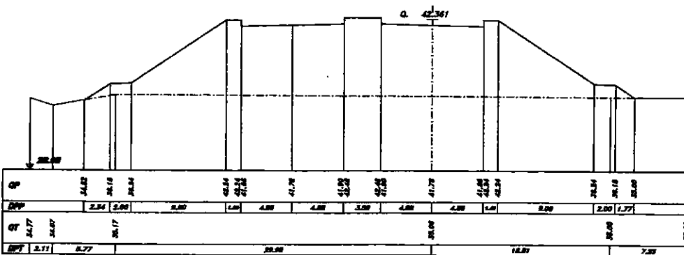
SEZIONE 78 PROGRESSIVA 6280.00
