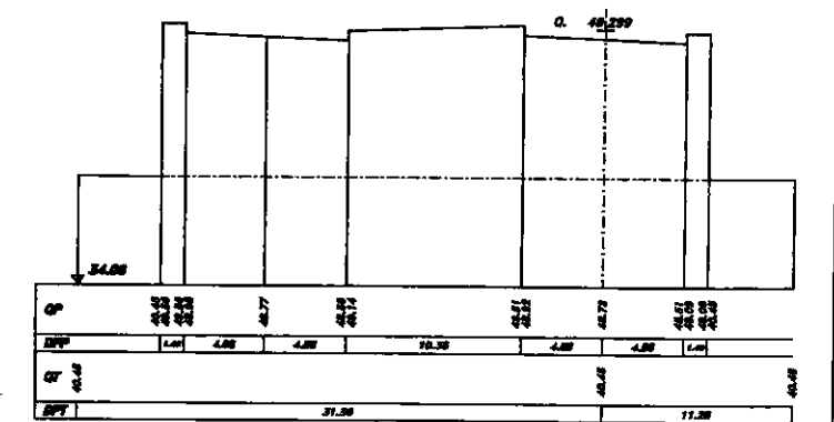
SEZIONE 77 PROGRESSIVA 6270.00
