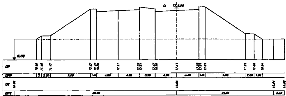
SEZIONE 264 PROGRESSIVA 22900.00
