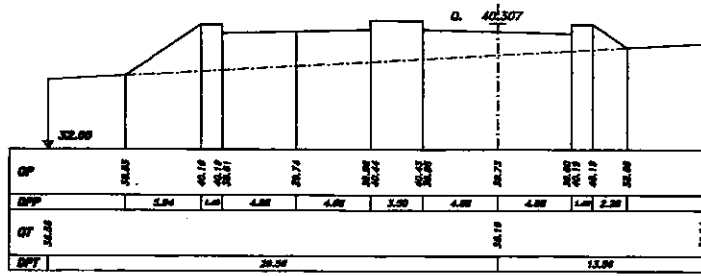
SEZIONE 69 PROGRESSIVA 5950.00
