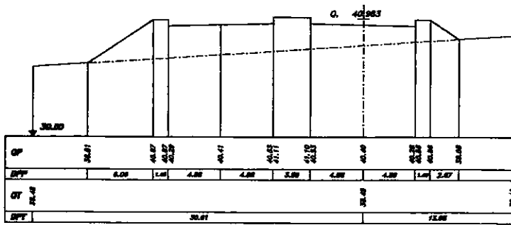
SEZIONE 72 PROGRESSIVA 5700.00
