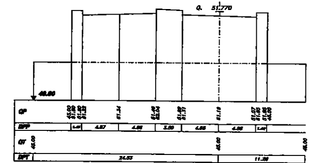
SEZIONE 791 PROGRESSIVA 54088.00
