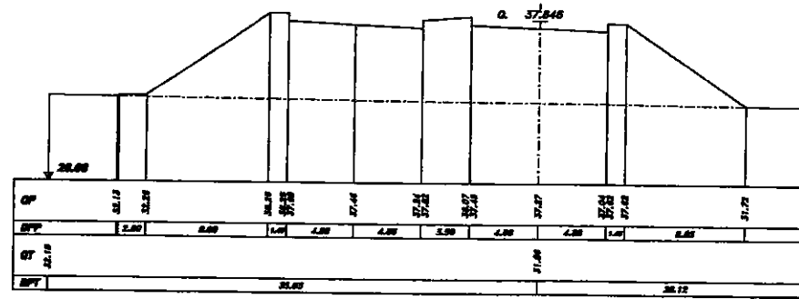
SEZIONE 578 PROGRESSIVA 41770.00
