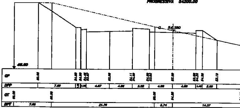
SEZIONE 795 PROGRESSIVA 54200.00
