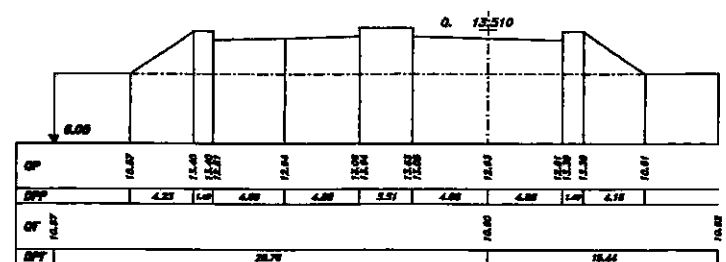
SEZIONE 277 PROGRESSIVA 23550.00
