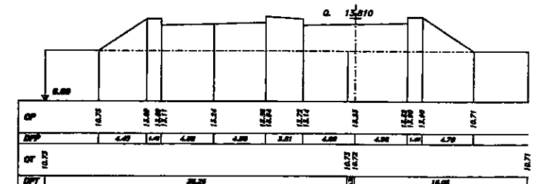
SEZIONE 275 PROGRESSIVA 23450.00
