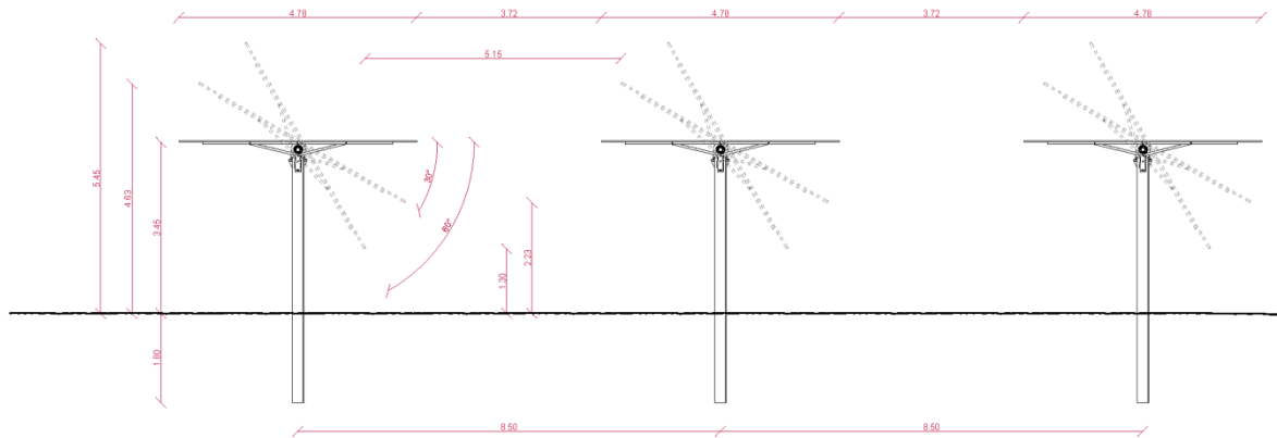
Figura 1: Prospetto trasversale Tracker Tipologia 2V (vista Est-Ovest).
