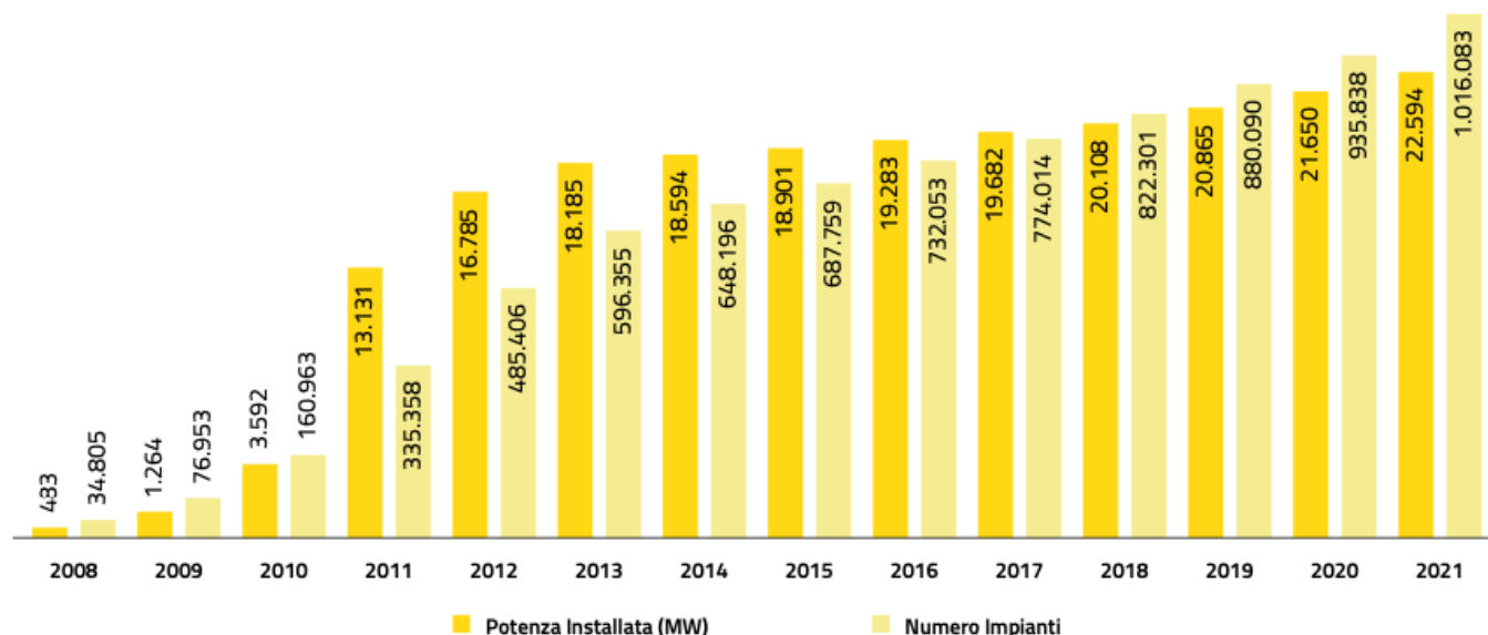
Evoluzione del numero e della potenza degli impianti fotovoltaici
