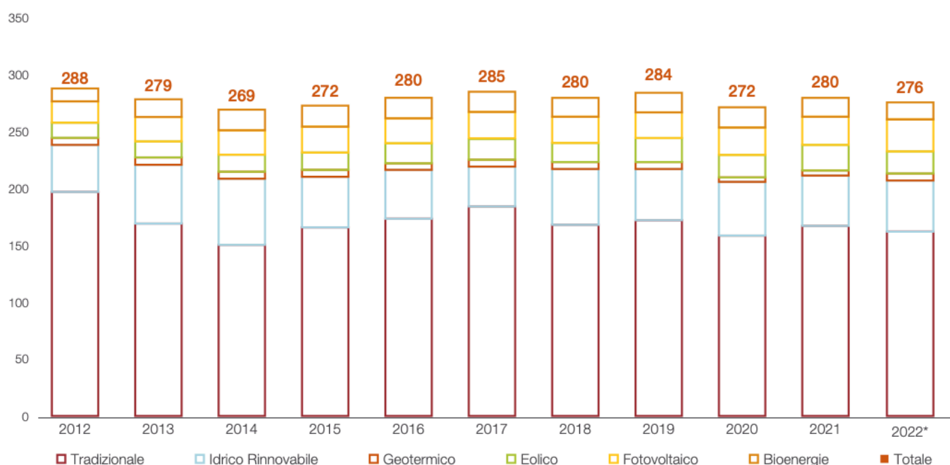
Dati TERNA: Evoluzione produzione netta nazionale per fonte (TWh)
