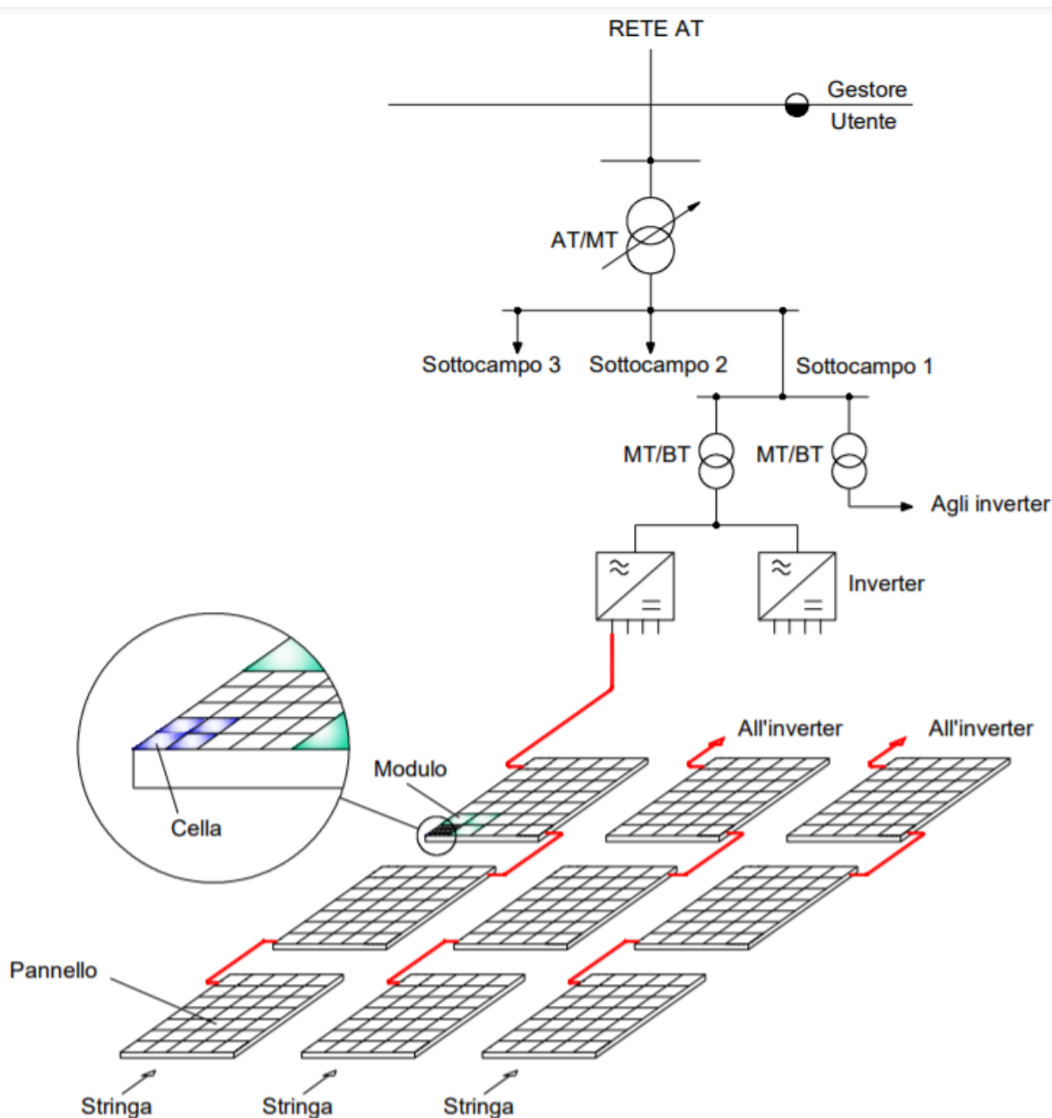
Schema sintetico della centrale di produzione solare di "TRAPANI SOLAR PARK"
