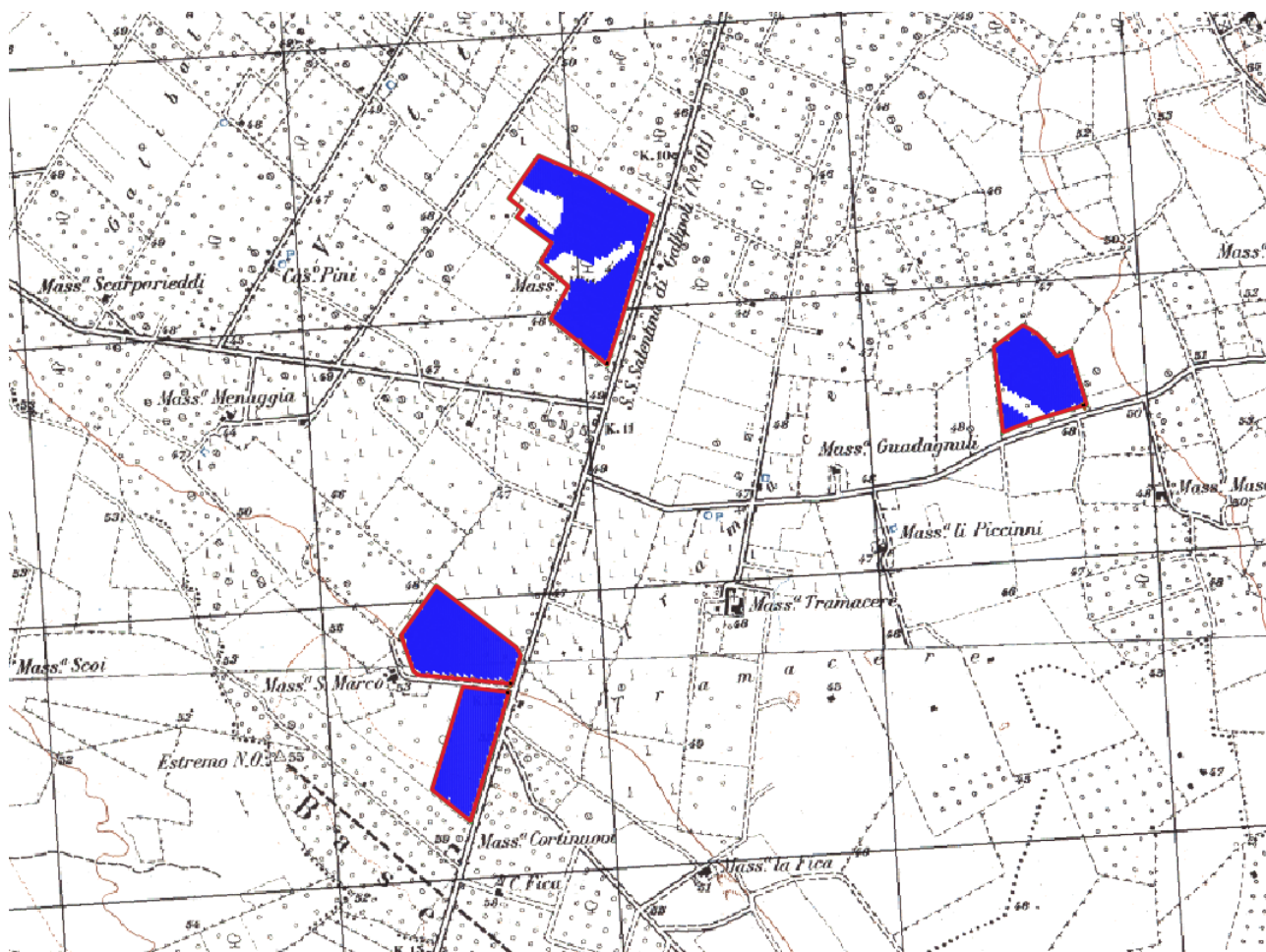
Figura 4.4. – Area di progetto con indicazione del posizionamento dei moduli fotovoltaici.
