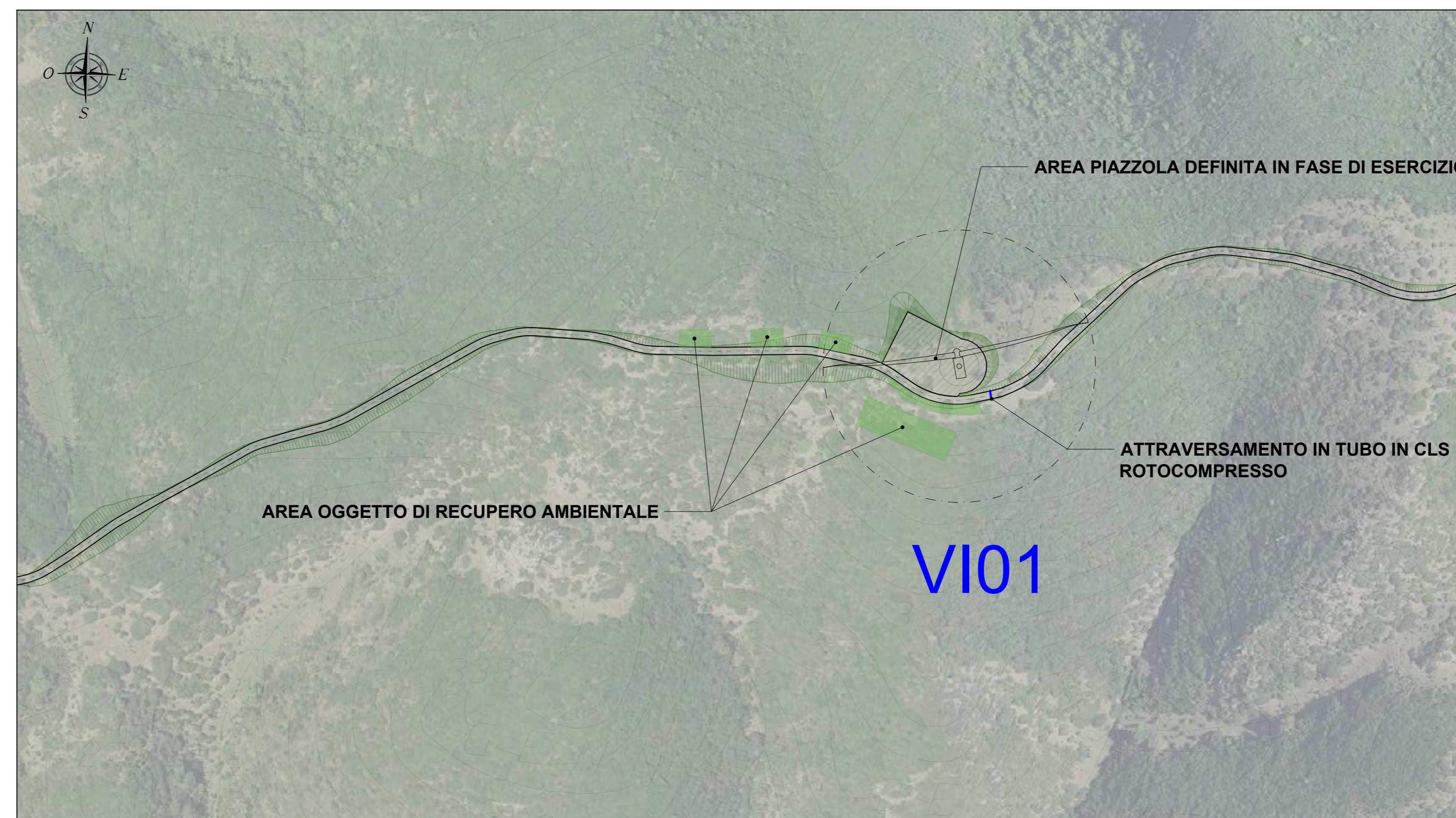
PLANIMETRIA QUADRO 4 - SCALA 1:2.000
