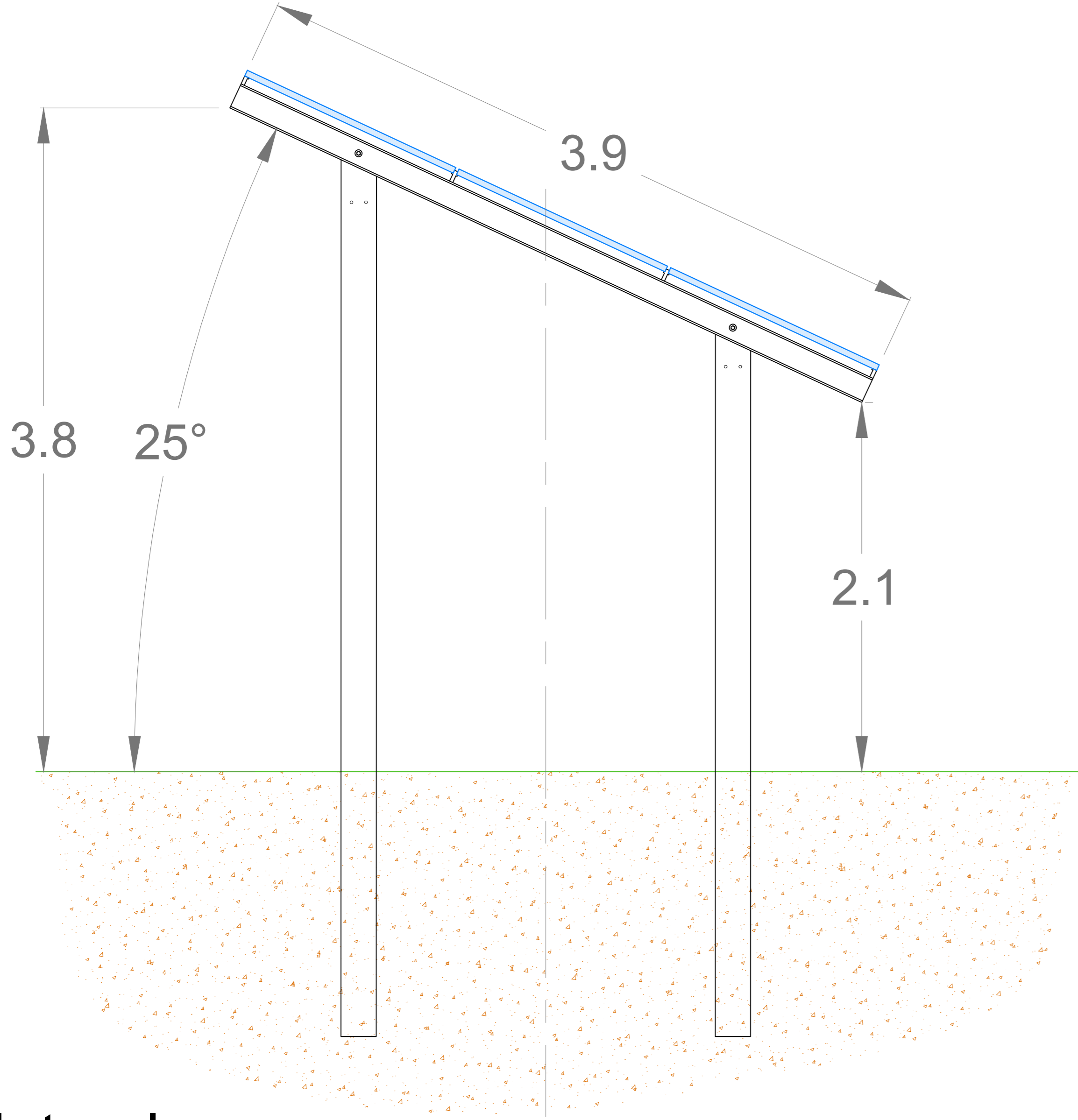
Vista laterale
