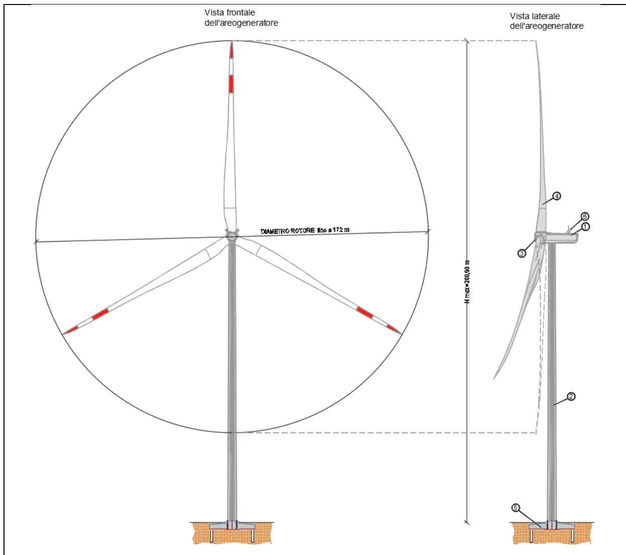
Figura 3-8 - Schema aerogeneratore H totale 200 m, diametro rotore fino a 172,0 m
