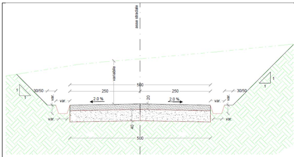
Figura 3-5 – Sezione tipo stradale in scavo
