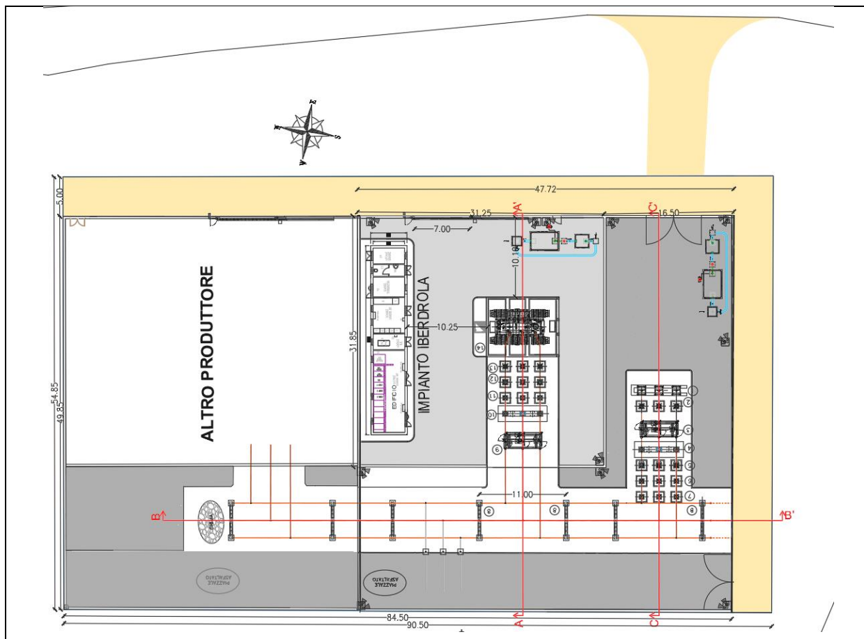
Figura 3-10 - Planimetria stazione utente ed ampliamenti futuri
