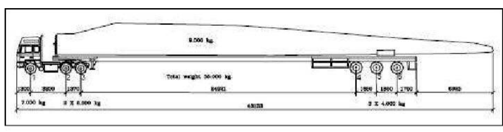
Figura 12 - Dimensioni autoarticolato
