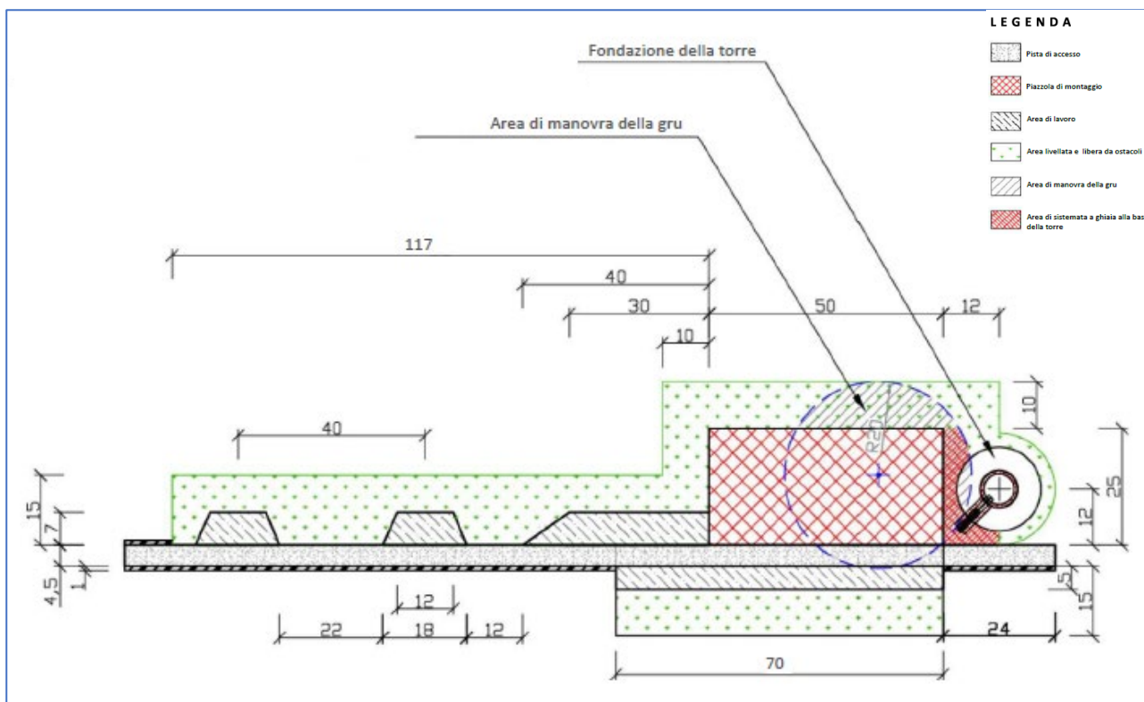
Figura 16 - tipologico della piazzola di montaggio
