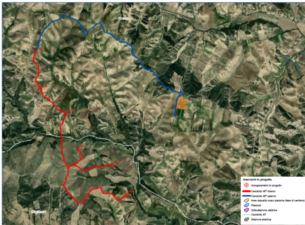
Figura 5 - layout impianto definitivo a n.6 aerogeneratori
