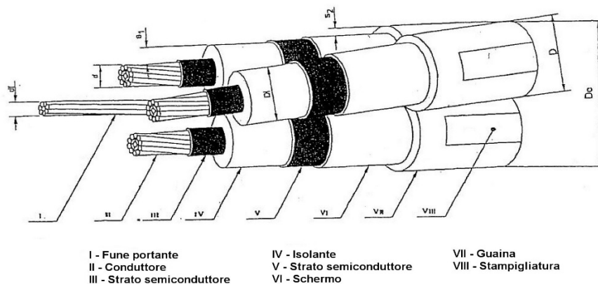
Figura 17 – Esempio di cavo
