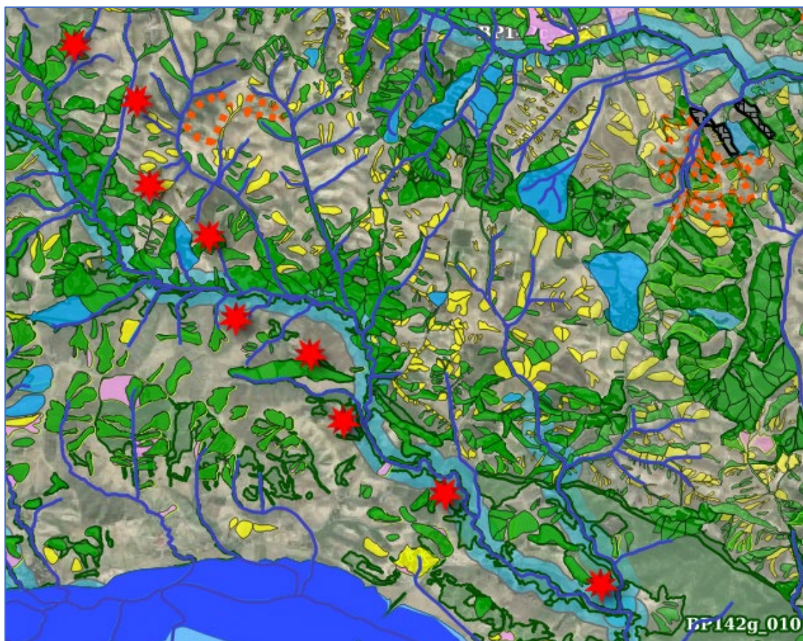
Figura 4 - Ipotesi di layout a 9 aerogeneratori - analisi vincolistica e buffer dai canali
