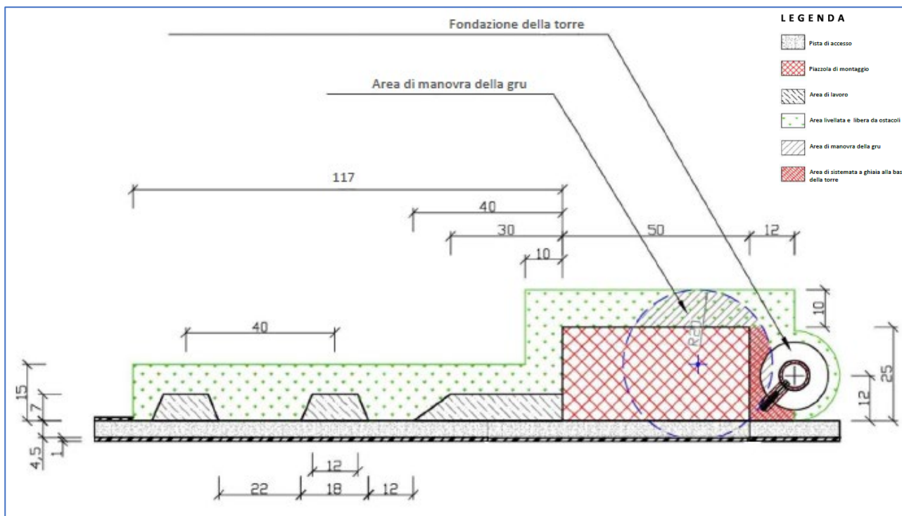
Figura 15 – tipologico della piazzola di montaggio (metodo di installazione Just in Time)
