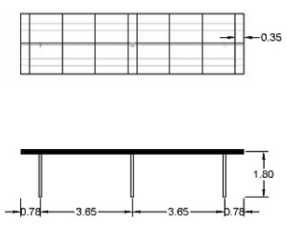
Tracker con configurazione a 6 moduli
