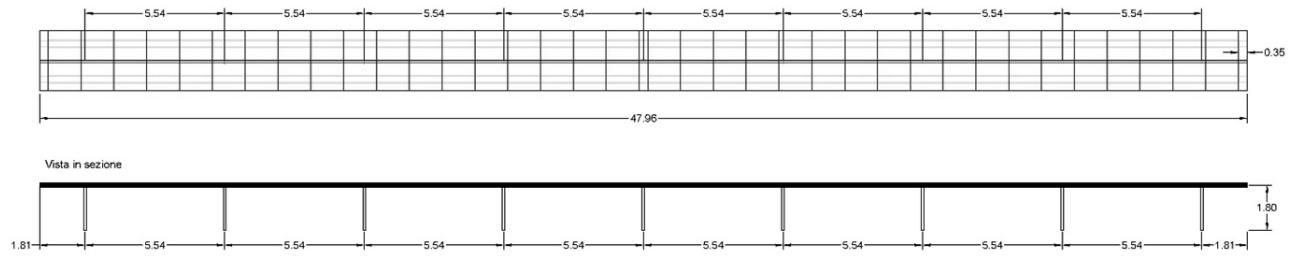
Tracker con configurazione a 24 moduli
