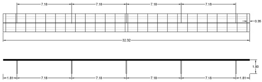
Tracker con configurazione a 12 moduli
