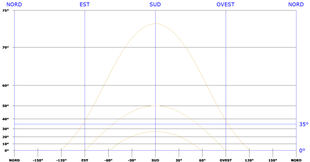
Fig. 2: Diagramma solare
