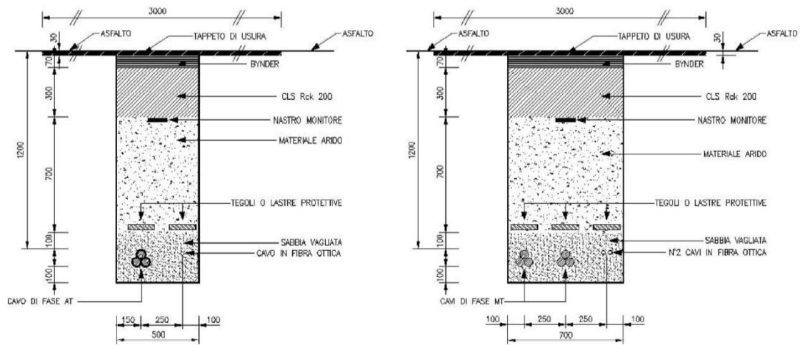
TIPICI DI POSA CAVI MT (DESTRA) E AT (SINISTRA) SU STRADE STERRATE
