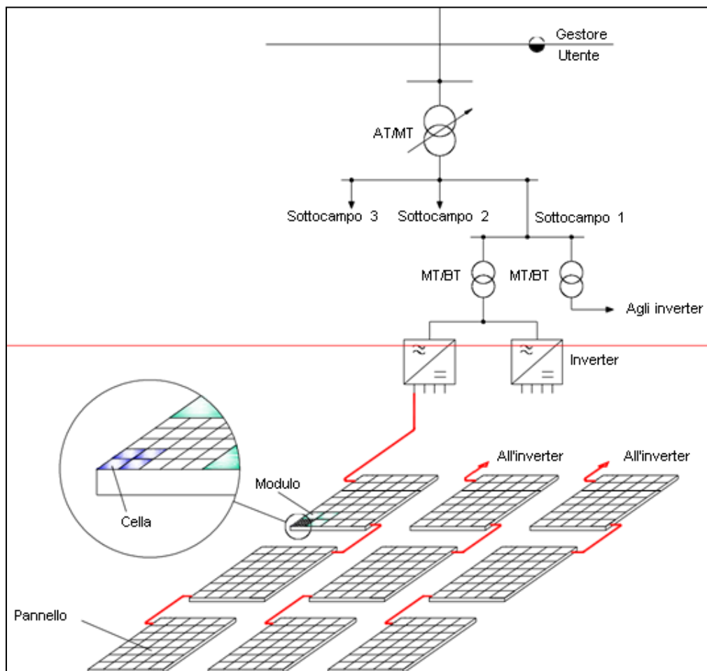
Figura 1: Schema collegamento centrale fotovoltaica
