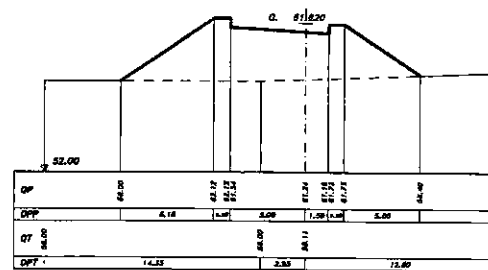
SEZIONE 37 PROGRESSIVA 455.00
