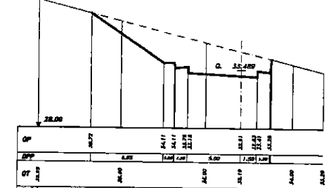
SEZIONE 44 PROGRESSIVA 190.00
