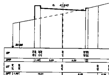
SEZIONE 15 PROGRESSIVA 380.00
