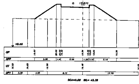
SEZIONE 76 PROGRESSIVA 210.00
