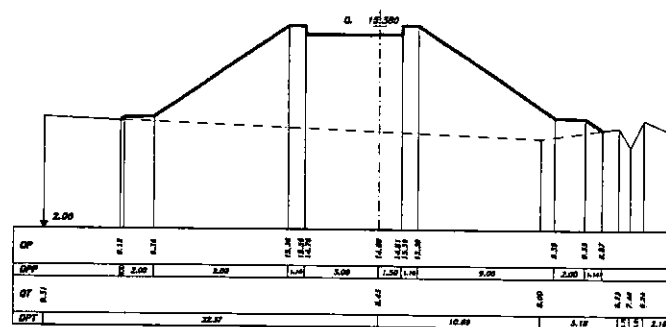
SEZIONE 85 PROGRESSIVA 400.00
