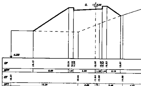
SEZIONE 92 PROGRESSIVA 160.00
