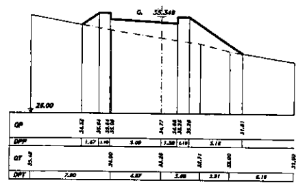
SEZIONE 41 PROGRESSIVA 100.00
