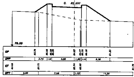
SEZIONE 22 PROGRESSIVA 170.00
