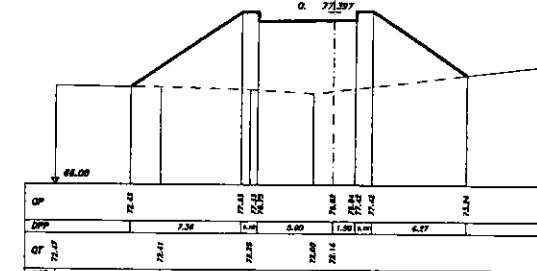
SEZIONE 15 PROGRESSIVA 290.00
