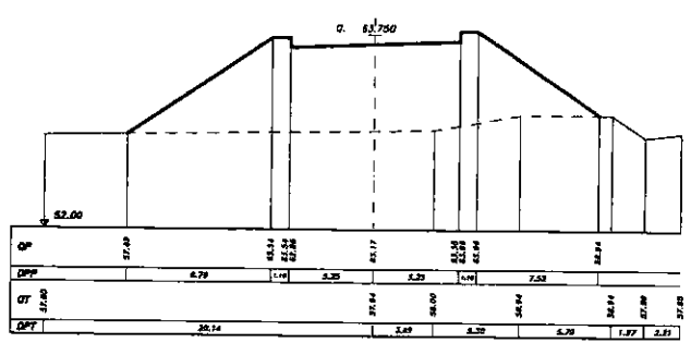
SEZIONE 8 PROGRESSIVA 370.00
