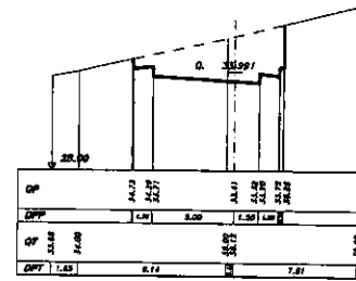
SEZIONE 53 PROGRESSIVA 90.00
