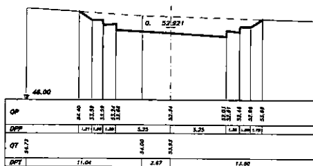
SEZIONE 6 PROGRESSIVA 250.00
