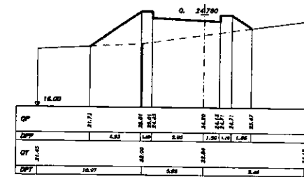
SEZIONE 21 PROGRESSIVA 355.00
