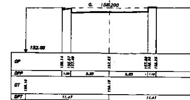
SEZIONE 8 PROGRESSIVA 350.00
