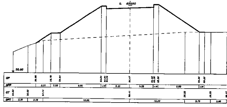
SEZIONE 7 PROGRESSIVA 344.00
