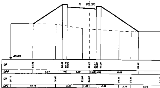
SEZIONE 58 PROGRESSIVA 245.00
