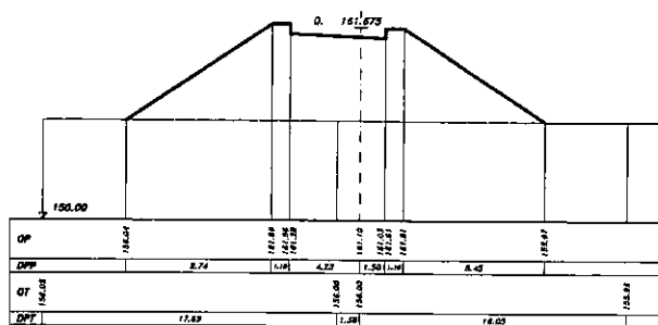
SEZIONE 55 PROGRESSIVA 205.00
