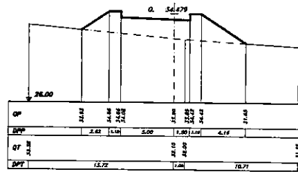
SEZIONE 1 PROGRESSIVA 240.00
