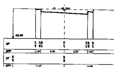
SEZIONE 3 PROGRESSIVA 118.00
