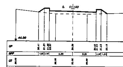
SEZIONE 5 PROGRESSIVA 218.00
