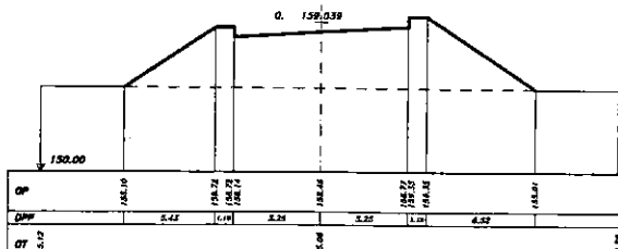
SEZIONE 16 PROGRESSIVA 725.00
