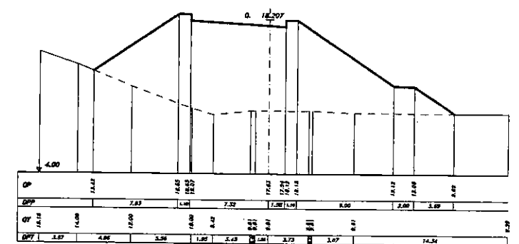
SEZIONE 32 PROGRESSIVA 1450.00
