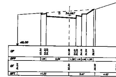
SEZIONE 18 PROGRESSIVA 240.00
