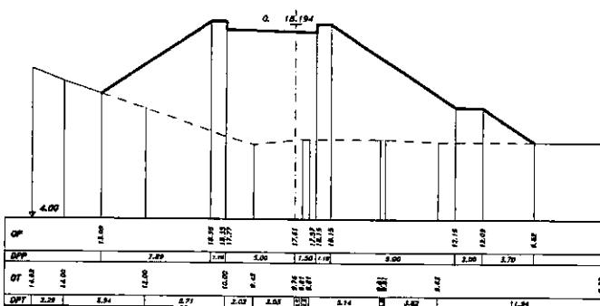
SEZIONE 94 PROGRESSIVA 485.00
