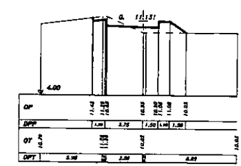
SEZIONE 38 PROGRESSIVA 1730.00
