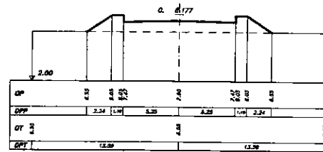
SEZIONE 3 PROGRESSIVA 105.00
