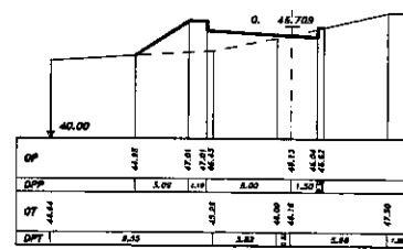
SEZIONE 25 PROGRESSIVA 325.00
