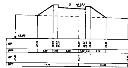
SEZIONE 32 PROGRESSIVA 170.00
