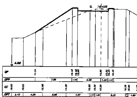
SEZIONE 87 PROGRESSIVA 480.00
