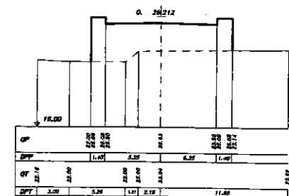
SEZIONE 4 PROGRESSIVA 60.00
