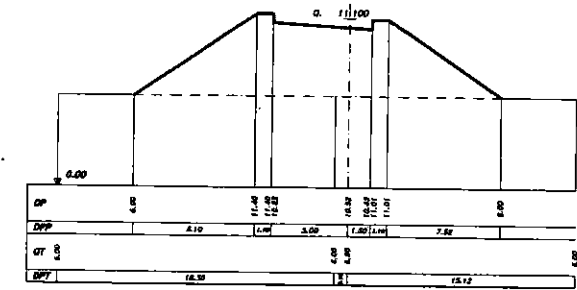
SEZIONE 33 PROGRESSIVA 400.00
