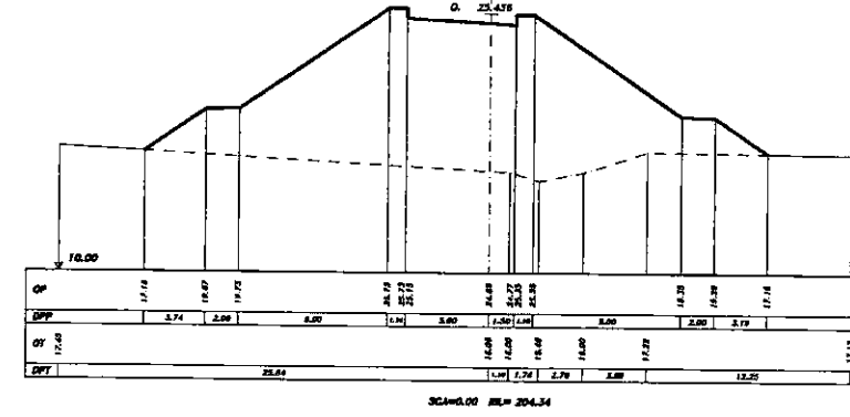
SEZIONE 63 PROGRESSIVA 380.00
