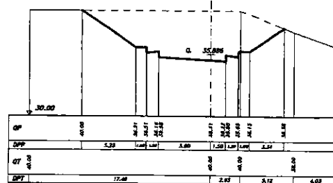
SEZIONE 32 PROGRESSIVA 230.00
