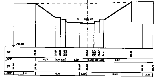
SEZIONE 25 PROGRESSIVA 290.00
