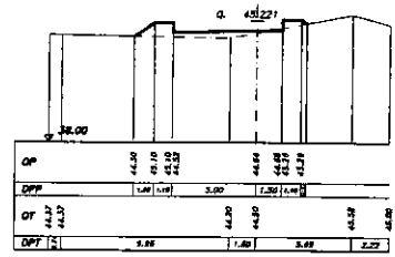
SEZIONE 29 PROGRESSIVA 50.00
