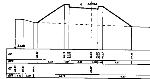
SEZIONE 38 PROGRESSIVA 495.00
