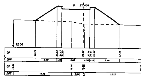
SEZIONE 12 PROGRESSIVA 225.00
