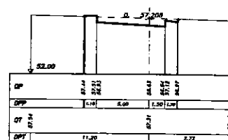
SEZIONE 53 PROGRESSIVA 80.00
