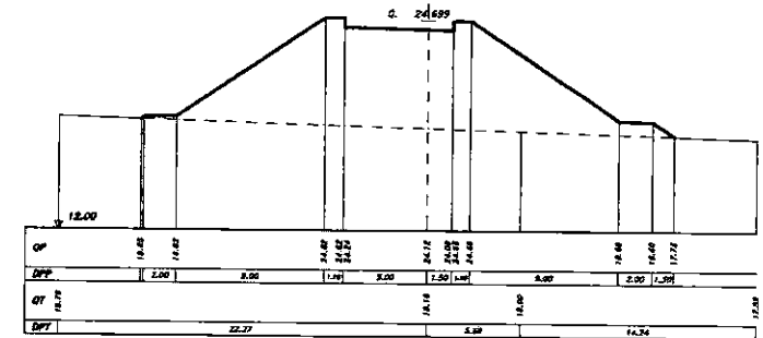
SEZIONE 19 PROGRESSIVA 112.00
