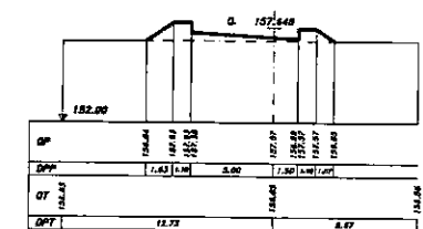
SEZIONE 46 PROGRESSIVA 360.00
