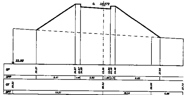
SEZIONE 61 PROGRESSIVA 180.00
