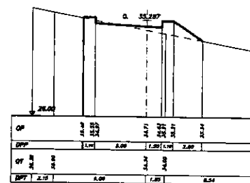
SEZIONE 42 PROGRESSIVA 130.00
