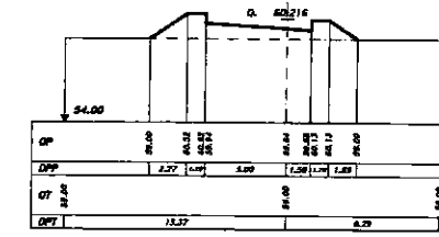
SEZIONE 39 PROGRESSIVA 535.00
