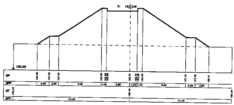
SEZIONE 32 PROGRESSIVA 40.00
