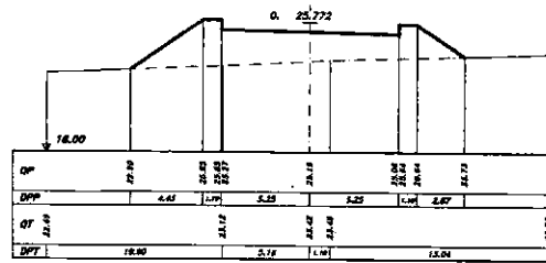
SEZIONE 6 PROGRESSIVA 165.00
