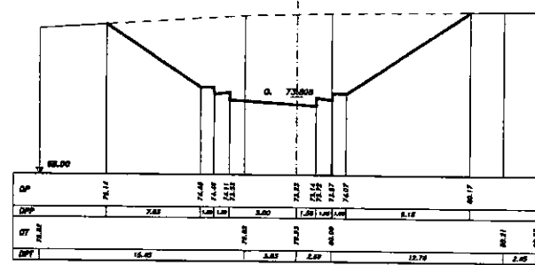
SEZIONE 26 PROGRESSIVA 320.00
