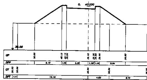
SEZIONE 10 PROGRESSIVA 345.00
