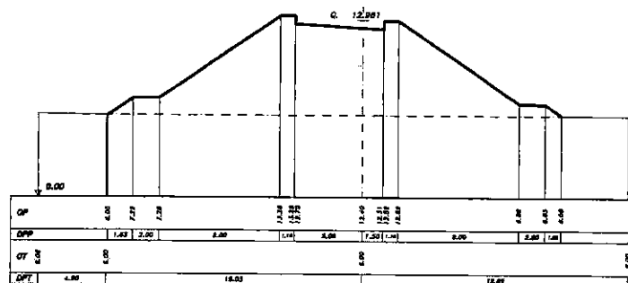
SEZIONE 26 PROGRESSIVA 325.00
