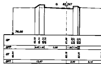
SEZIONE 23 PROGRESSIVA 210.00
