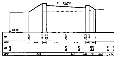
SEZIONE 5 PROGRESSIVA 160.00
