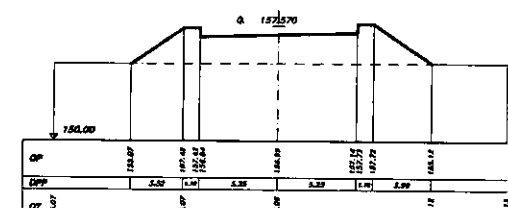
SEZIONE 15 PROGRESSIVA 690.00
