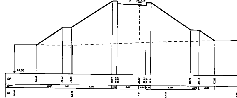
SEZIONE 17 PROGRESSIVA 255.00
