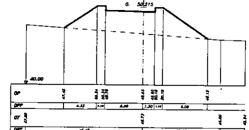
SEZIONE 15 PROGRESSIVA 170.00
