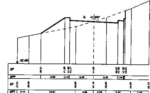
SEZIONE 13 PROGRESSIVA 330.00
