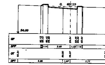
SEZIONE 34 PROGRESSIVA 335.00
