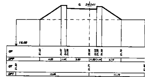
SEZIONE 12 PROGRESSIVA 290.00
