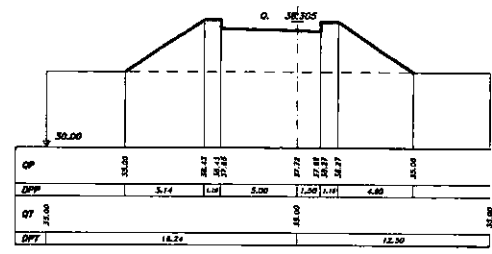
SEZIONE 1 PROGRESSIVA 7.00
