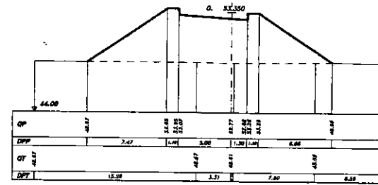
SEZIONE 22 PROGRESSIVA 200.00
