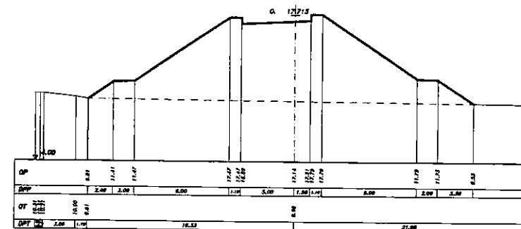
SEZIONE 95 PROGRESSIVA 530.00
