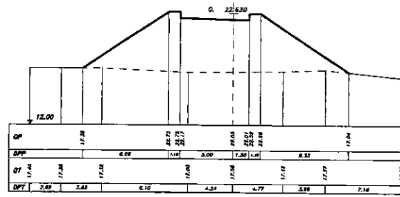
SEZIONE 11 PROGRESSIVA 198.00
