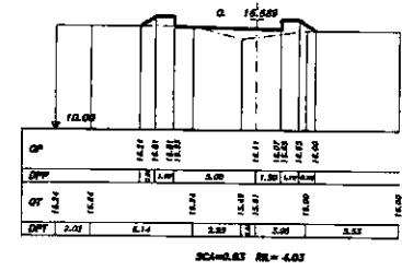
SEZIONE 77 PROGRESSIVA 220.41
