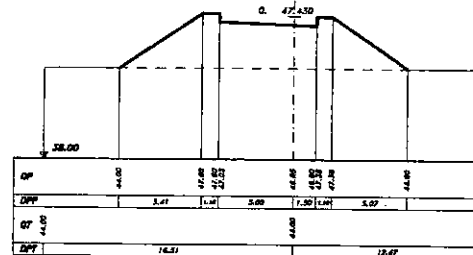
SEZIONE 14 PROGRESSIVA 130.00
