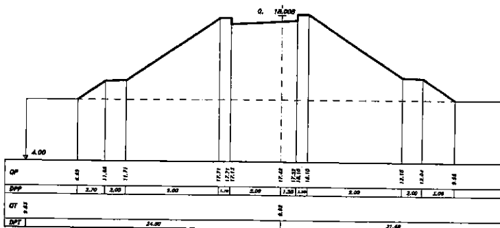
SEZIONE 96 PROGRESSIVA 550.00
