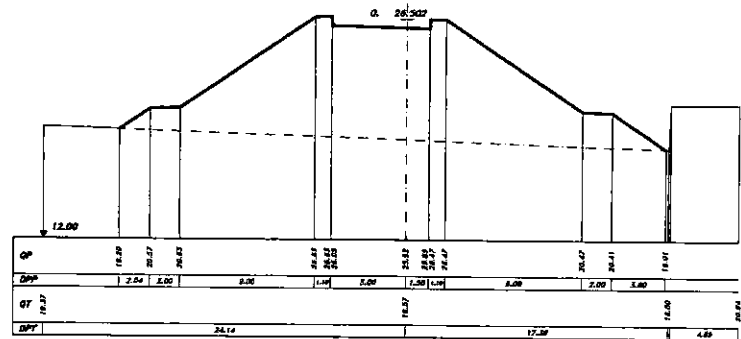
SEZIONE 20 PROGRESSIVA 147.00
