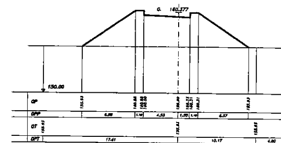
SEZIONE 54 PROGRESSIVA 170.00
