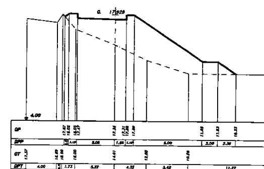
SEZIONE 83 PROGRESSIVA 115.00
