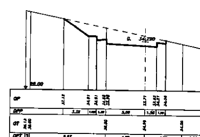
SEZIONE 43 PROGRESSIVA 160.00
