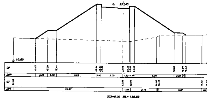
SEZIONE 61 PROGRESSIVA 310.00
