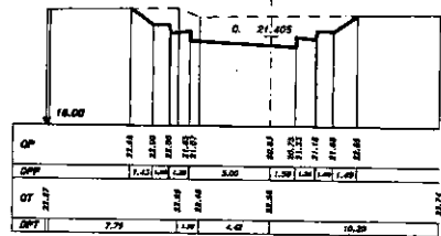
SEZIONE 24 PROGRESSIVA 465.00
