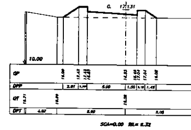
SEZIONE 74 PROGRESSIVA 108.00
