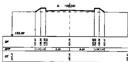
SEZIONE 12 PROGRESSIVA 550.00
