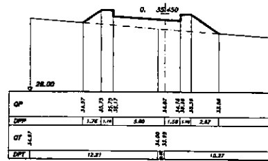
SEZIONE 31 PROGRESSIVA 190.00
