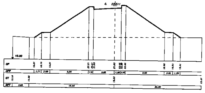
SEZIONE 39 PROGRESSIVA 357.00
