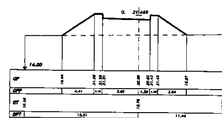
SEZIONE 9 PROGRESSIVA 112.00
