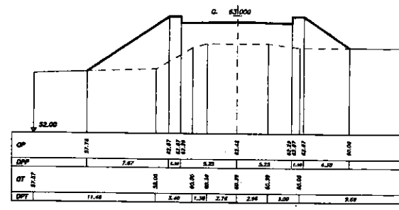
SEZIONE 3 PROGRESSIVA 125.00
