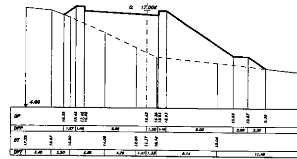
SEZIONE 28 PROGRESSIVA 1235.00
