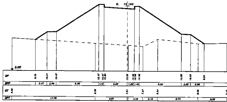
SEZIONE 27 PROGRESSIVA 1180.00
