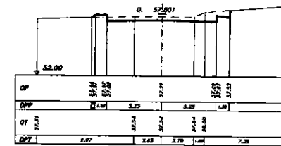
SEZIONE 11 PROGRESSIVA 520.00
