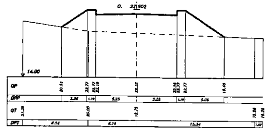
SEZIONE 1 PROGRESSIVA 65.00
