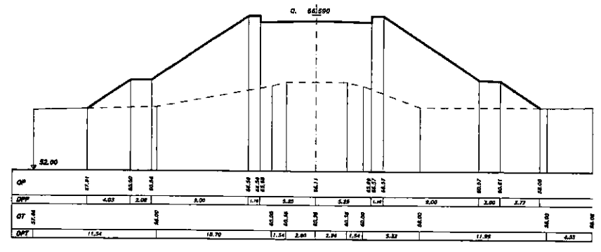
SEZIONE 5 PROGRESSIVA 202.00
