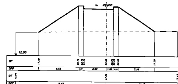
SEZIONE 10 PROGRESSIVA 147.00
