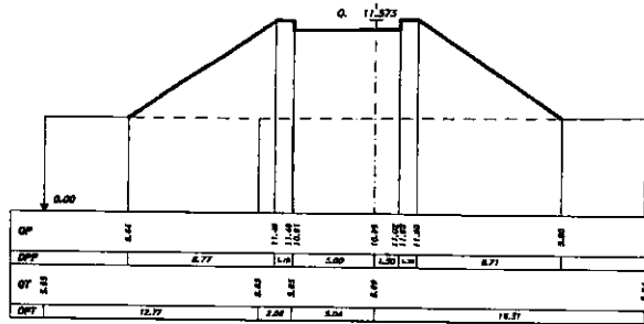
SEZIONE 12 PROGRESSIVA 35.00
