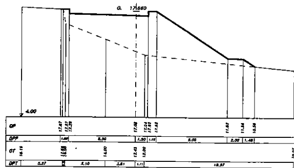
SEZIONE 30 PROGRESSIVA 1310.00
