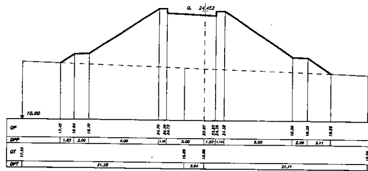
SEZIONE 35 PROGRESSIVA 210.00
