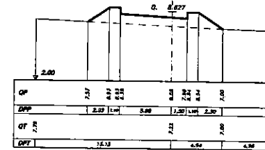
SEZIONE 32 PROGRESSIVA 375.00
