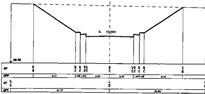
SEZIONE 6 PROGRESSIVA 265.00
