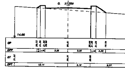
SEZIONE 3 PROGRESSIVA 175.00
