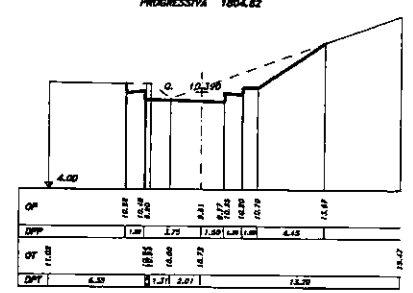
SEZIONE 39 PROGRESSIVA 1804.82
