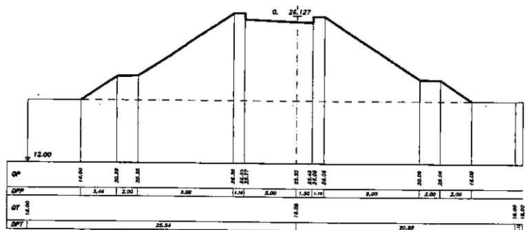
SEZIONE 16 PROGRESSIVA 225.00
