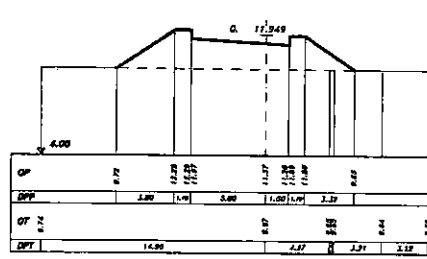
SEZIONE 37 PROGRESSIVA 1680.00
