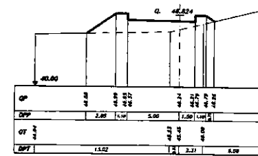
SEZIONE 26 PROGRESSIVA 365.00
