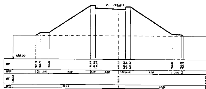
SEZIONE 41 PROGRESSIVA 180.00
