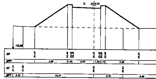
SEZIONE 11 PROGRESSIVA 255.00
