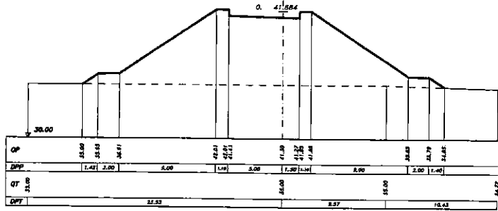
SEZIONE 8 PROGRESSIVA 285.00
