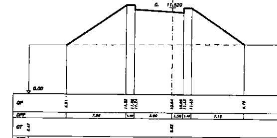
SEZIONE 24 PROGRESSIVA 235.00
