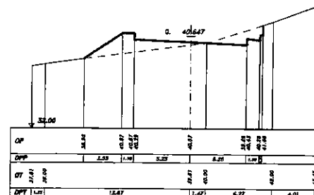
SEZIONE 15 PROGRESSIVA 380.00
