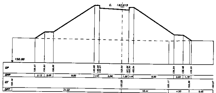
SEZIONE 34 PROGRESSIVA 120.00
