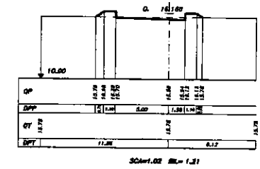
SEZIONE 77 PROGRESSIVA 220.41
