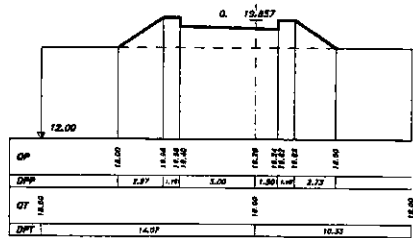
SEZIONE 17 PROGRESSIVA 42.00
