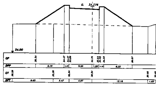
SEZIONE 18 PROGRESSIVA 235.00
