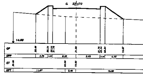
SEZIONE 2 PROGRESSIVA 130.00
