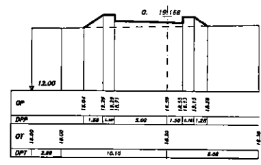
SEZIONE 6 PROGRESSIVA 7.00
