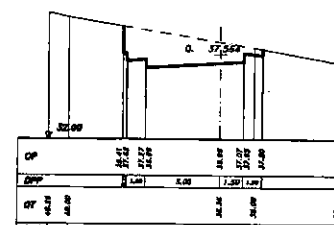
SEZIONE 63 PROGRESSIVA 264.00
