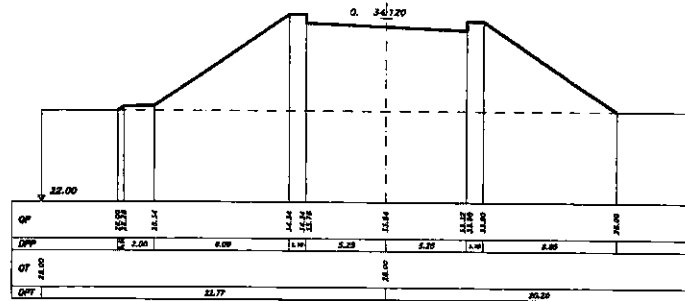
SEZIONE 11 PROGRESSIVA 290.00
