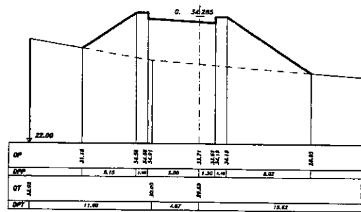
SEZIONE 40 PROGRESSIVA 70.00
