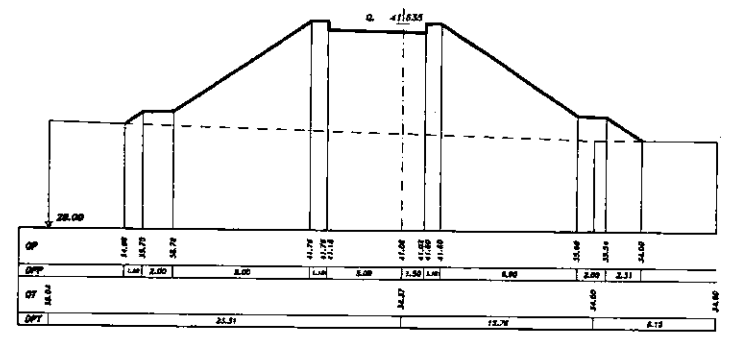
SEZIONE 3 PROGRESSIVA 77.00
