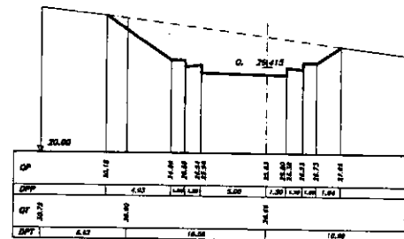
SEZIONE 4 PROGRESSIVA 360.00
