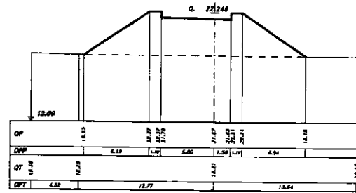
SEZIONE 18 PROGRESSIVA 77.00
