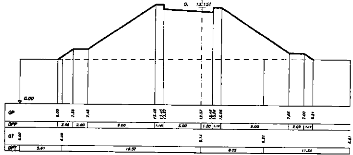
SEZIONE 30 PROGRESSIVA 310.00
