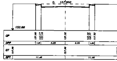
SEZIONE 6 PROGRESSIVA 250.00
