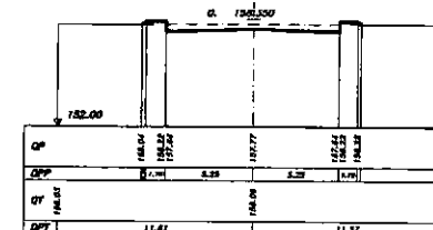
SEZIONE 9 PROGRESSIVA 400.00
