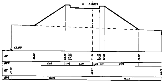
SEZIONE 33 PROGRESSIVA 215.00
