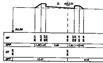
SEZIONE 33 PROGRESSIVA 295.00
