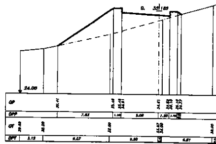
SEZIONE 52 PROGRESSIVA 60.00
