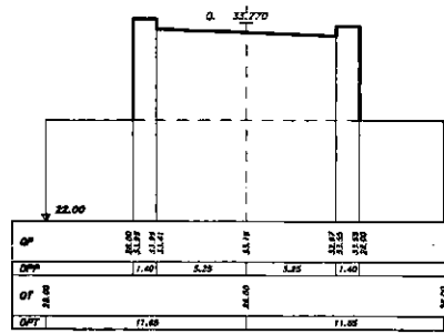
SEZIONE 5 PROGRESSIVA 160.00
