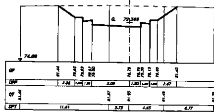
SEZIONE 26 PROGRESSIVA 320.00
