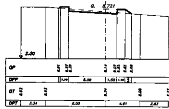
SEZIONE 20 PROGRESSIVA 110.00
