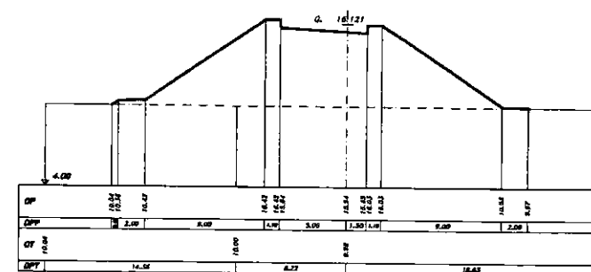
SEZIONE 34 PROGRESSIVA 1530.00
