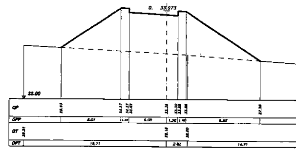
SEZIONE 60 PROGRESSIVA 180.00
