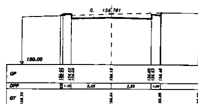
SEZIONE 12 PROGRESSIVA 550.00
