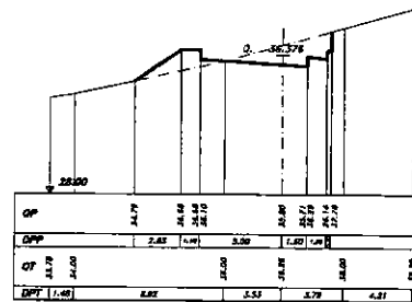
SEZIONE 51 PROGRESSIVA 30.00
