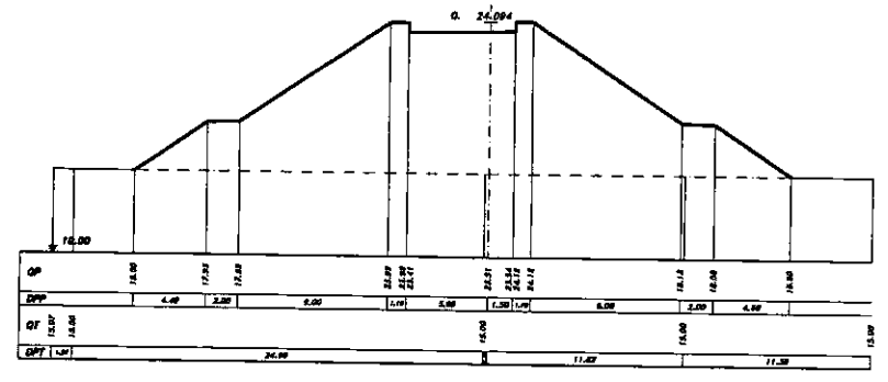
SEZIONE 38 PROGRESSIVA 325.00
