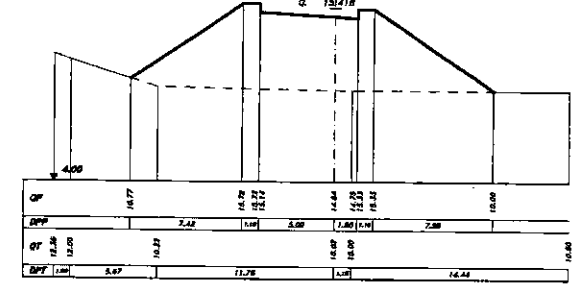
SEZIONE 26 PROGRESSIVA 1150.00
