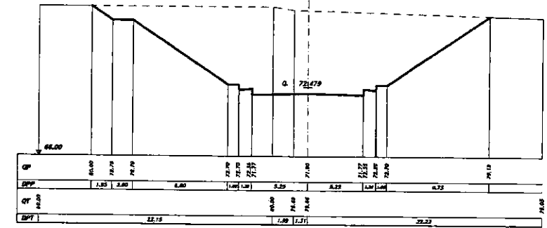
SEZIONE 3 PROGRESSIVA 115.00
