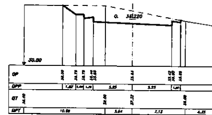
SEZIONE 12 PROGRESSIVA 300.00
