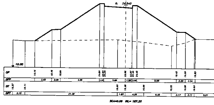
SEZIONE 62 PROGRESSIVA 345.00
