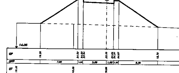
SEZIONE 15 PROGRESSIVA 180.00
