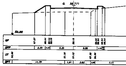
SEZIONE 10 PROGRESSIVA 470.00
