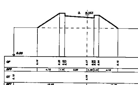
SEZIONE 23 PROGRESSIVA 205.00
