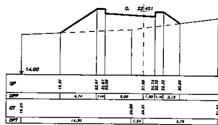
SEZIONE 22 PROGRESSIVA 395.00
