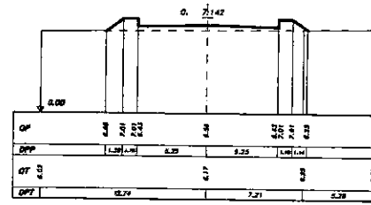
SEZIONE 4 PROGRESSIVA 135.00
