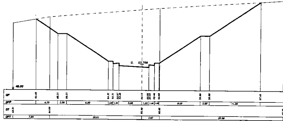
SEZIONE 16 PROGRESSIVA 170.00
