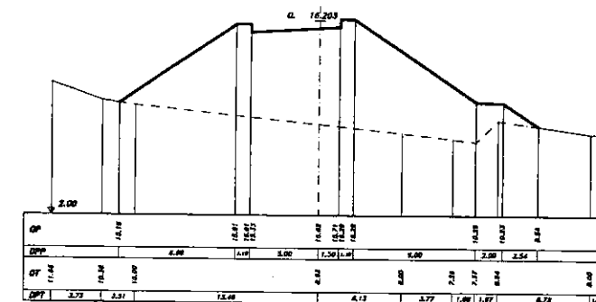
SEZIONE 93 PROGRESSIVA 215.00
