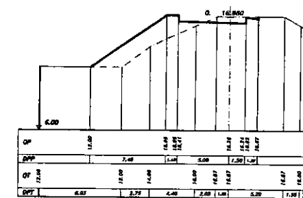
SEZIONE 88 PROGRESSIVA 520.83
