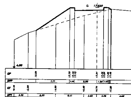
SEZIONE 82 PROGRESSIVA 80.00
