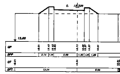
SEZIONE 7 PROGRESSIVA 42.00
