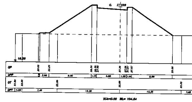
SEZIONE 49 PROGRESSIVA 305.00
