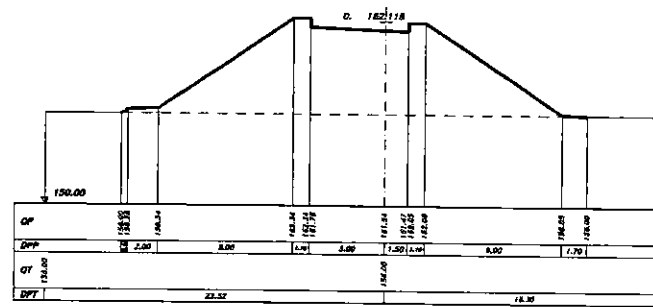
SEZIONE 42 PROGRESSIVA 220.00
