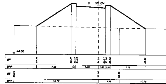
SEZIONE 21 PROGRESSIVA 150.00
