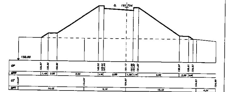
SEZIONE 35 PROGRESSIVA 160.00
