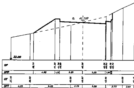
SEZIONE 14 PROGRESSIVA 360.00
