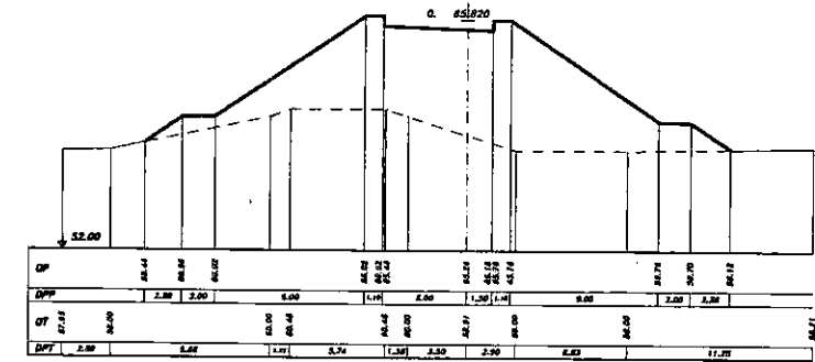
SEZIONE 39 PROGRESSIVA 535.00
