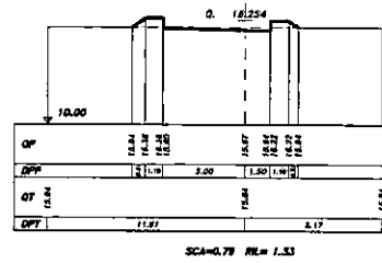
SEZIONE 76 PROGRESSIVA 210.00
