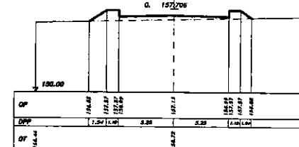
SEZIONE 14 PROGRESSIVA 640.00
