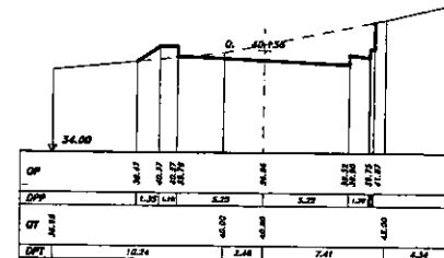
SEZIONE 16 PROGRESSIVA 420.00
