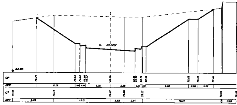
SEZIONE 1 PROGRESSIVA 25.00
