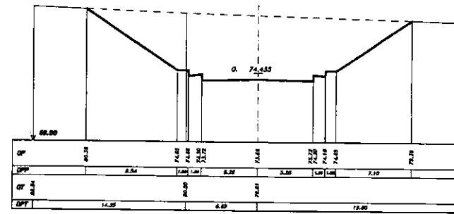
SEZIONE 5 PROGRESSIVA 215.00
