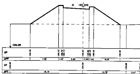
SEZIONE 44 PROGRESSIVA 290.00
