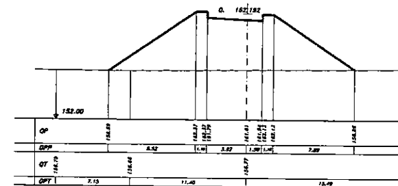
SEZIONE 56 PROGRESSIVA 240.00
