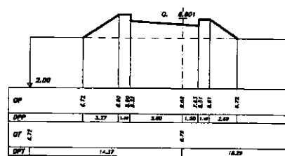
SEZIONE 25 PROGRESSIVA 290.00
