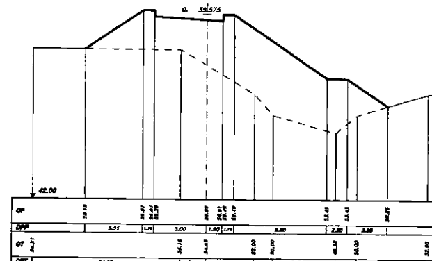
SEZIONE 57 PROGRESSIVA 220.00
