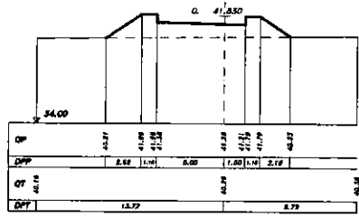
SEZIONE 12 PROGRESSIVA 30.00
