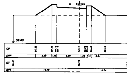
SEZIONE 36 PROGRESSIVA 415.00
