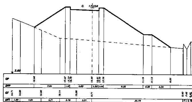
SEZIONE 84 PROGRESSIVA 350.00
