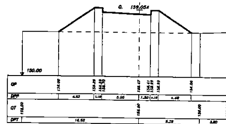
SEZIONE 45 PROGRESSIVA 325.00
