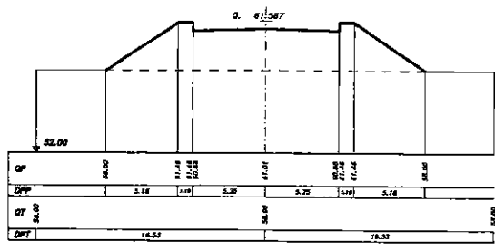
SEZIONE 1 PROGRESSIVA 83.00
