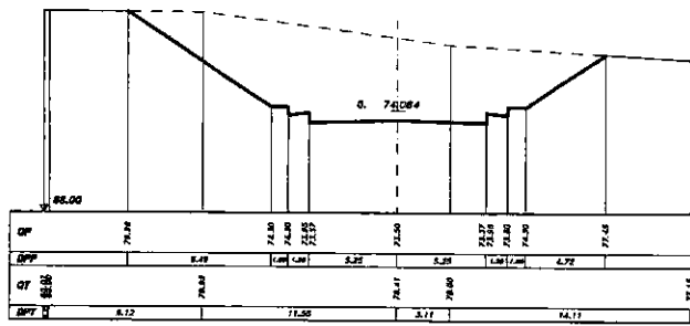
SEZIONE 4 PROGRESSIVA 165.00
