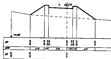
SEZIONE 14 PROGRESSIVA 135.00
