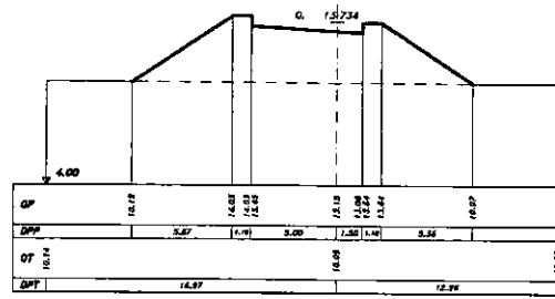
SEZIONE 24 PROGRESSIVA 1060.00
