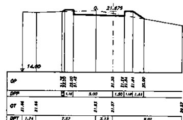
SEZIONE 12 PROGRESSIVA 45.00
