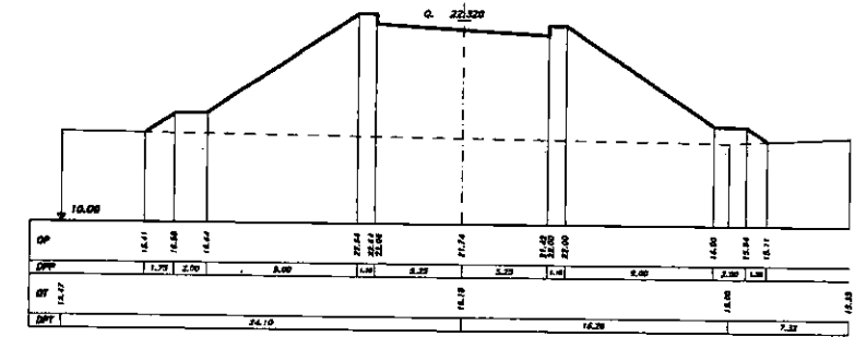
SEZIONE 7 PROGRESSIVA 335.50
