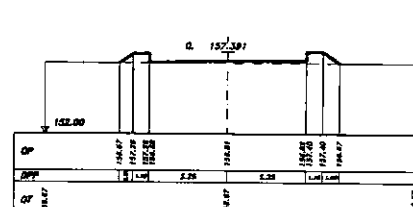
SEZIONE 10 PROGRESSIVA 450.00
