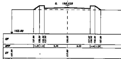
SEZIONE 11 PROGRESSIVA 500.00
