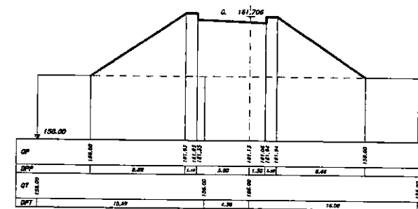
SEZIONE 43 PROGRESSIVA 260.00
