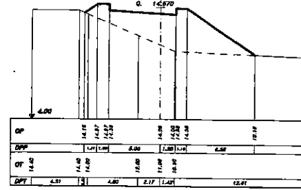
SEZIONE 25 PROGRESSIVA 1110.00
