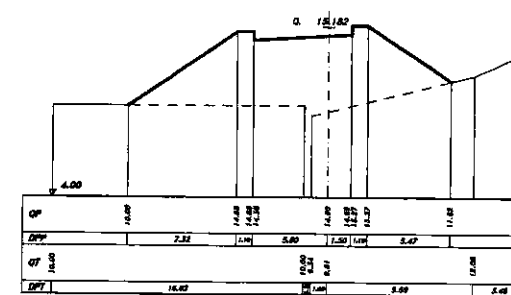
SEZIONE 86 PROGRESSIVA 430.00
