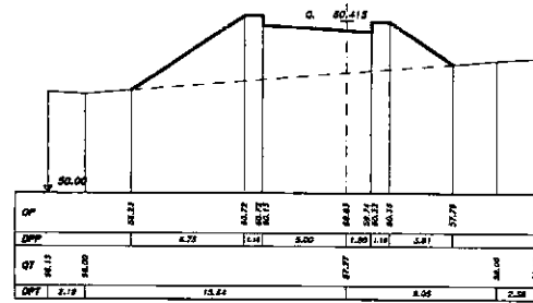
SEZIONE 36 PROGRESSIVA 415.00
