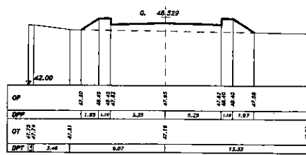
SEZIONE 1 PROGRESSIVA 65.00
