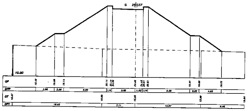
SEZIONE 37 PROGRESSIVA 290.00
