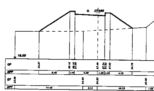
SEZIONE 20 PROGRESSIVA 315.00
