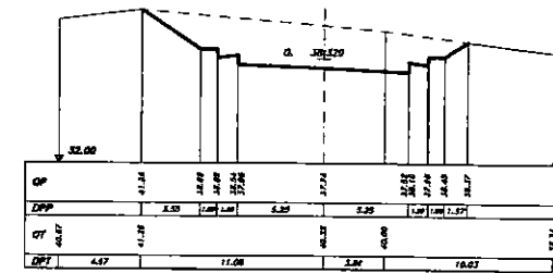
SEZIONE 13 PROGRESSIVA 330.00
