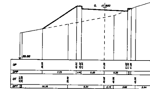
SEZIONE 12 PROGRESSIVA 300.00
