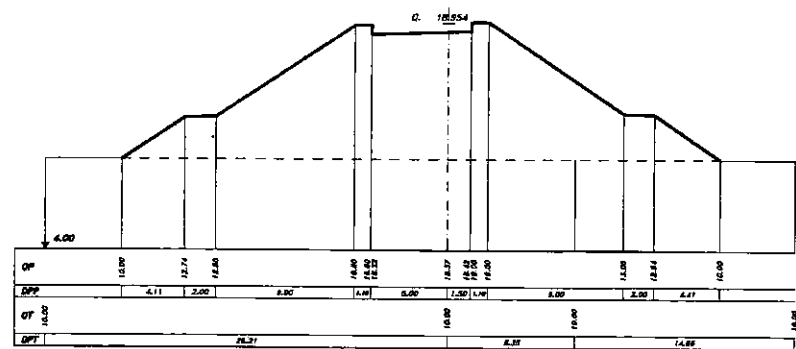
SEZIONE 81 PROGRESSIVA 41.00
