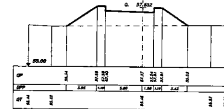
SEZIONE 55 PROGRESSIVA 150.00
