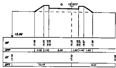
SEZIONE 16 PROGRESSIVA 7.00
