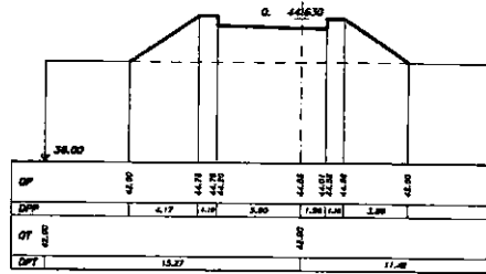
SEZIONE 16 PROGRESSIVA 210.00
