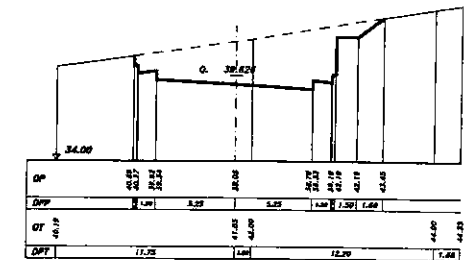
SEZIONE 17 PROGRESSIVA 450.00
