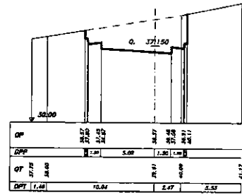
SEZIONE 50 PROGRESSIVA 0.00
