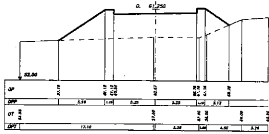
SEZIONE 9 PROGRESSIVA 420.00
