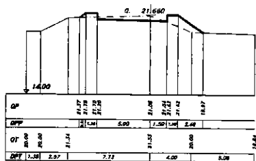
SEZIONE 11 PROGRESSIVA 0.00
