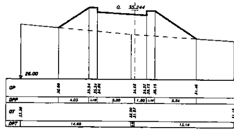
SEZIONE 30 PROGRESSIVA 182.00
