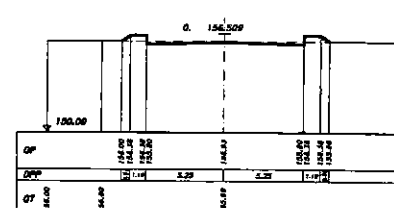
SEZIONE 13 PROGRESSIVA 590.00
