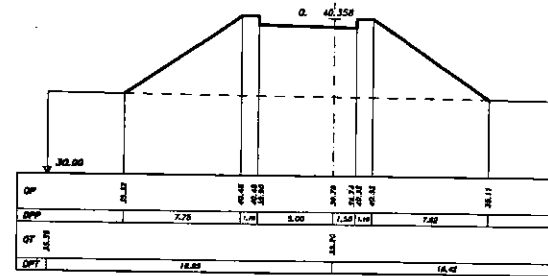
SEZIONE 9 PROGRESSIVA 320.00
