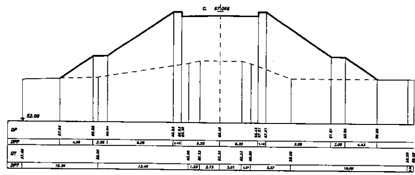
SEZIONE 6 PROGRESSIVA 214.00
