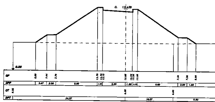
SEZIONE 15 PROGRESSIVA 140.00
