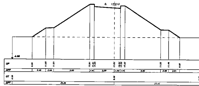
SEZIONE 33 PROGRESSIVA 1480.00
