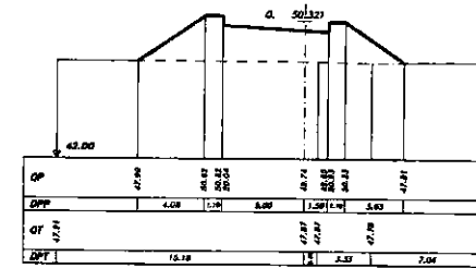
SEZIONE 23 PROGRESSIVA 240.00
