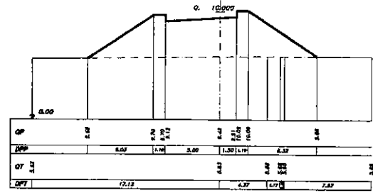
SEZIONE 11 PROGRESSIVA 0.00
