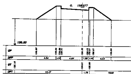
SEZIONE 53 PROGRESSIVA 135.00
