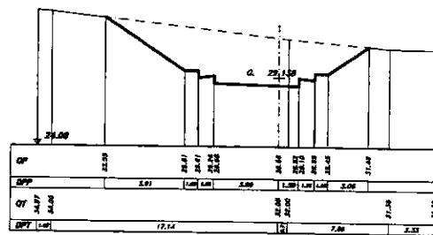
SEZIONE 3 PROGRESSIVA 320.00
