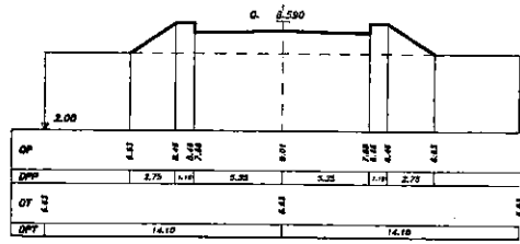
SEZIONE 2 PROGRESSIVA 85.00
