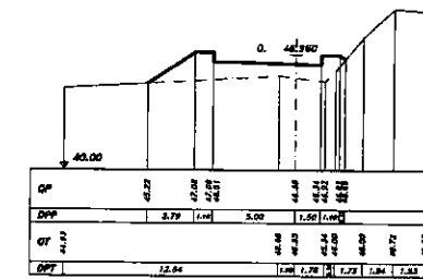
SEZIONE 27 PROGRESSIVA 410.00
