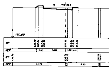
SEZIONE 51 PROGRESSIVA 60.00
