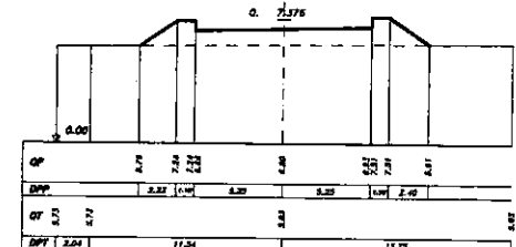
SEZIONE 8 PROGRESSIVA 359.32
