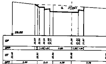
SEZIONE 2 PROGRESSIVA 280.00
