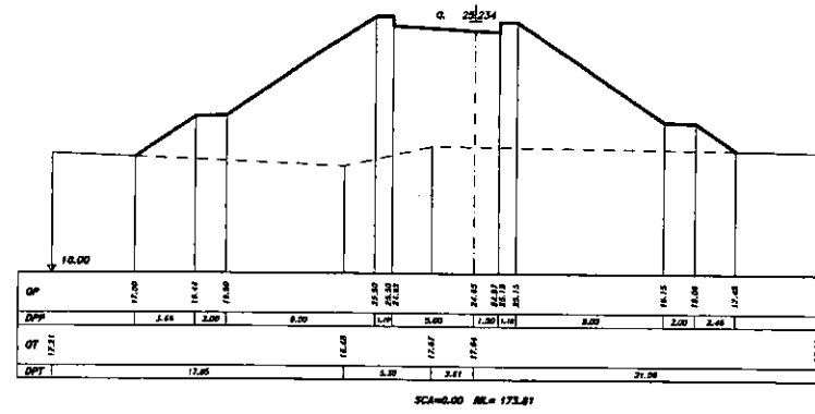
SEZIONE 64 PROGRESSIVA 410.00
