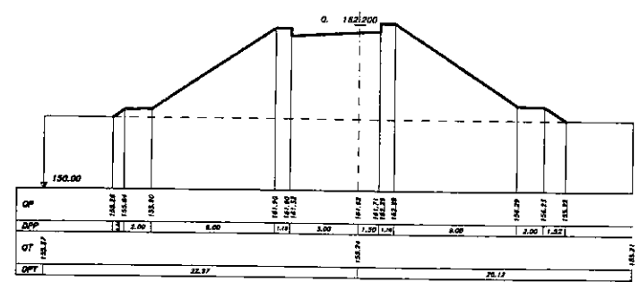
SEZIONE 31 PROGRESSIVA 0.00
