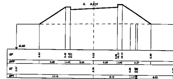
SEZIONE 8 PROGRESSIVA 359.32
