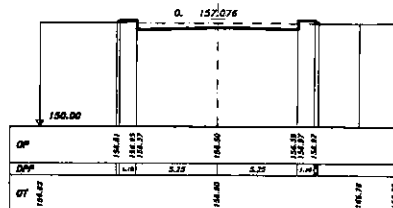
SEZIONE 11 PROGRESSIVA 500.00
