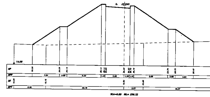
SEZIONE 47 PROGRESSIVA 240.00
