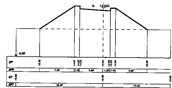
SEZIONE 35 PROGRESSIVA 1580.00
