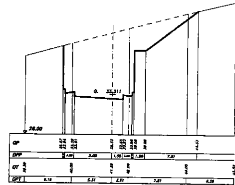
SEZIONE 54 PROGRESSIVA 120.00
