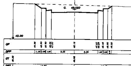
SEZIONE 4 PROGRESSIVA 168.00
