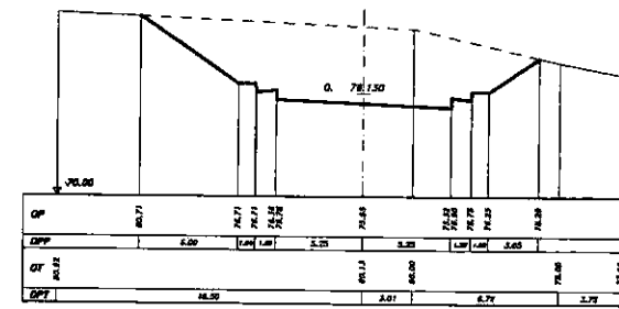
SEZIONE 8 PROGRESSIVA 330.00
