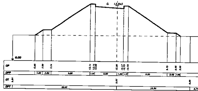
SEZIONE 31 PROGRESSIVA 350.00
