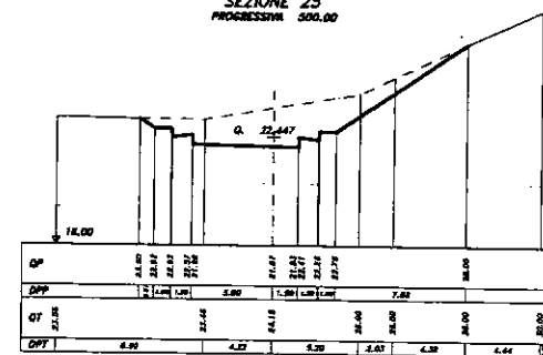
SEZIONE 25 PROGRESSIVA 500.00
