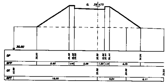
SEZIONE 2 PROGRESSIVA 42.00
