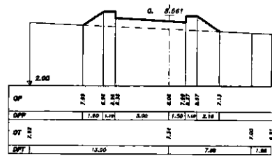
SEZIONE 21 PROGRESSIVA 140.00
