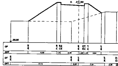
SEZIONE 19 PROGRESSIVA 275.00
