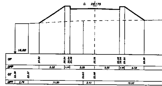
SEZIONE 3 PROGRESSIVA 45.00
