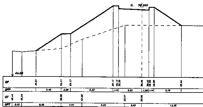
SEZIONE 56 PROGRESSIVA 185.00
