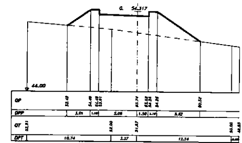
SEZIONE 35 PROGRESSIVA 285.00
