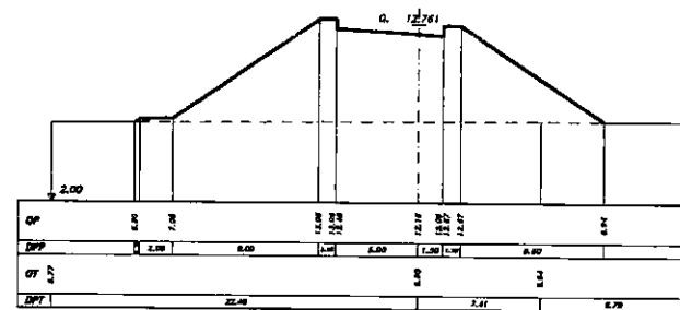
SEZIONE 25 PROGRESSIVA 290.00
