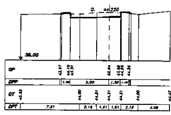
SEZIONE 28 PROGRESSIVA 0.00
