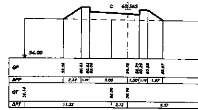
SEZIONE 32 PROGRESSIVA 255.00
