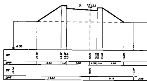
SEZIONE 36 PROGRESSIVA 1630.00
