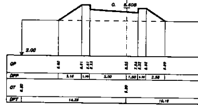
SEZIONE 31 PROGRESSIVA 350.00
