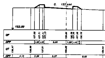
SEZIONE 52 PROGRESSIVA 100.00
