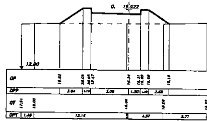
SEZIONE 8 PROGRESSIVA 77.00
