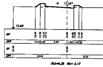
SEZIONE 73 PROGRESSIVA 43.00
