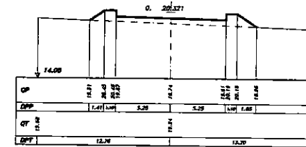
SEZIONE 4 PROGRESSIVA 220.00
