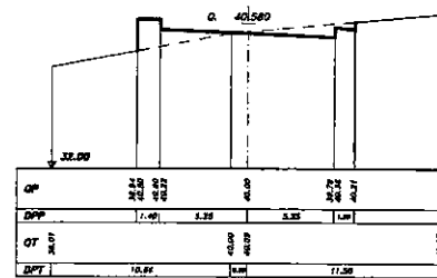
SEZIONE 10 PROGRESSIVA 260.00
