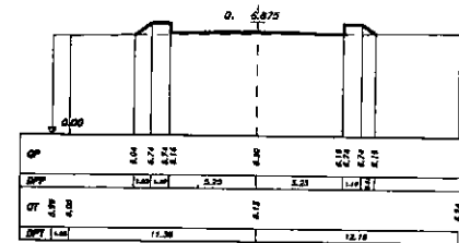
SEZIONE 5 PROGRESSIVA 205.00
