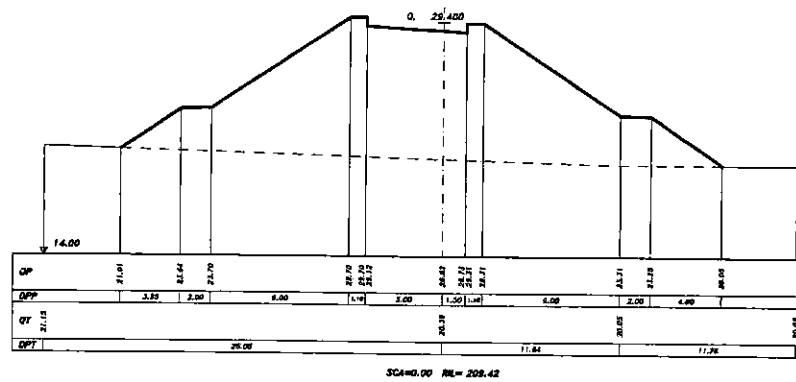
SEZIONE 48 PROGRESSIVA 270.00
