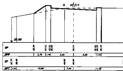
SEZIONE 14 PROGRESSIVA 360.00
