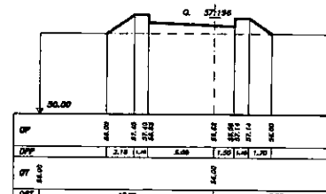
SEZIONE 54 PROGRESSIVA 120.00
