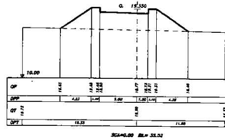
SEZIONE 72 PROGRESSIVA 13.00
