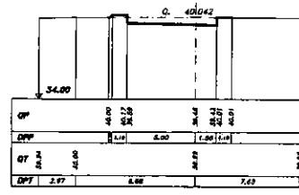
SEZIONE 11 PROGRESSIVA 10.00
