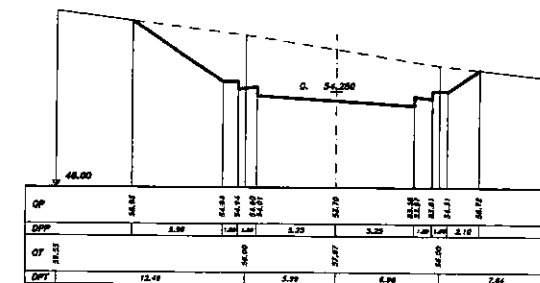
SEZIONE 8 PROGRESSIVA 320.50
