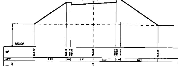
SEZIONE 17 PROGRESSIVA 760.00
