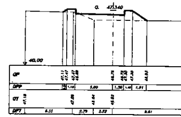
SEZIONE 31 PROGRESSIVA 150.00
