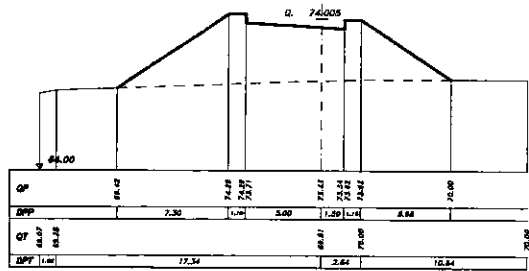
SEZIONE 12 PROGRESSIVA 170.00
