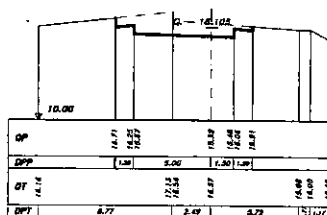
SEZIONE 91 PROGRESSIVA 115.00
