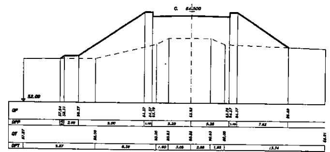
SEZIONE 4 PROGRESSIVA 155.00
