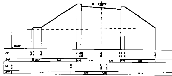
SEZIONE 6 PROGRESSIVA 310.00
