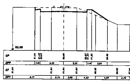
SEZIONE 2 PROGRESSIVA 75.00
