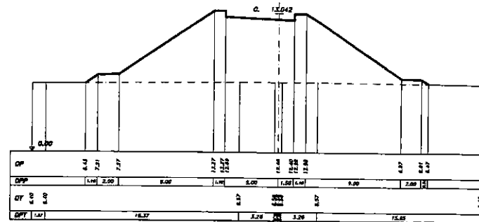
SEZIONE 16 PROGRESSIVA 180.00
