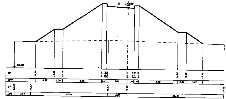
SEZIONE 36 PROGRESSIVA 250.00
