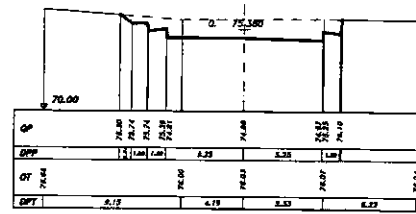
SEZIONE 7 PROGRESSIVA 305.00
