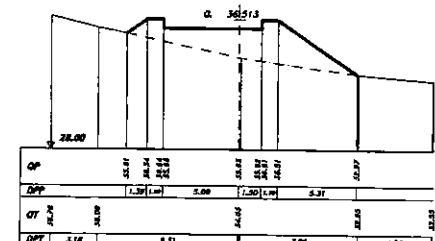
SEZIONE 62 PROGRESSIVA 227.00
