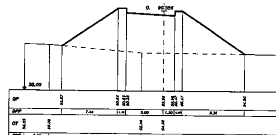
SEZIONE 59 PROGRESSIVA 270.00
