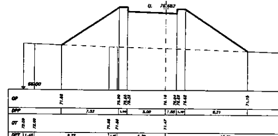
SEZIONE 16 PROGRESSIVA 331.00
