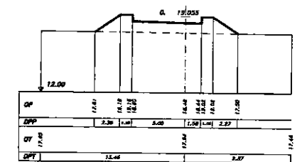
SEZIONE 14 PROGRESSIVA 303.00
