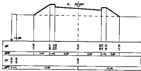
SEZIONE 5 PROGRESSIVA 265.00
