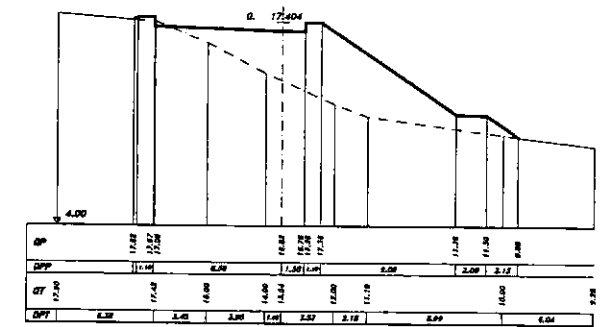
SEZIONE 29 PROGRESSIVA 1270.00
