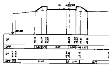
SEZIONE 34 PROGRESSIVA 255.00
