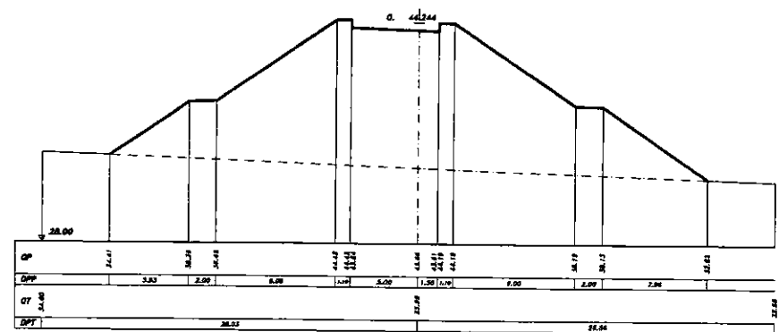
SEZIONE 5 PROGRESSIVA 147.00
