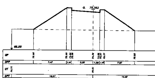
SEZIONE 13 PROGRESSIVA 210.00
