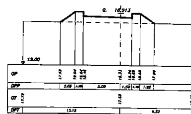
SEZIONE 15 PROGRESSIVA 338.00
