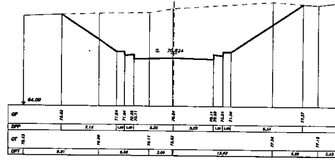
SEZIONE 2 PROGRESSIVA 65.00
