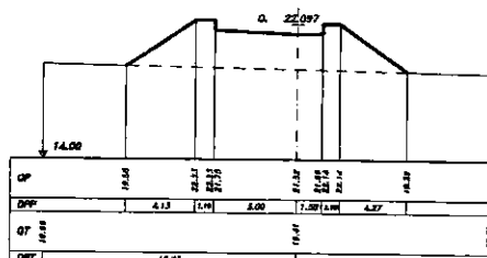
SEZIONE 13 PROGRESSIVA 90.00
