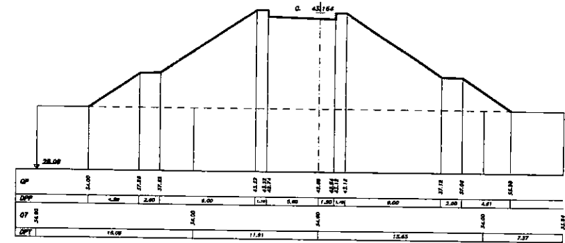
SEZIONE 7 PROGRESSIVA 252.00
