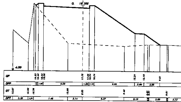
SEZIONE 31 PROGRESSIVA 1410.00
