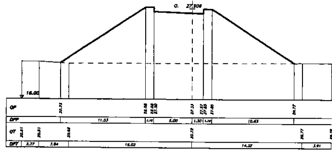
SEZIONE 10 PROGRESSIVA 220.00
