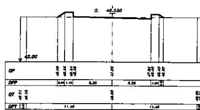
SEZIONE 2 PROGRESSIVA 95.00
