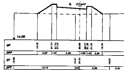
SEZIONE 23 PROGRESSIVA 430.00
