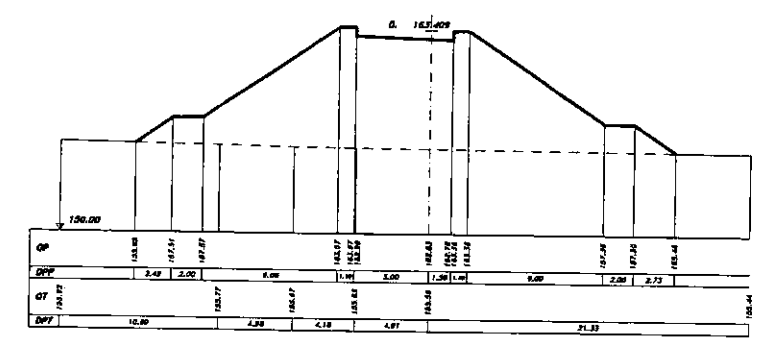
SEZIONE 33 PROGRESSIVA 80.00
