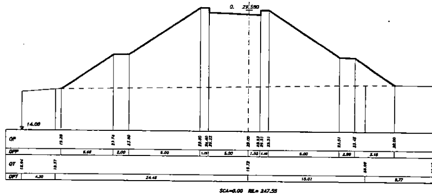
SEZIONE 46 PROGRESSIVA 310.00
