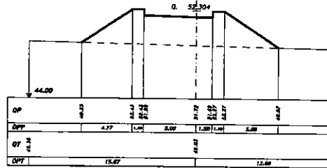
SEZIONE 16 PROGRESSIVA 210.00
