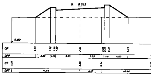
SEZIONE 7 PROGRESSIVA 310.00
