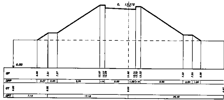
SEZIONE 14 PROGRESSIVA 100.00
