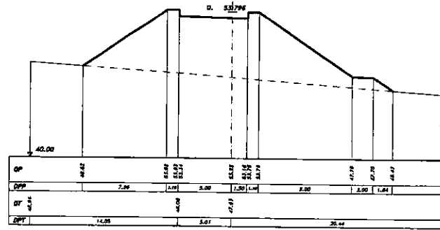
SEZIONE 34 PROGRESSIVA 255.00
