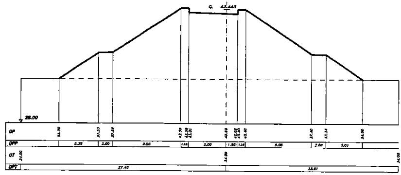
SEZIONE 4 PROGRESSIVA 112.00
