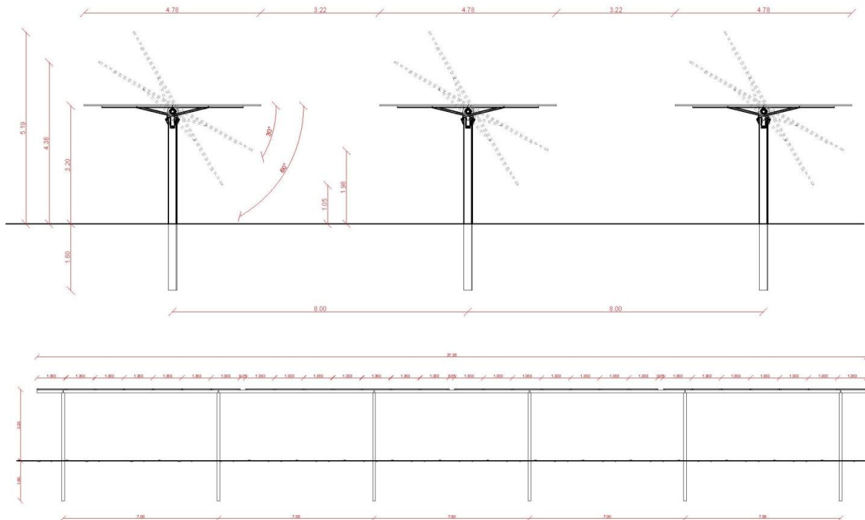
Figura 5- Sezioni tipo inseguitori monoassiali (trasversale – longitudinale).
