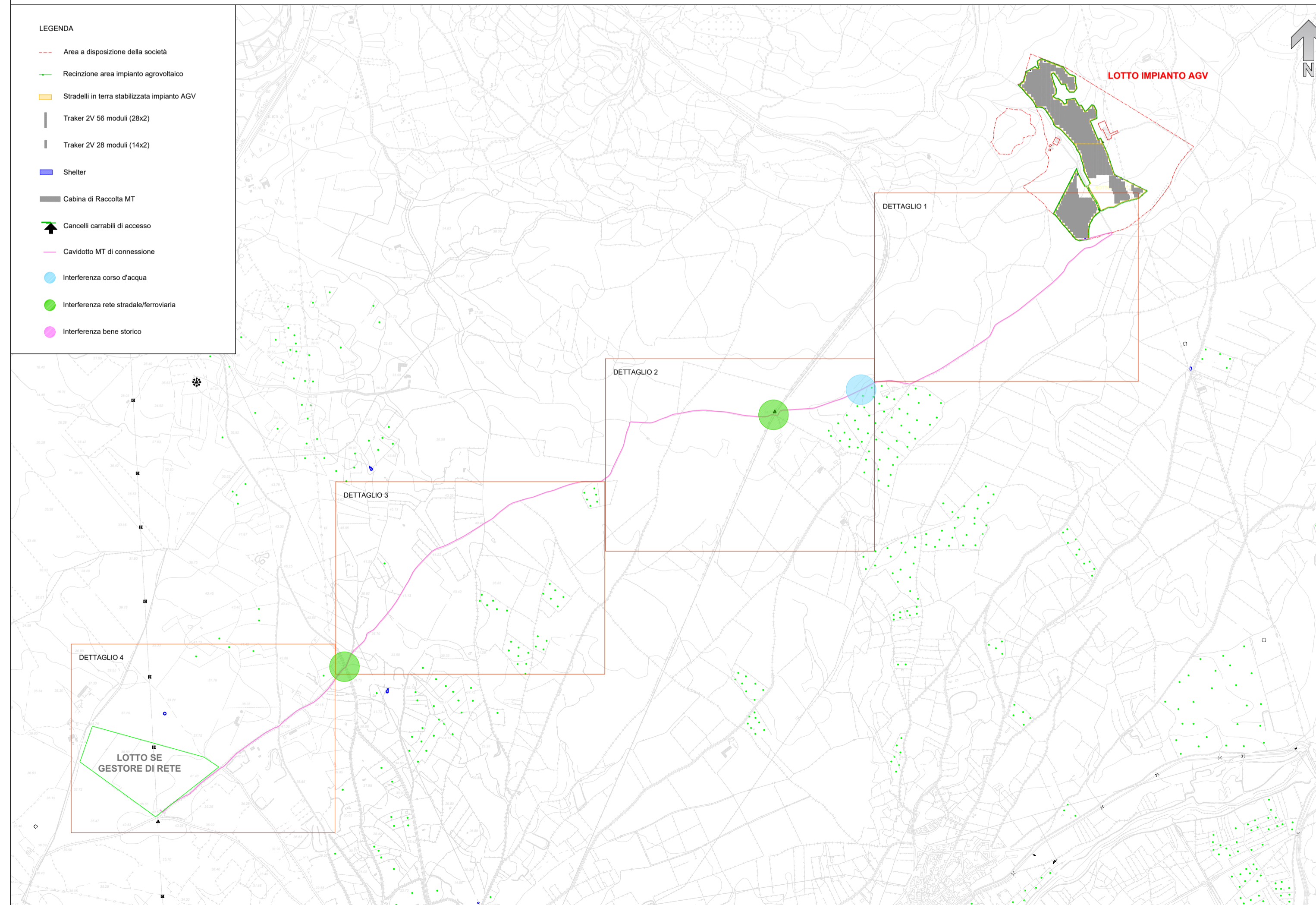
Stralcio CTR - Fogli 515130-514160-529010-528040_Lotto Impianto + linea di connessione MT Scala 1:20.000
