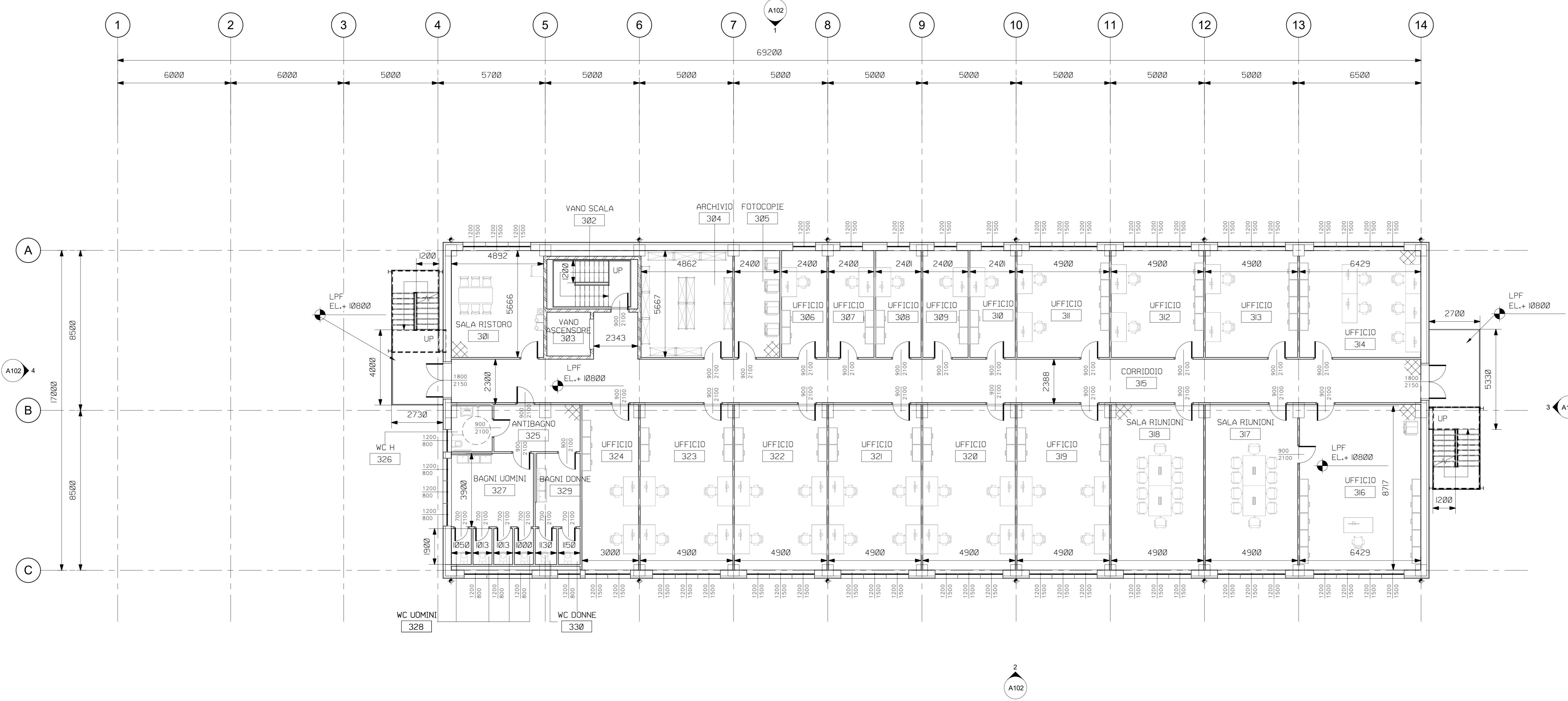
3 PIANTA SECONDO PIANO 1 : 100
