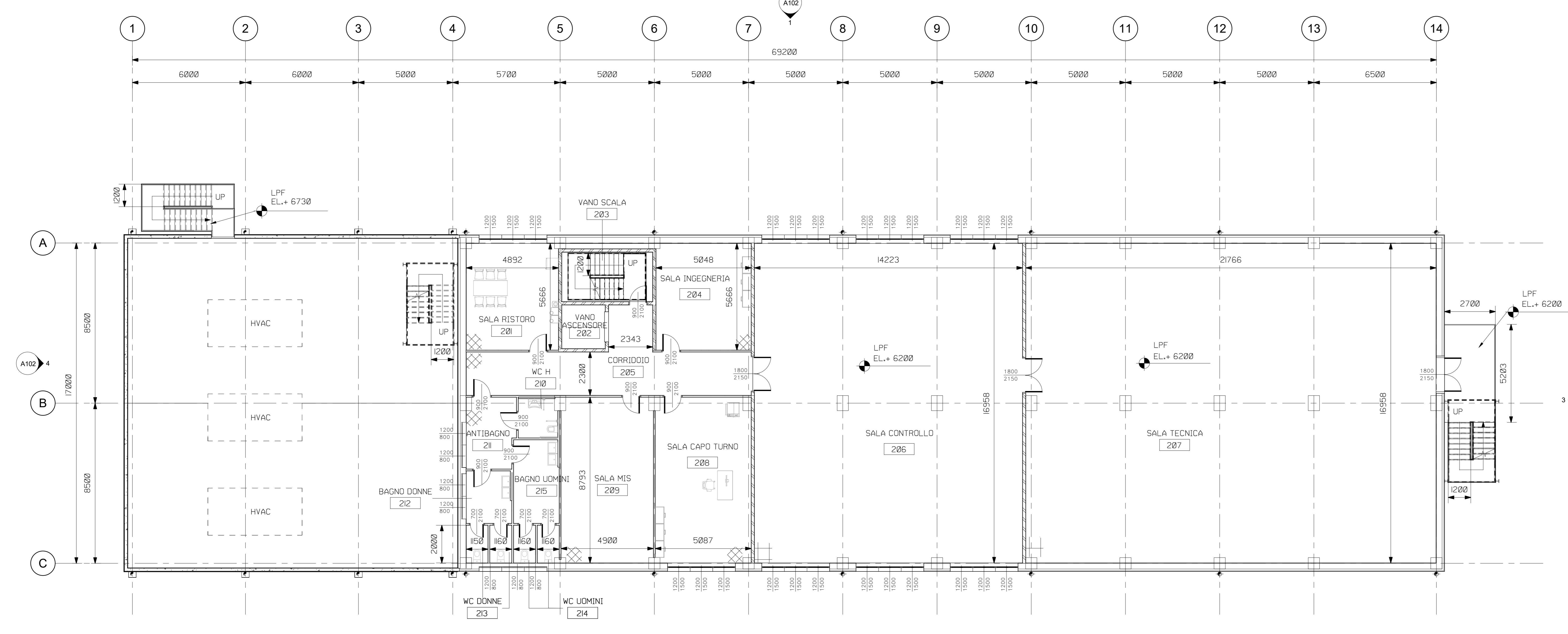
1 PIANTA PIANO TERRA 1 : 100
